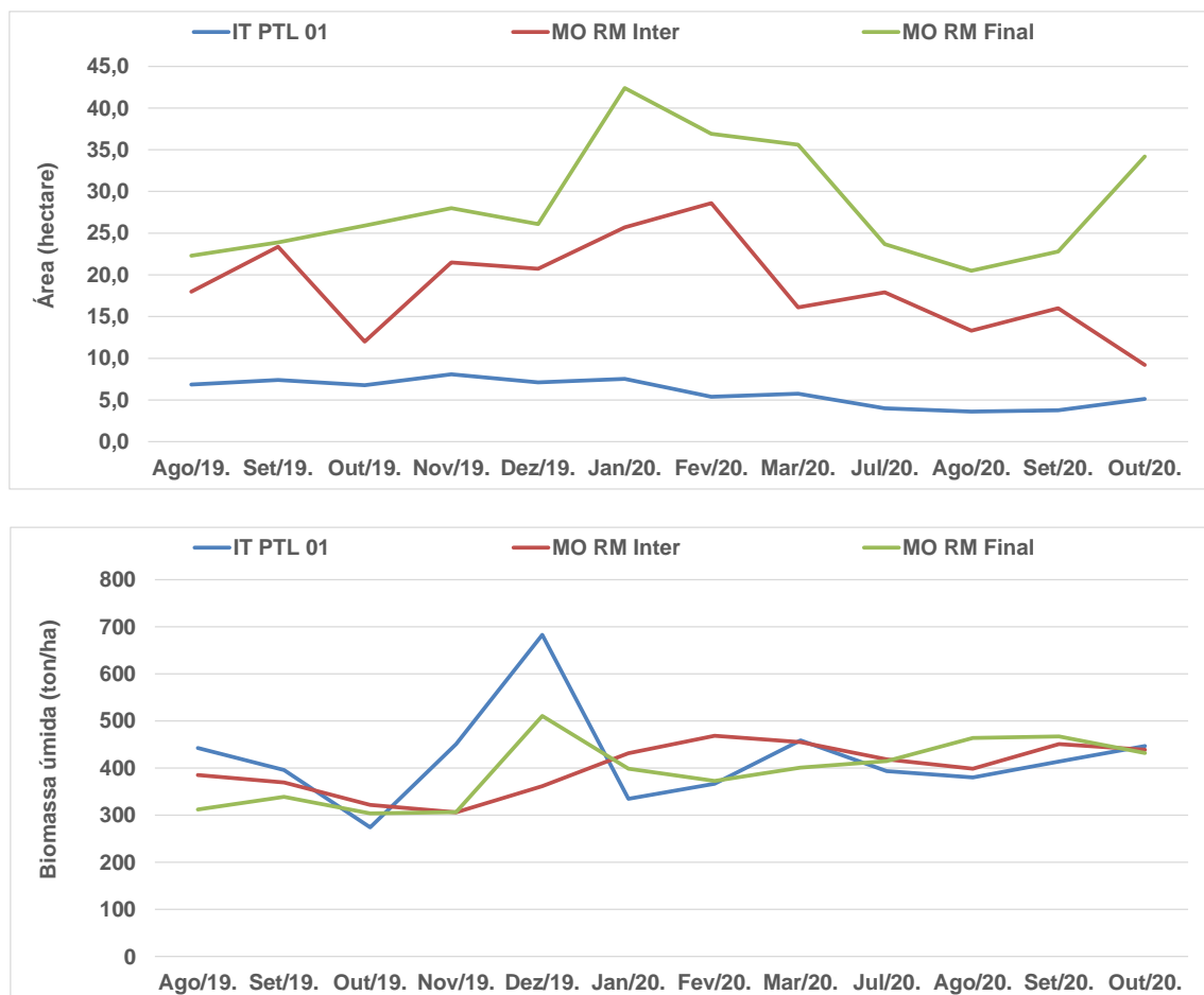
Figura 7 – Variação temporal da área coberta por macrófitas (acima) e da biomassa úmida específica (abaixo) nos prados monitorados, demonstrando as respectivas diferenças entre os meses de amostragem.
