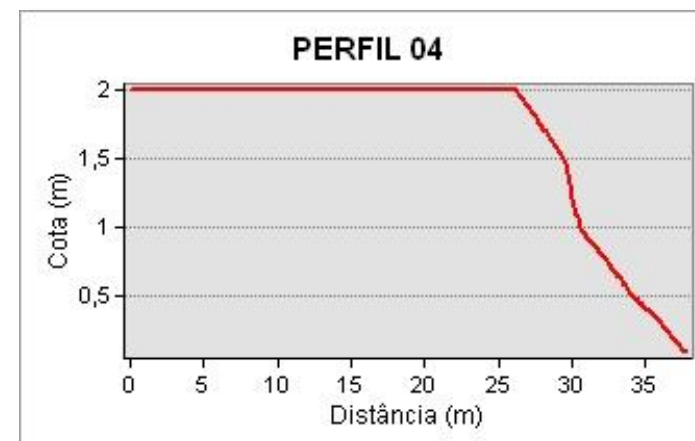
Figura 32 - Perfis de elevação gerados a partir modelo numérico de terreno da área de monitoramento 5.2.
