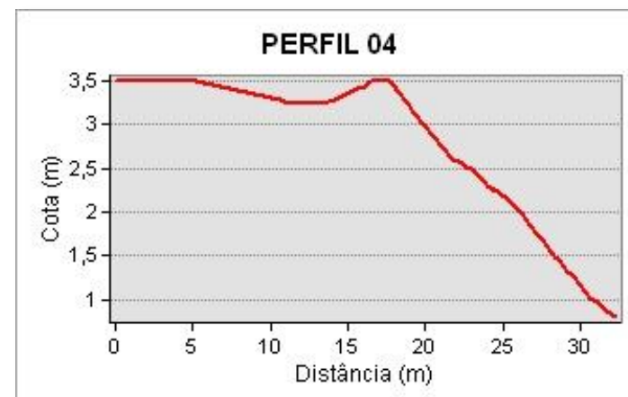
Figura 26 - Perfis de elevação gerados a partir modelo numérico de terreno da área de monitoramento 5.1A.
