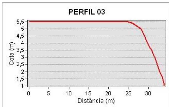
Figura 47 - Perfis de elevação gerados a partir modelo numérico de terreno da área de monitoramento B-10.
