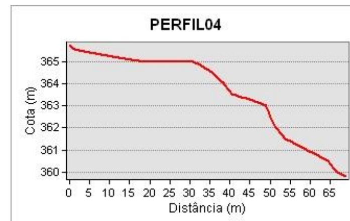
Figura 8 - Perfis de elevação gerados a partir modelo numérico de terreno da área de monitoramento 1.3.
