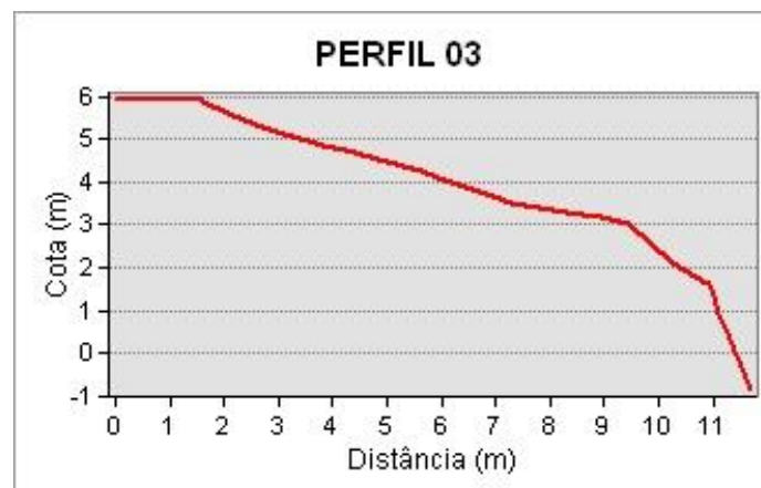
Figura 29 - Perfis de elevação gerados a partir modelo numérico de terreno da área de monitoramento 5.1B.
