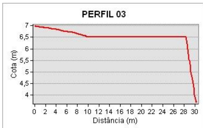
Figura 38 - Perfis de elevação gerados a partir modelo numérico de terreno da área de monitoramento B-06.
