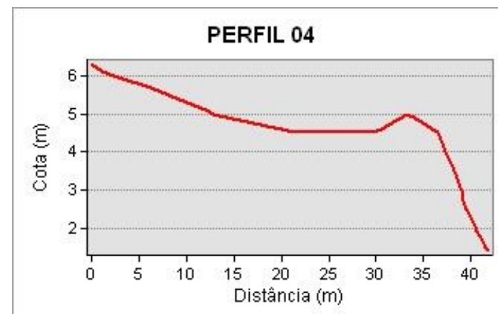
Figura 20 - Perfis de elevação gerados a partir modelo numérico de terreno da área de monitoramento 4.3A.
