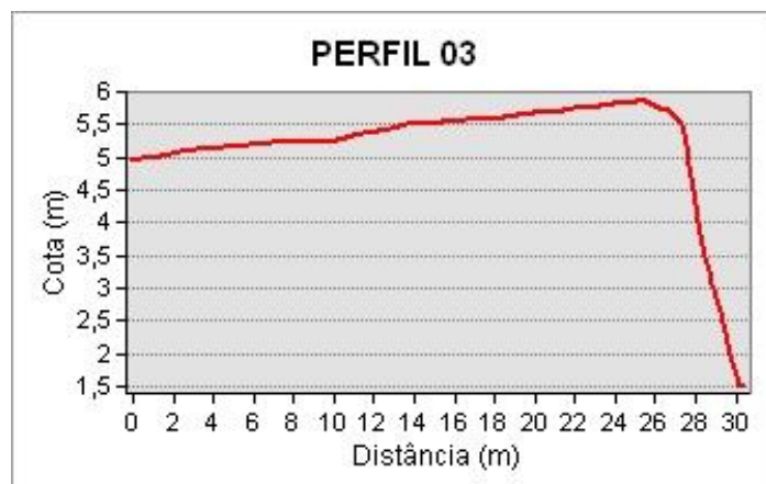
Figura 44 - Perfis de elevação gerados a partir modelo numérico de terreno da área de monitoramento B-09.
