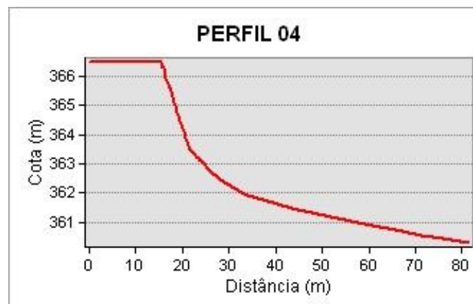
Figura 5 - Perfis de elevação gerados a partir modelo numérico de terreno da área de monitoramento 1.1.
