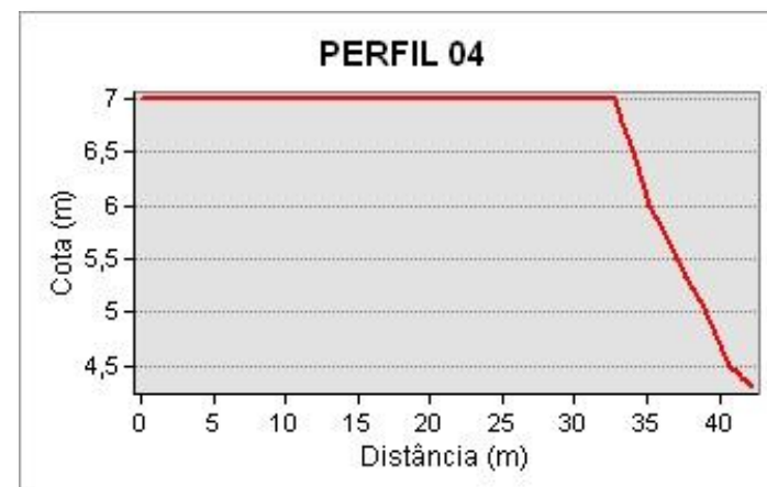
Figura 35 - Perfis de elevação gerados a partir modelo numérico de terreno da área de monitoramento B-05.
