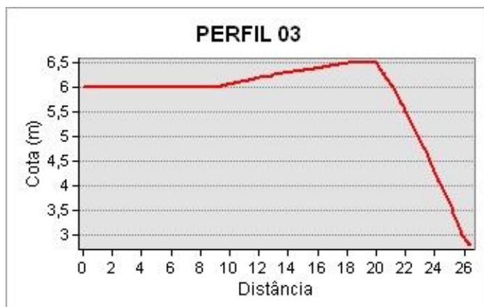
Figura 41 - Perfis de elevação gerados a partir modelo numérico de terreno da área de monitoramento B-08.
