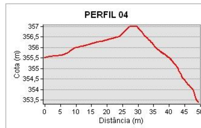
Figura 14 - Perfis de elevação gerados a partir modelo numérico de terreno da área de monitoramento 2.5.
