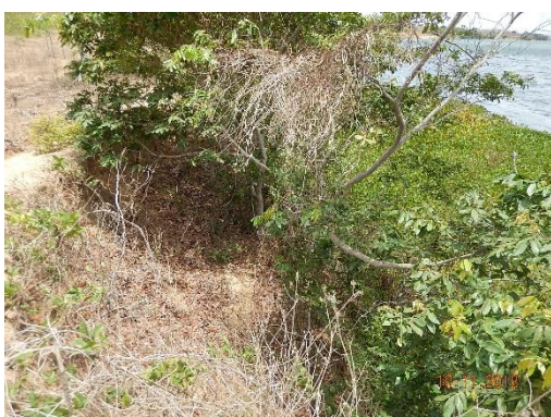
Foto 31- Detalhe da elevada inclinação do talude e exposição do solo.
