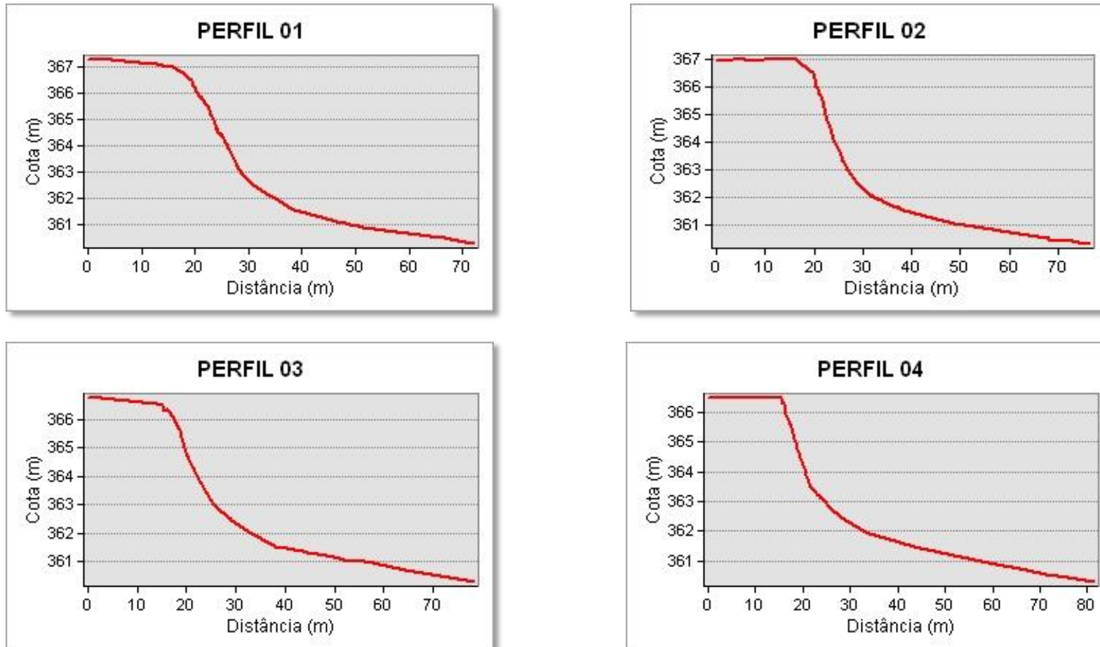
Figura 5 - Perfis de elevação gerados a partir modelo numérico de terreno da área de monitoramento 1.1.
