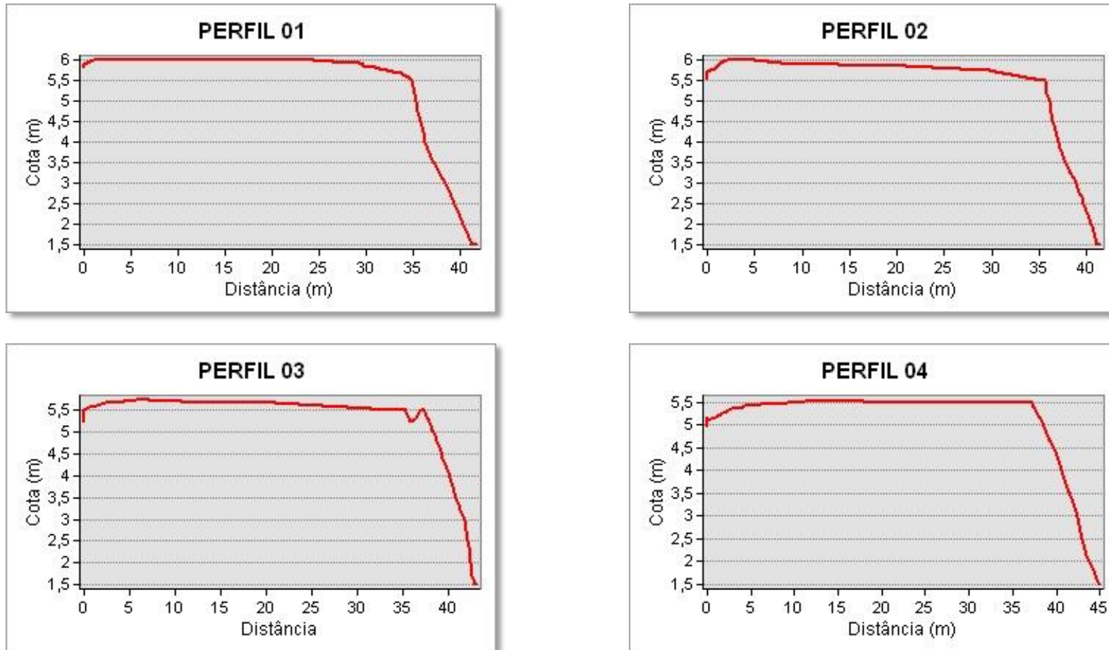
Figura 23 - Perfis de elevação gerados a partir modelo numérico de terreno da área de monitoramento 4.3B.
