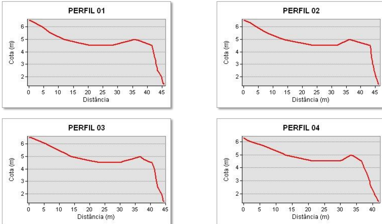
Figura 20 - Perfis de elevação gerados a partir modelo numérico de terreno da área de monitoramento 4.3A.
