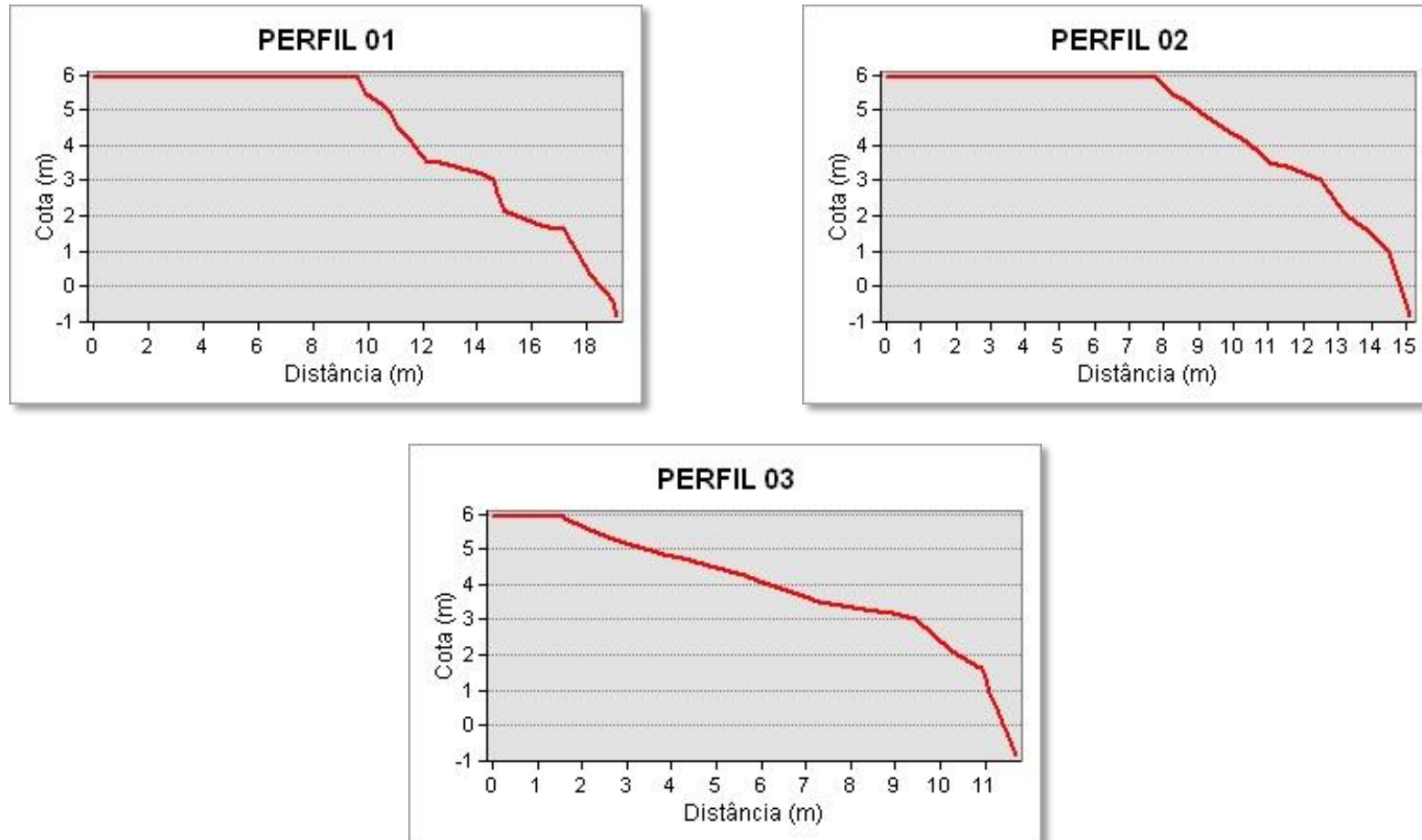
Figura 29 - Perfis de elevação gerados a partir modelo numérico de terreno da área de monitoramento 5.1B.
