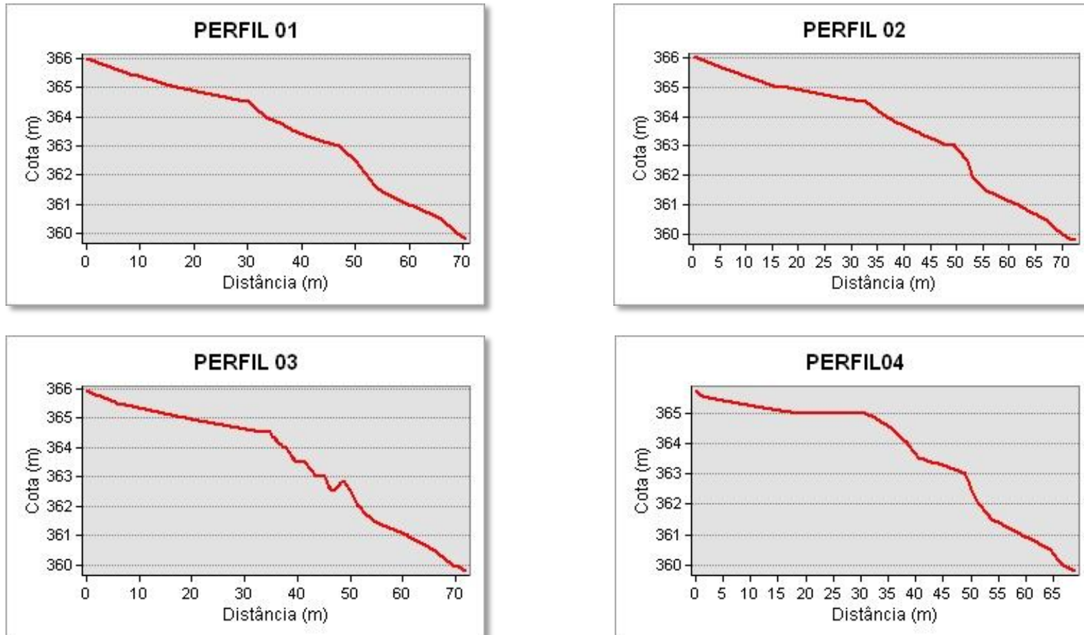
Figura 8 - Perfis de elevação gerados a partir modelo numérico de terreno da área de monitoramento 1.3.
