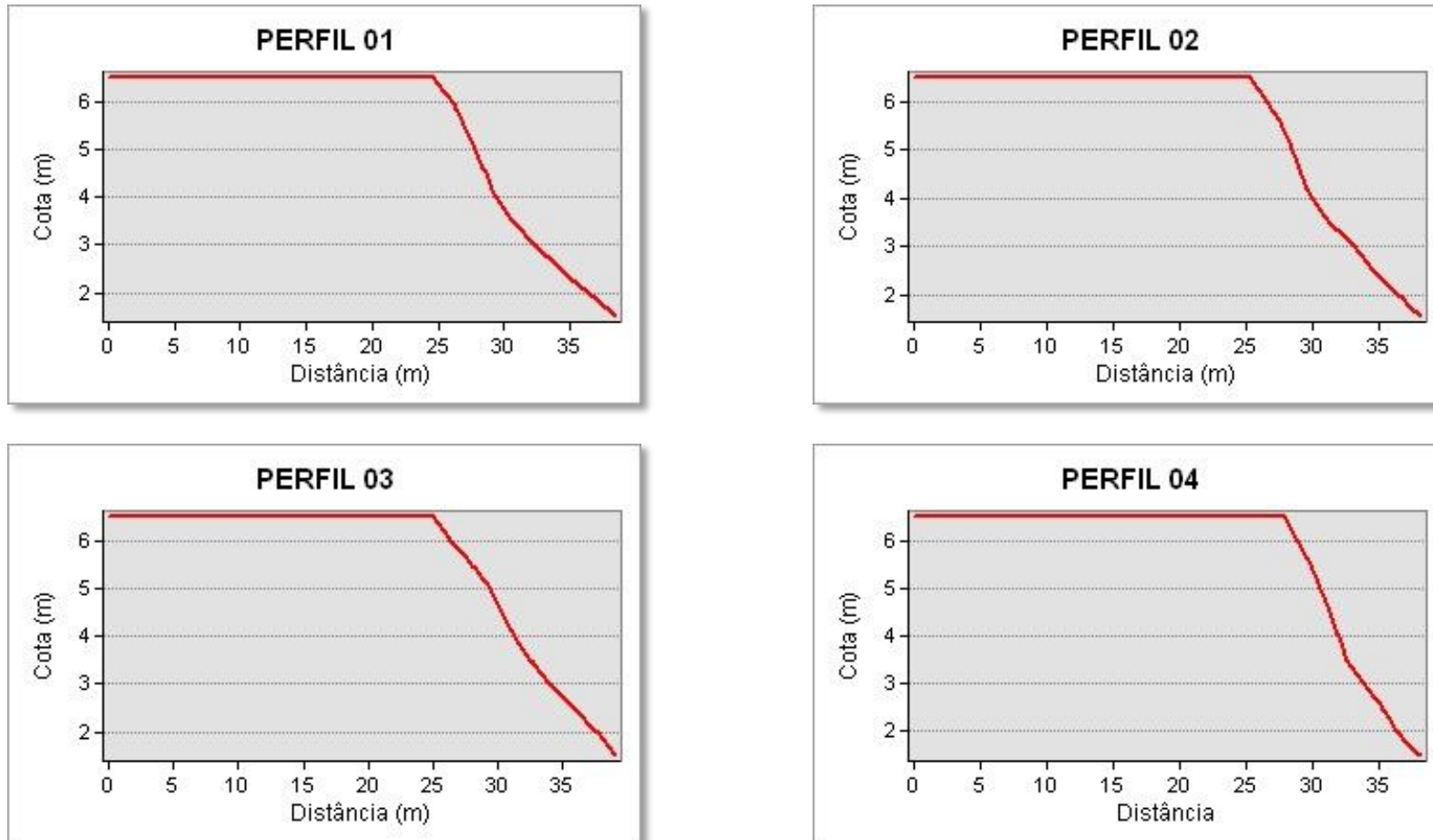
Figura 17 - Perfis de elevação gerados a partir modelo numérico de terreno da área de monitoramento 4.2.
