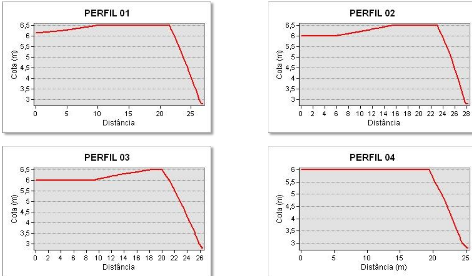
Figura 41 - Perfis de elevação gerados a partir modelo numérico de terreno da área de monitoramento B-08.
