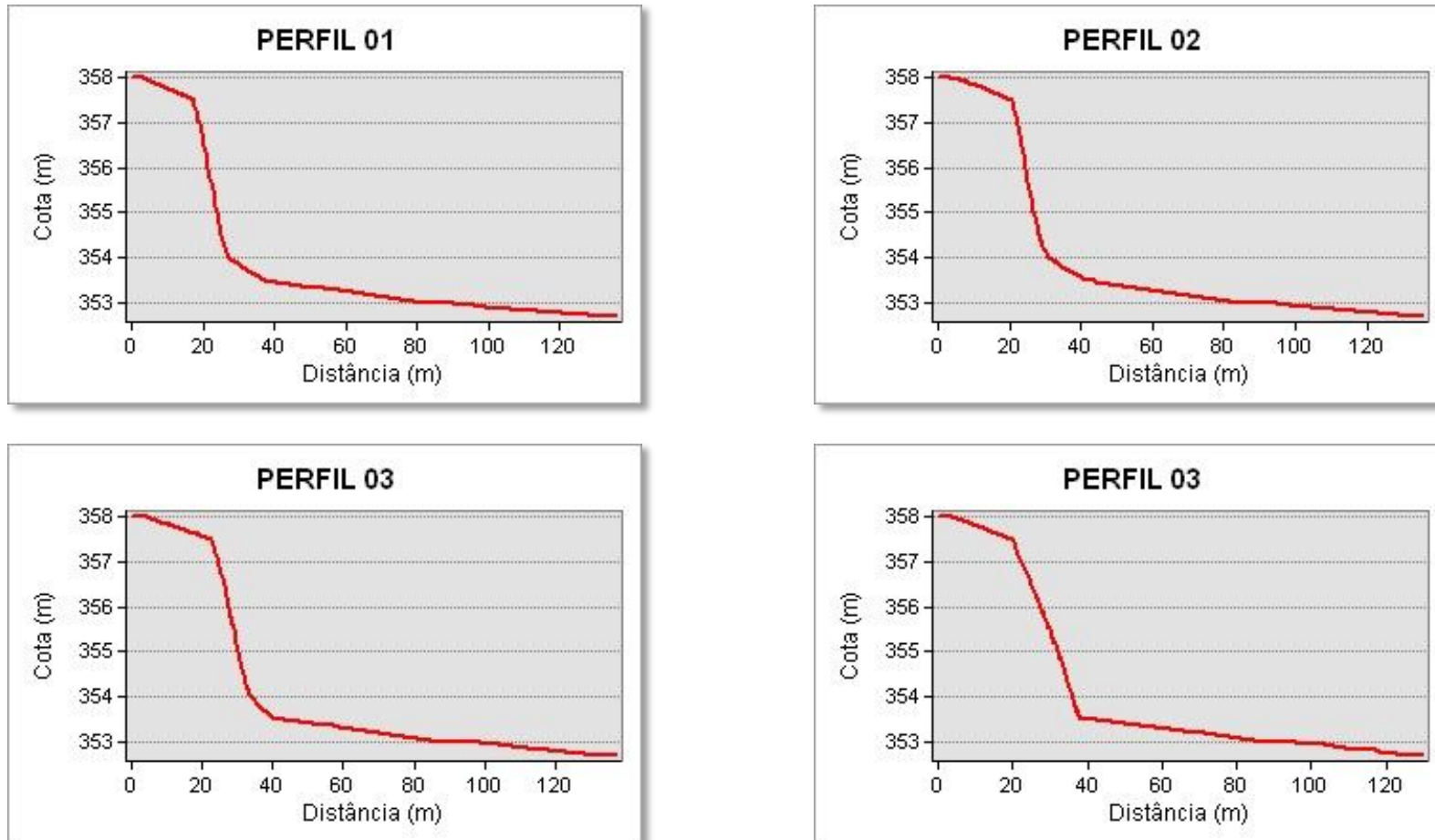
Figura 11 - Perfis de elevação gerados a partir modelo numérico de terreno da área de monitoramento 2.1.
