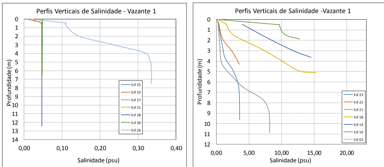
Figura 15 - Perfis verticais de salinidade para as estações amostrais. Campanha 25 - Vazante 1 - 14/10/2018. CONAMA 357/2005 (I - águas doces: águas com salinidade igual ou inferior a 0,5 ‰).
