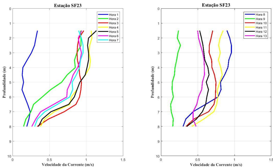
Figura 9 - Perfis verticais de velocidade de corrente na estação fixa ESF 23. Campanha 25 - 12/10/2018.
