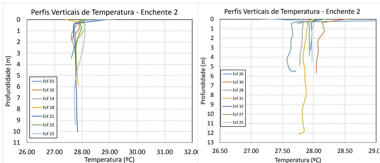
Figura 26 - Perfis verticais de temperatura para as estações amostrais. Campanha 25 -Enchente 2 - 15/10/2018.
