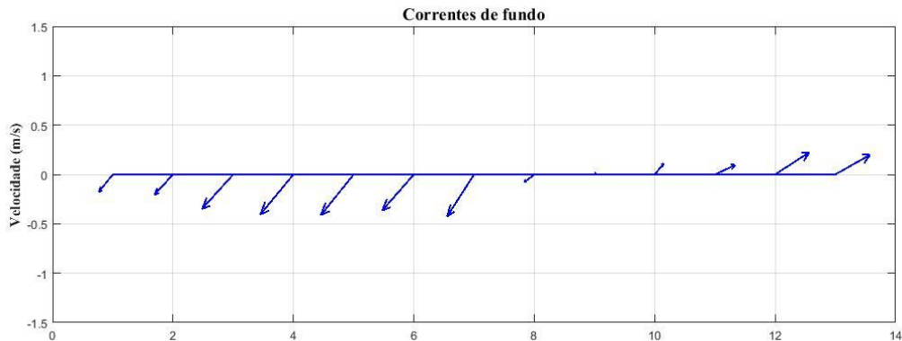
Figura 32 - Diagrama de vetores das correntes em superfície, meia água e fundo para a estação fixa ESF 23. Campanha 26 - 23/10/2018.
