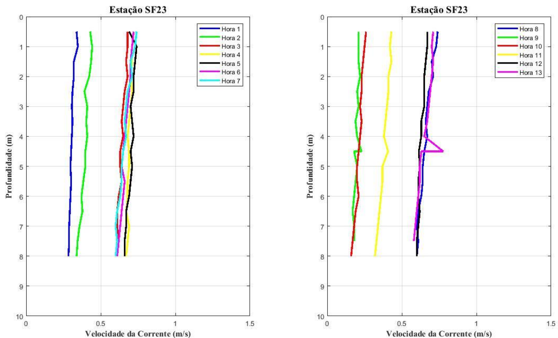
Figura 33 - Perfis verticais de velocidade de corrente na estação fixa ESF 23. Campanha 26 - 23/10/2018.
