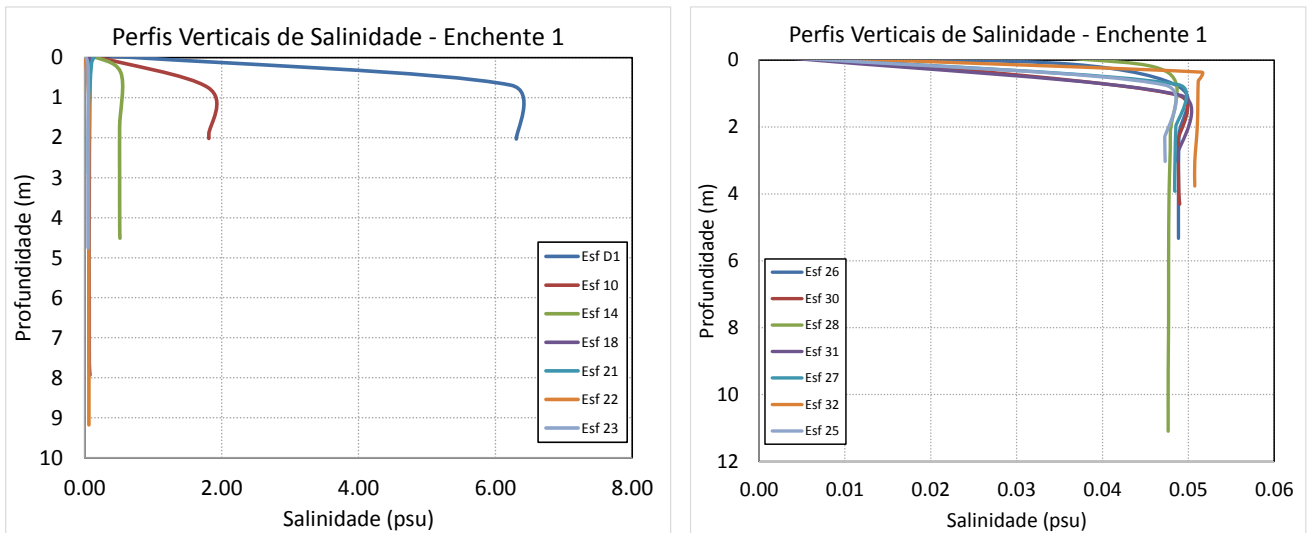
Figura 43 - Perfis verticais de salinidade para as estações amostrais. Campanha 26 - Enchente 1 - 25/10/2018.
