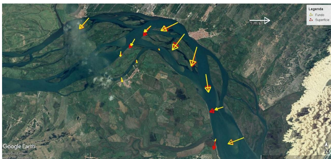
Figura 36 - Média vertical da velocidade e direção da corrente em cada estação amostral. Campanha 26 - Vazante 1 - 25/10/2018.
