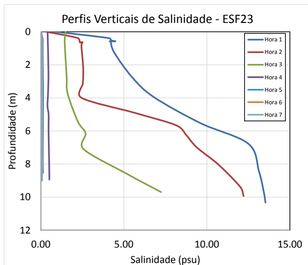
Figura 35 - Perfis verticais de salinidade na estação fixa ESF 23 Campanha 26 - 23/10/2018. Resolução CONAMA 357/2005 (I - águas doces: águas com salinidade igual ou inferior a 0,5 ‰).
