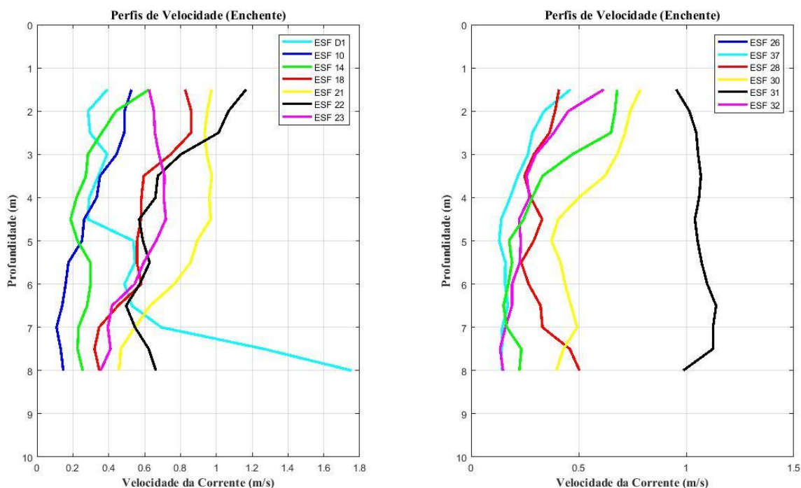
Figura 25 - Perfis verticais de velocidade de corrente para as estações amostrais em período de maré enchente. Campanha 25 - Enchente 2 - 15/10/2018.
