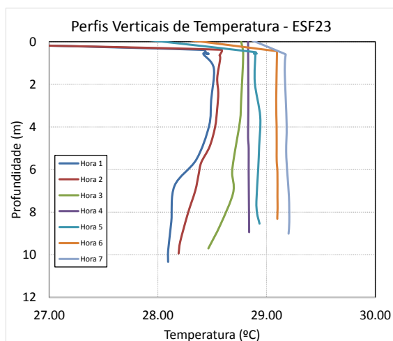
Figura 34 - Perfis verticais de temperatura para a estação fixa na estação fixa ESF 23. Campanha 26 - 23/10/2018.
