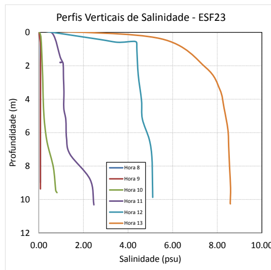
Figura 35 - Perfis verticais de salinidade na estação fixa ESF 23 Campanha 26 - 23/10/2018. Resolução CONAMA 357/2005 (I - águas doces: águas com salinidade igual ou inferior a 0,5 ‰).
