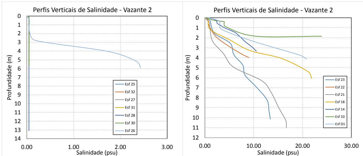
Figura 23 - Perfis verticais de salinidade para as estações amostrais. Campanha 25 - Vazante 2 - 15/10/2018. Resolução CONAMA 357/2005 (I - águas doces: águas com salinidade igual ou inferior a 0,5 ‰).
