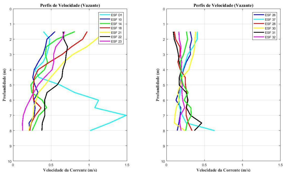
Figura 13 - Perfis verticais de velocidade de corrente para as estações amostrais em período de maré vazante. Campanha 25 - Vazante 1 - 14/10/2018.
