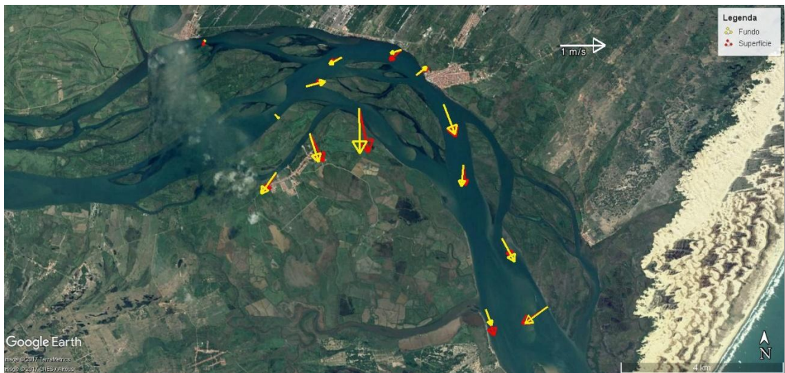
Figura 24 - Média vertical da velocidade e direção da corrente em cada estação amostral. Campanha 25 - Enchente 2 - 15/10/2018.
