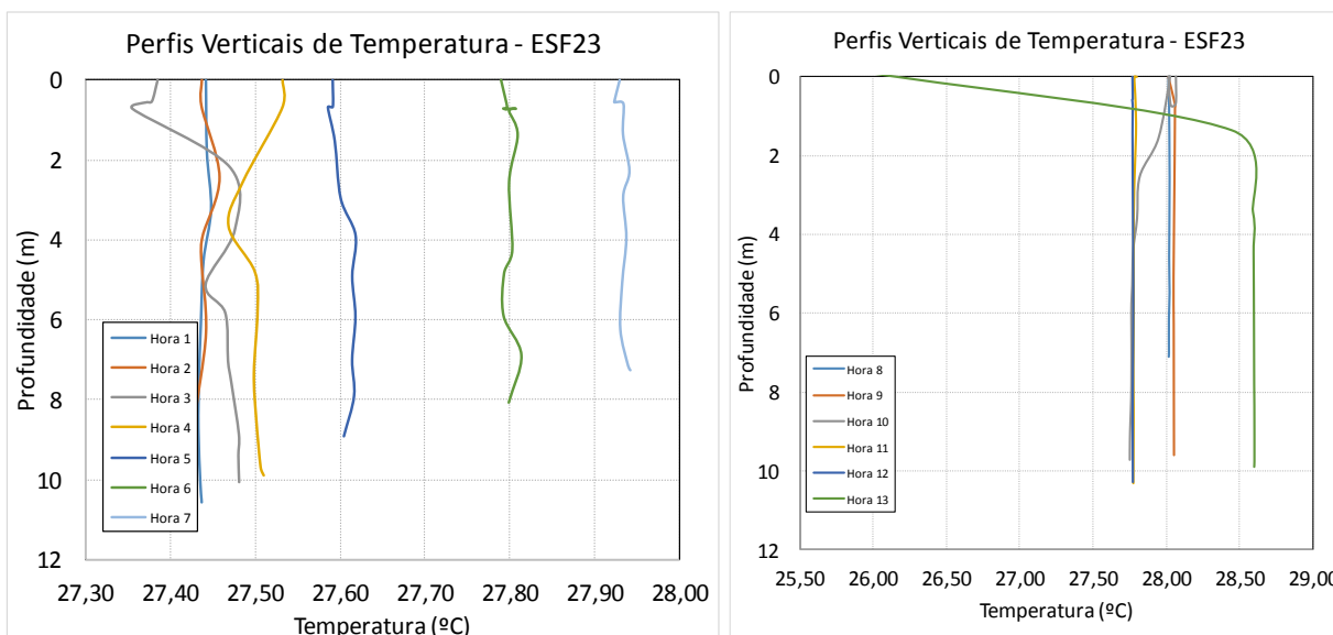
Figura 10 - Perfis verticais de temperatura para a estação amostral fixa ESF 23. Campanha 25 - 12/10/2018.
