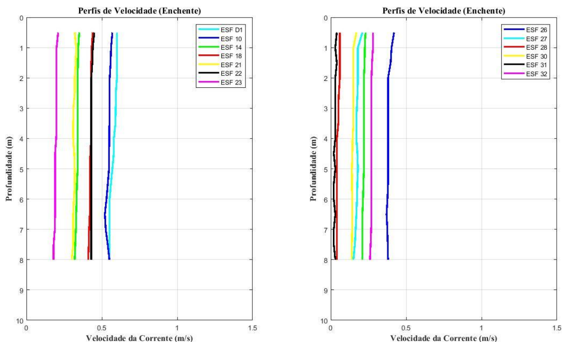
Figura 49 - Perfis verticais de velocidade de corrente para as estações amostrais em período de maré enchente. Campanha 26 - Enchente 2 - 26/10/2018.
