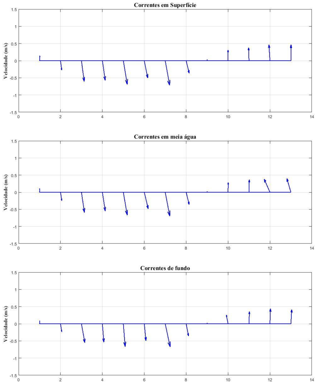
Figura 28 - Diagrama de vetores das correntes em superfície, meia água e fundo para a estação fixa ESF 32. Campanha 26-24/10/2018.
