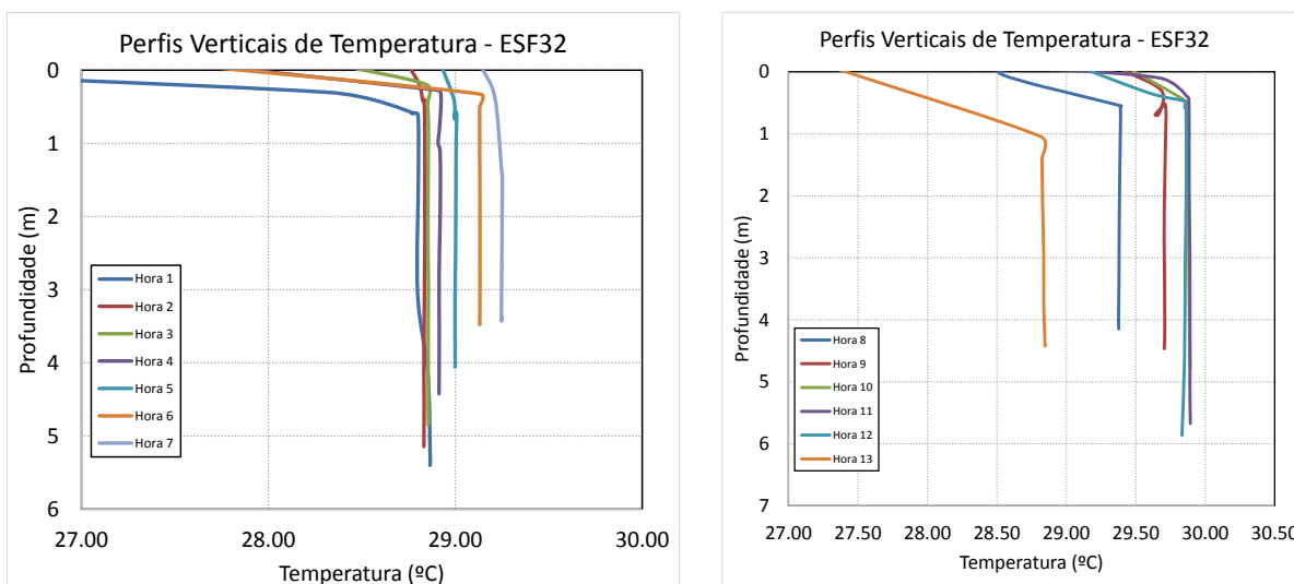
Figura 30- Perfis verticais de temperatura para a estação fixa ESF_32. Campanha 2 - 13 horas - Campanha 26 - 24/10/2018.
