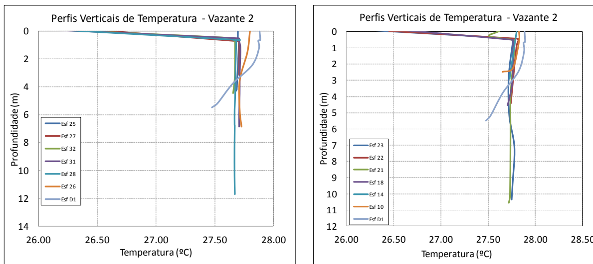
Figura 46 -Perfis verticais de temperatura para as estações amostrais. Campanha 26 - Vazante 2 - 26/10/2018.
