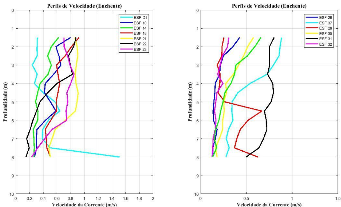
Figura 17 - Perfis verticais de velocidade de corrente para as estações amostrais em período de maré enchente. Campanha 25 - Enchente 1 - 14/10/2018.
