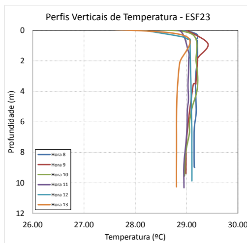
Figura 34 - Perfis verticais de temperatura para a estação fixa na estação fixa ESF 23. Campanha 26 - 23/10/2018.
