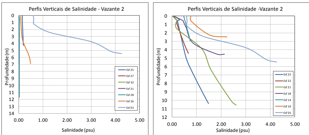
Figura 47 - Perfis verticais de salinidade para as estações amostrais. Campanha 26 - Vazante 2 - 26/10/2018.
