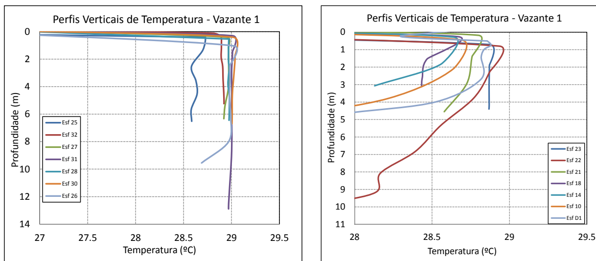
Figura 38 -Perfis verticais de temperatura para as estações amostrais. Campanha 26 – Vazante1 -25/10/2018.
