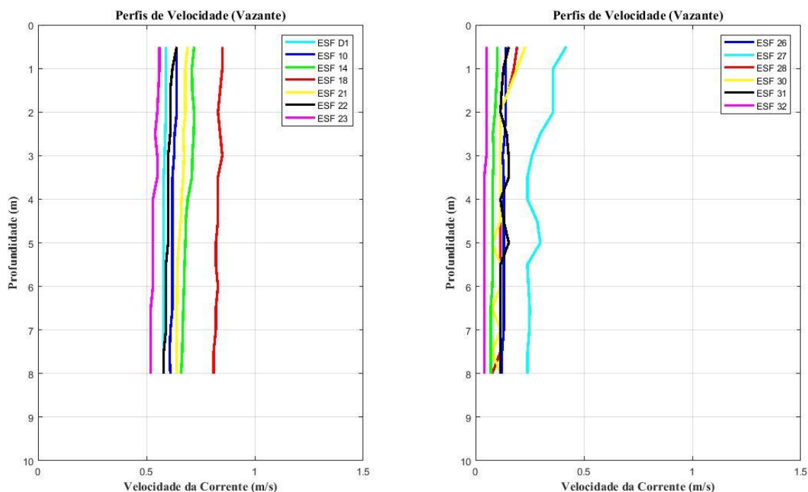
Figura 45 - Perfis verticais de velocidade de corrente para as estações amostrais em período de maré vazante. Campanha 26 - Vazante 2 - 26/10/2018.
