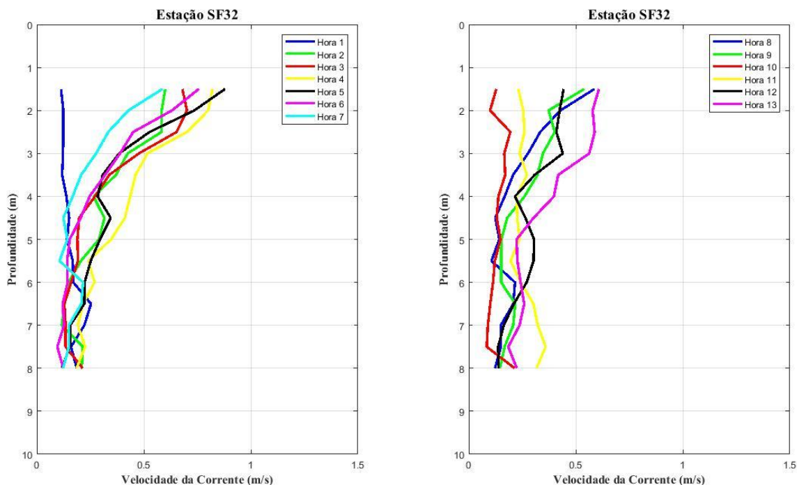
Figura 5 - Perfis verticais de velocidade de corrente na estação fixa ESF 32. Campanha 25 - 13/10/2018.
