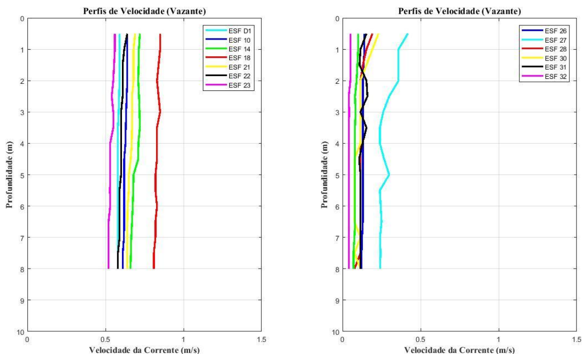
Figura 37 - Perfis verticais de velocidade de corrente para as estações amostrais em período de maré vazante Campanha 26 - Vazante 1 - 25/10/2018.
