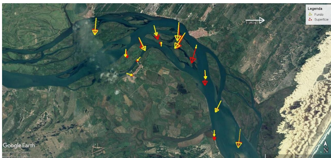
Figura 12 - Média vertical da velocidade e direção da corrente em cada estação amostral. Campanha 21 - Vazante 1 - 17/04/2018.
