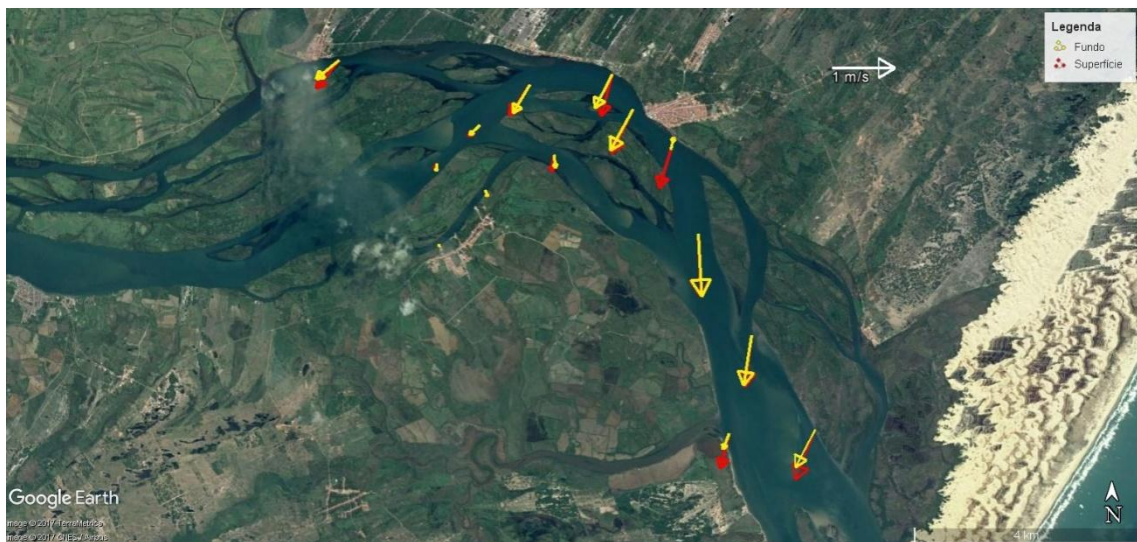
Figura 20 - Média vertical da velocidade e direção da corrente em cada estação amostral. Campanha 25 - Vazante 2 - 15/10/2018.
