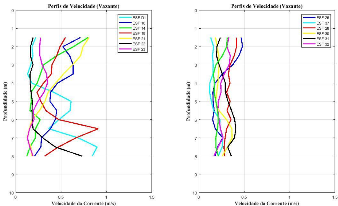
Figura 21 - Perfis verticais de velocidade de corrente para as estações amostrais em período de maré vazante. Campanha 25 - Vazante 2 - 15/10/2018.
