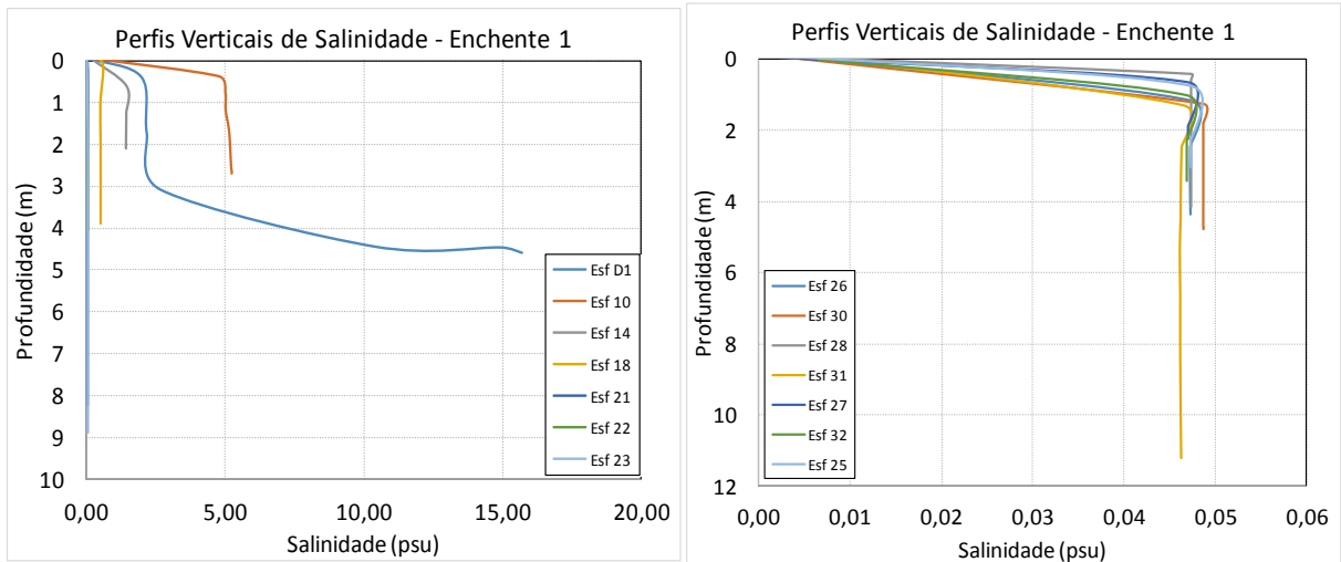
Figura 19 - Perfis verticais de salinidade para as estações amostrais. Campanha 25 - Enchente 1 - 14/10/2018. Resolução CONAMA 357/2005 (I - águas doces: águas com salinidade igual ou inferior a 0,5 ‰).
