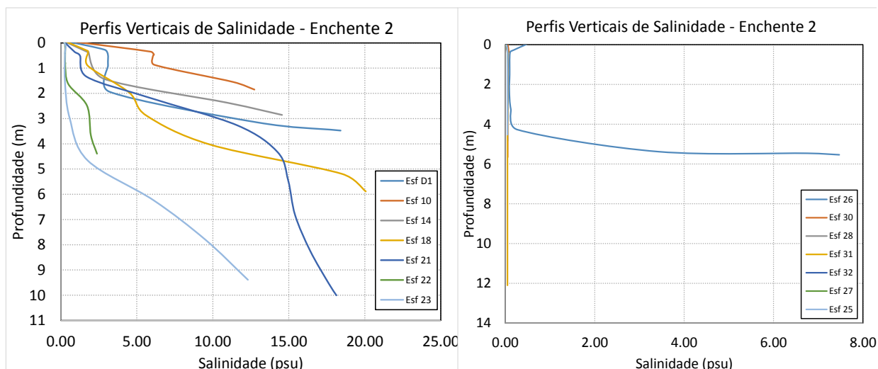
Figura 27 - Perfis verticais de salinidade para as estações amostrais. Campanha 25 - Enchente 2 - 15/10/2018. Resolução CONAMA 357/2005 (I - águas doces: águas com salinidade igual ou inferior a 0,5 ‰).
