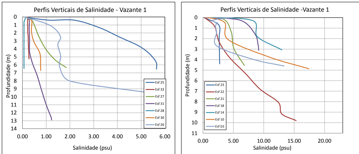
Figura 39 -Perfis verticais de salinidade para as estações amostrais. Campanha 26 - Vazante 1 - 25/10/2018.
