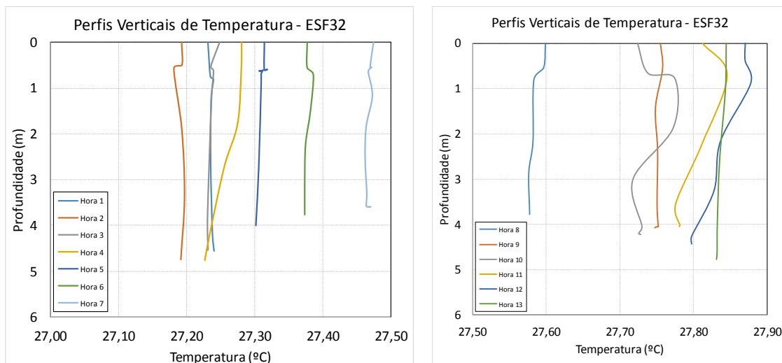
Figura 6 - Perfis verticais de temperatura para a estação amostral fixa ESF 32. Campanha 25 - Vazante 13/10/2018.
