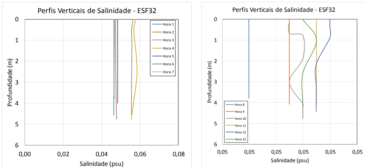
Figura 7 - Perfis verticais de salinidade para a estação amostral fixa ESF 32. Campanha 25 - 13/10/2018. Resolução CONAMA 357/2005 (I - águas doces: águas com salinidade igual ou inferior a 0,5 ‰).
