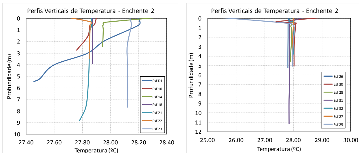
Figura 50 - Perfis verticais de temperatura para as estações amostrais. Campanha 26 - Enchente 2 - 26/10/2018.
