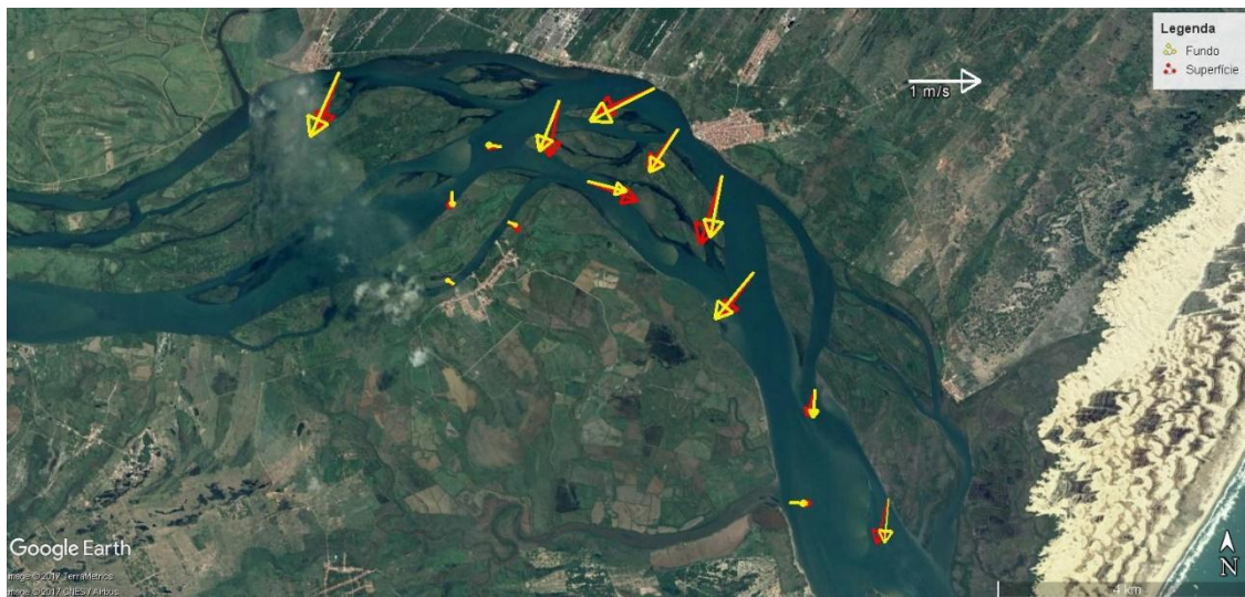
Figura 40 - Média vertical da velocidade e direção da corrente em cada estação amostral. Campanha 26 - Enchente 1 - 25/10/2018.
