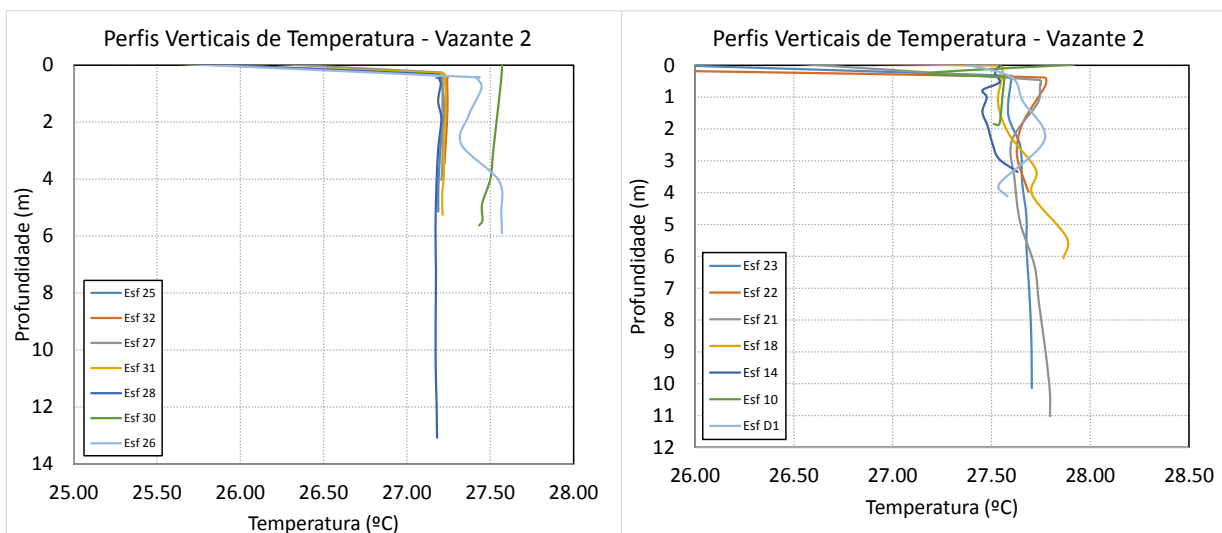
Figura 22 - Perfis verticais de temperatura para as estações amostrais. Campanha 25 - Vazante 2 - 15/10/2018.
