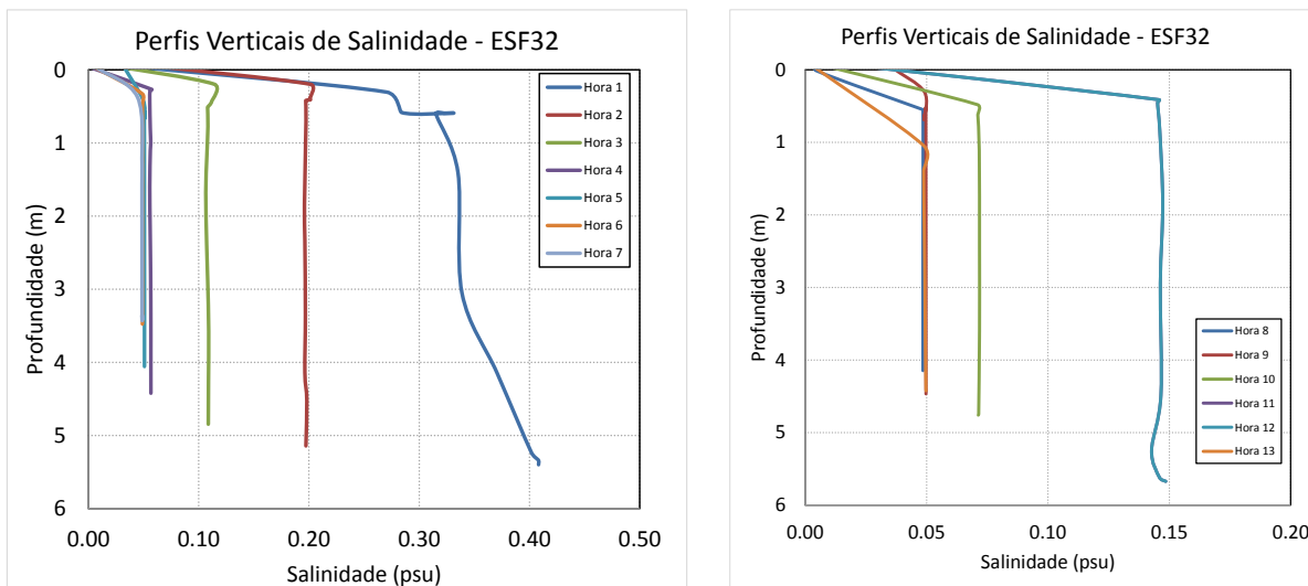
Figura 31- Perfis verticais de salinidade na estação fixa ESF_32. Campanha 26 - 24/10/2018. Resolução CONAMA 357/2005 (I - águas doces: águas com salinidade igual ou inferior a 0,5 ‰).
