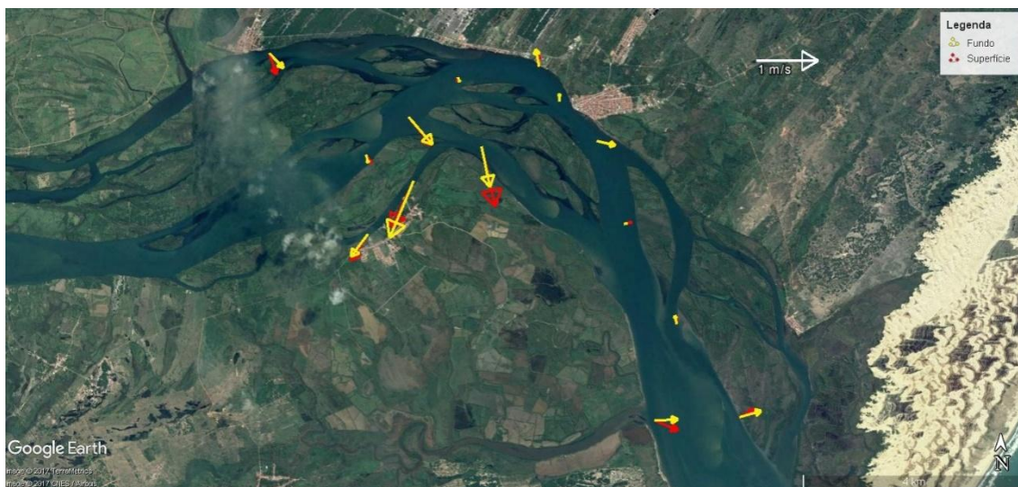
Figura 16 - Média vertical da velocidade e direção da corrente em cada estação amostral. Campanha 25 - Enchente 1 - 14/10/2018.
