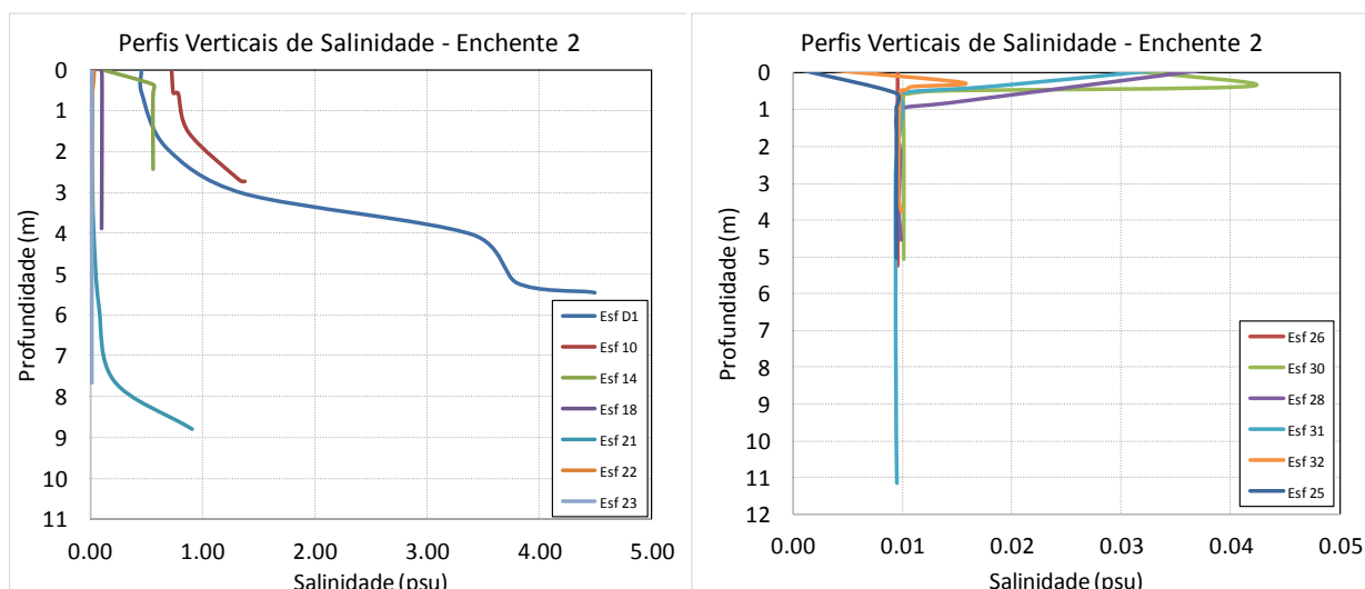
Figura 51 -Perfis verticais de salinidade para as estações amostrais. Campanha 26 - Enchente 2 - 26/10/2018.
