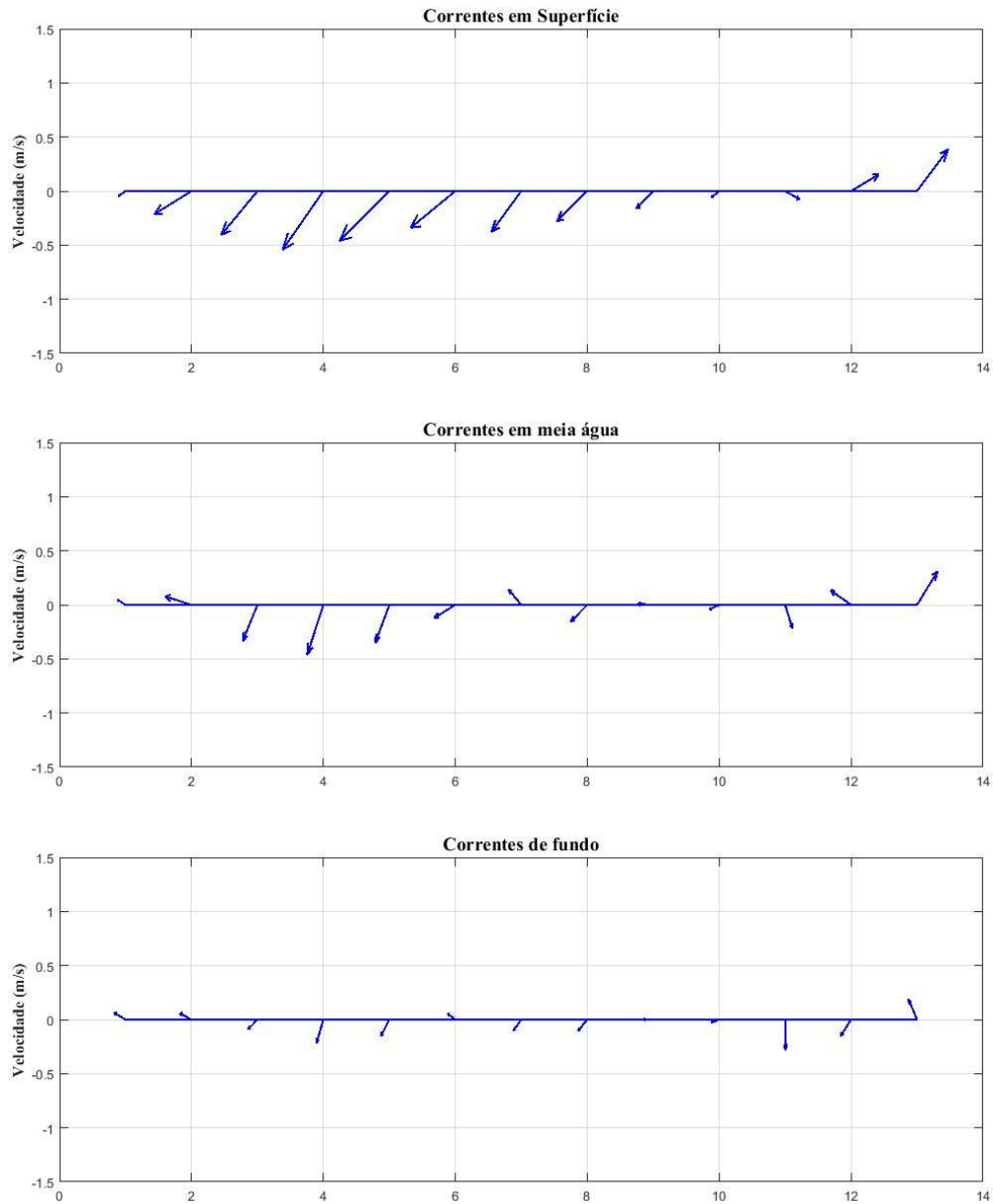
Figura 4 - Diagrama de vetores das correntes em superfície, meia água e fundo para a estação fixa ESF 32. Campanha 25 - 13/10/2018.
