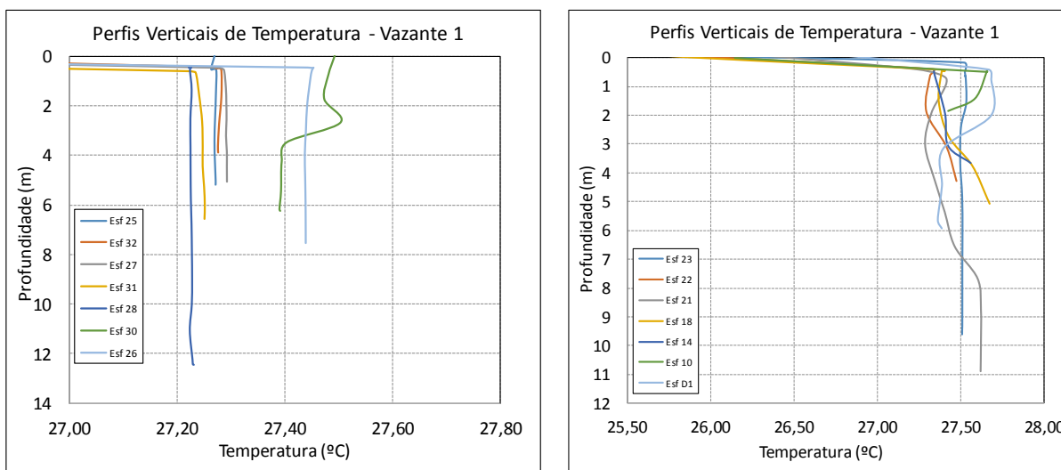
Figura 14 - Perfis verticais de temperatura para as estações amostrais. Campanha 25- Vazante 1 - 14/10/2018.
