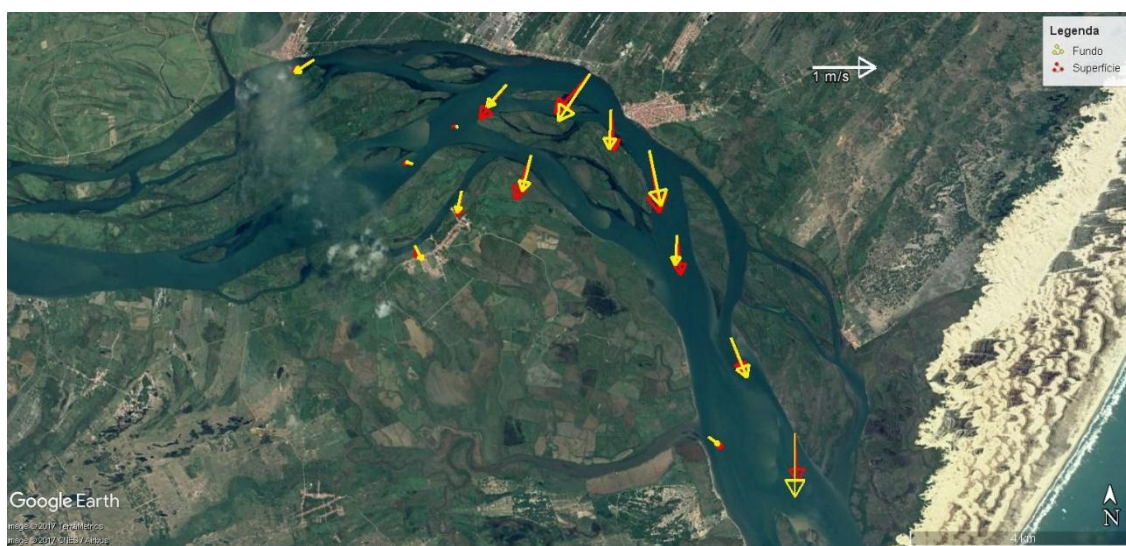
Figura 48 - Média vertical da velocidade e direção da corrente em cada estação amostral. Campanha 26 - Enchente 2 - 26/10/2018.
