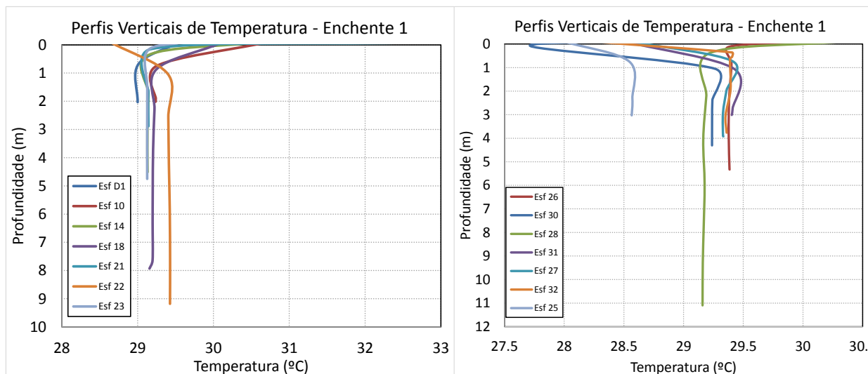
Figura 42 - Perfis verticais de temperatura para as estações amostrais. Campanha 26 - Enchente 1 - 25/10/2018.
