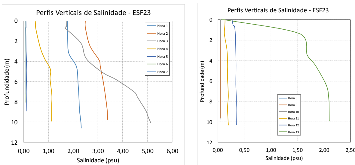
Figura 11 - Perfis verticais de salinidade para a estação amostral fixa ESF 23. Campanha 25 - 12/10/2018. Resolução CONAMA 357/2005 (I - águas doces: águas com salinidade igual ou inferior a 0,5 ‰).
