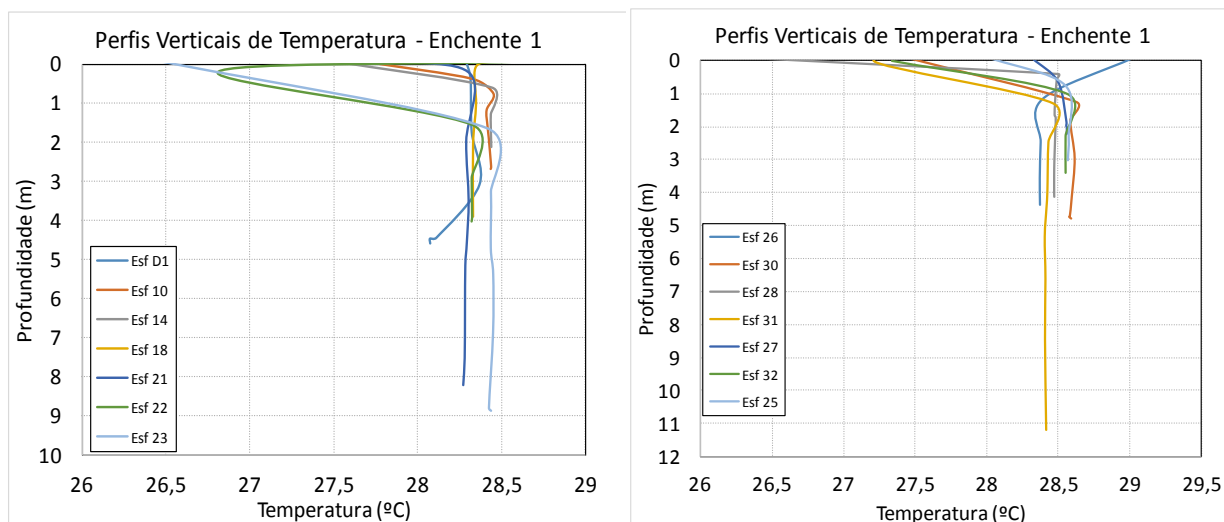
Figura 18 - Perfis verticais de temperatura para as estações amostrais. Campanha 25 - Enchente 1 - 14/10/2018.
