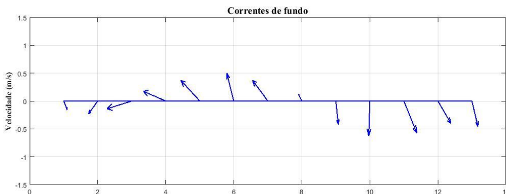
Figura 8 - Diagrama de vetores das correntes em superfície, meia água e fundo para a estação fixa ESF 23. Campanha 25 - 12/10/2018.
