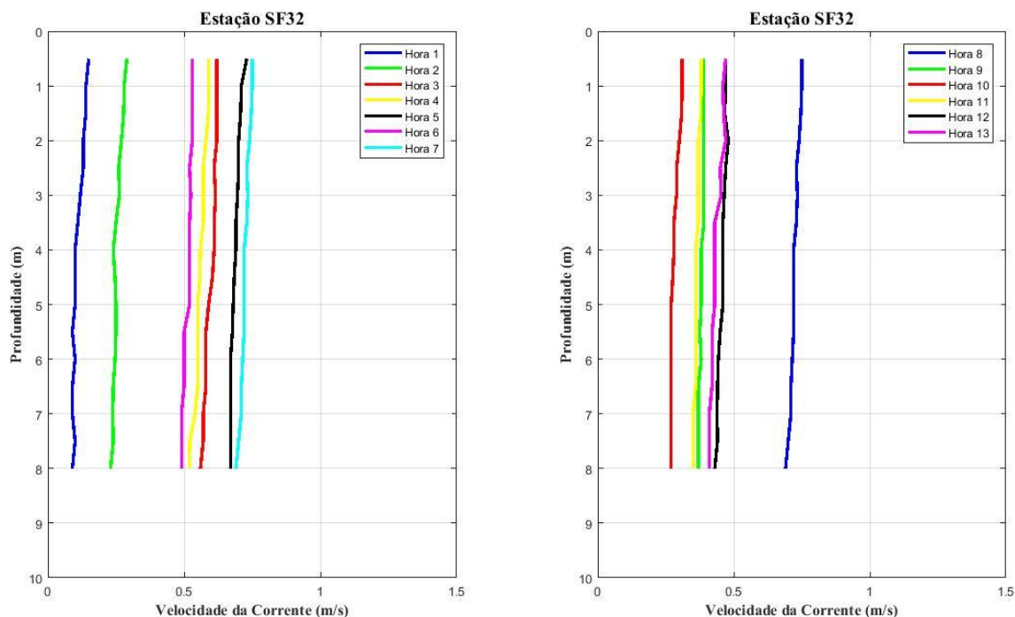
Figura 29 - Perfis verticais de velocidade de corrente na estação fixa ESF 32. Campanha 26 - 24/10/2018.
