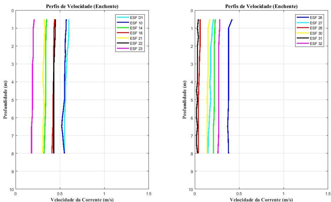
Figura 41 - Perfis verticais de velocidade de corrente para as estações amostrais em período de maré enchente. Campanha 26 - Enchente 1 - 25/10/2018.
