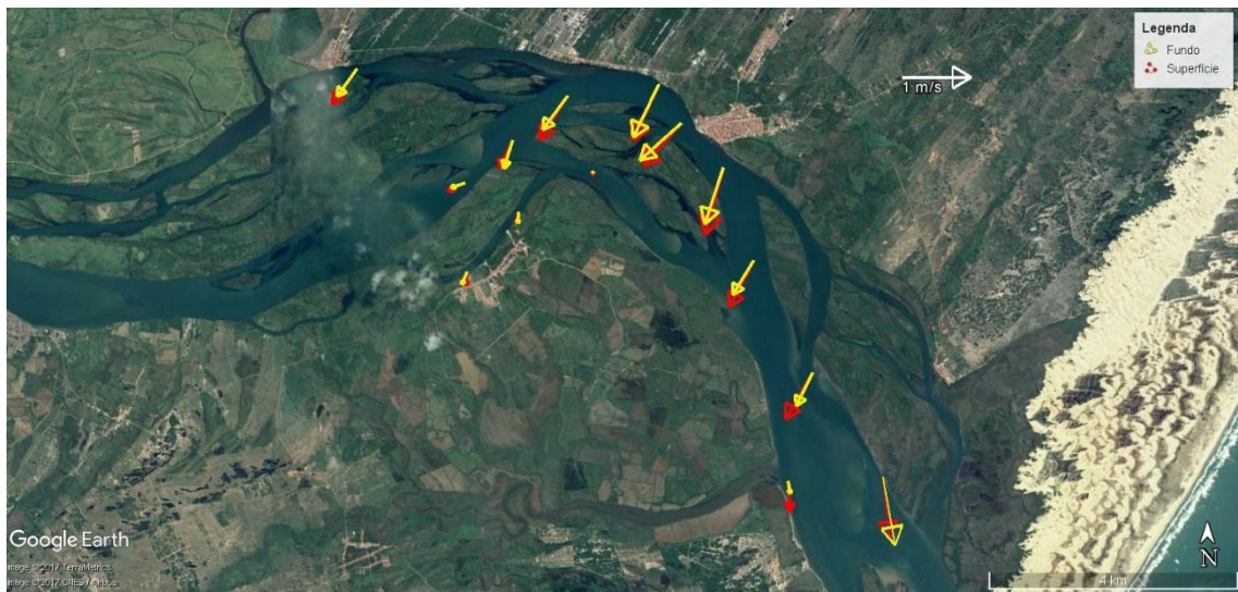
Figura 44 - Média vertical da velocidade e direção da corrente em cada estação amostral. Campanha 26 - Vazante 2-26/10/2018.
