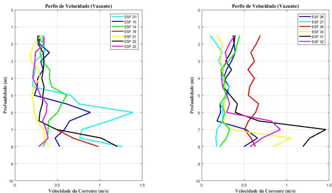
Figura 37 - Perfis verticais de velocidade de corrente para as estações amostrais em período de maré vazante Campanha 20 - Vazante 1 - 05/04/2018.
