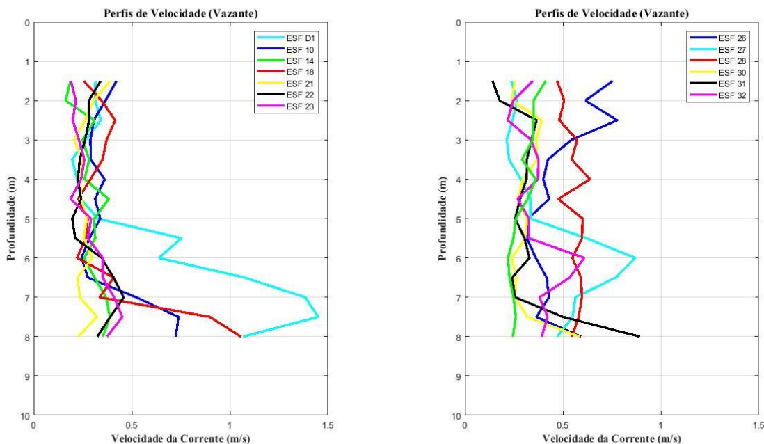
Figura 21 - Perfis verticais de velocidade de corrente para as estações amostrais em período de maré vazante. Campanha 19 - Vazante 2 - 21/03/2018.
