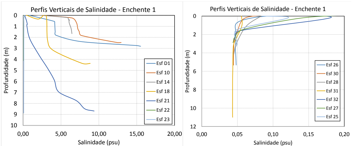
Figura 43 - Perfis verticais de salinidade para as estações amostrais. Campanha 20 - Enchente 1 - 05/04/2018.
