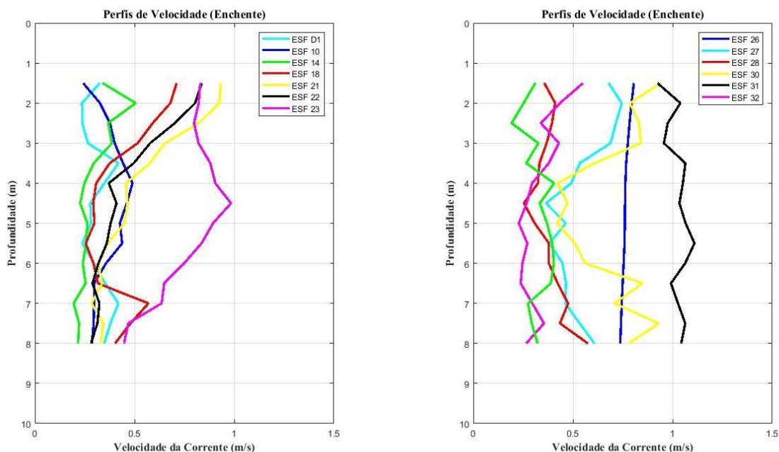
Figura 41 - Perfis verticais de velocidade de corrente para as estações amostrais em período de maré enchente. Campanha 20 - Enchente 1 - 05/04/2018.
