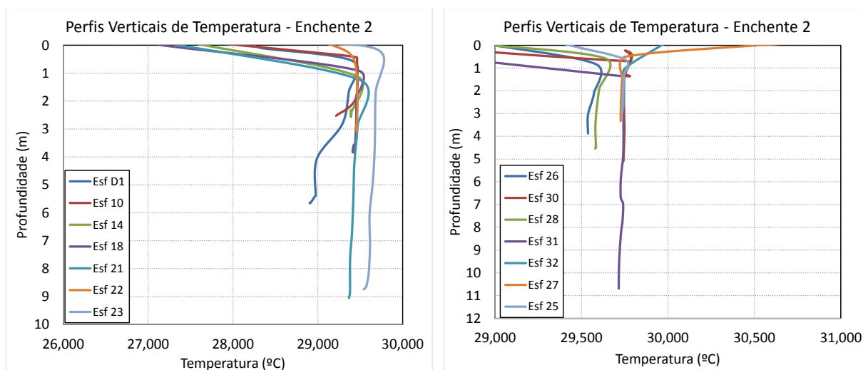
Figura 50 - Perfis verticais de temperatura para as estações amostrais. Campanha 20 - Enchente 2 - 06/04/2018.
