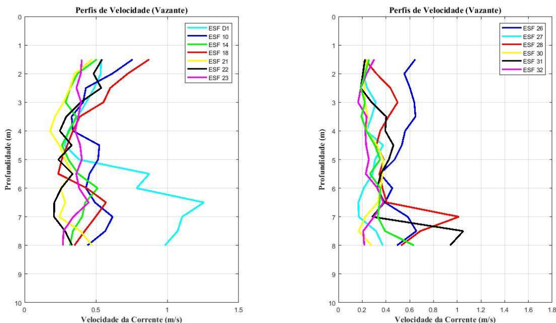
Figura 13 - Perfis verticais de velocidade de corrente para as estações amostrais em período de maré vazante. Campanha 19 - Vazante 1 - 20/03/2018.
