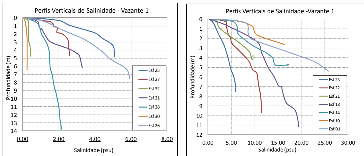
Figura 15 - Perfis verticais de salinidade para as estações amostrais. Campanha 19 - Vazante 1 - 20/03/2018. CONAMA 357/2005 (I - águas doces: águas com salinidade igual ou inferior a 0,5‰).
