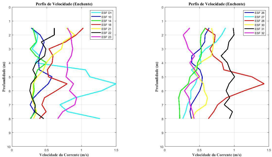
Figura 25 - Perfis verticais de velocidade de corrente para as estações amostrais em período de maré enchente. Campanha 19 - Enchente 2 - 21/03/2018.
