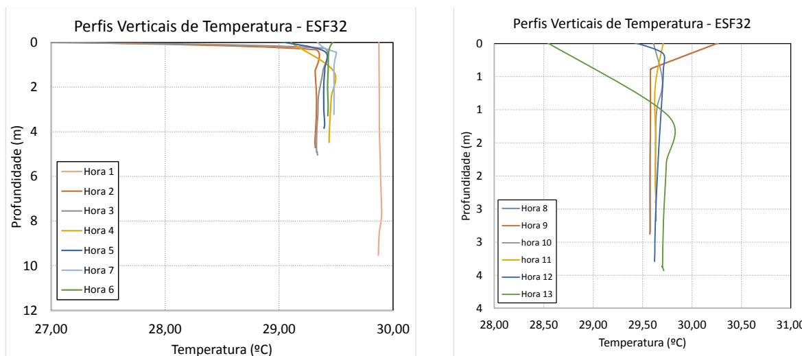
Figura 30- Perfis verticais de temperatura para a estação fixa ESF_32. Campanha 2 - 13 horas - Campanha 20 - 04/04/2018.
