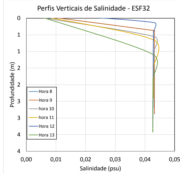
Figura 31- Perfis verticais de salinidade na estação fixa ESF_32. Campanha 20 - 04/04/2018. Resolução CONAMA 357/2005 (I - águas doces: águas com salinidade igual ou inferior a 0,5‰).
