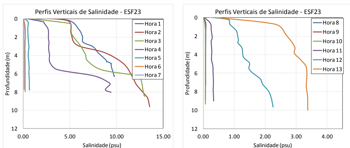
Figura 11 - Perfis verticais de salinidade para a estação amostral fixa ESF 23. Campanha 19 - 18/03/2018. Resolução CONAMA 357/2005 (I - águas doces: águas com salinidade igual ou inferior a 0,5‰).
