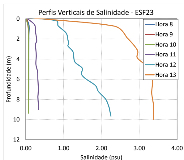
Figura 35 - Perfis verticais de salinidade na estação fixa ESF 23 Campanha 20 - 03/04/2018. Resolução CONAMA 357/2005 (I - águas doces: águas com salinidade igual ou inferior a 0,5‰).
