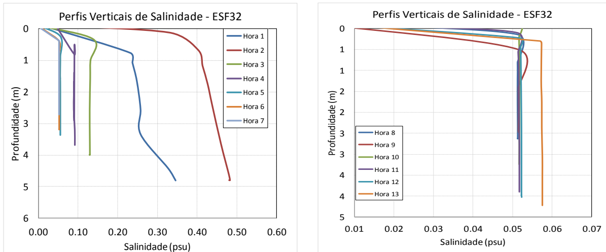
Figura 7 - Perfis verticais de salinidade para a estação amostral fixa ESF 32. Campanha 19 - 19/03/2018. Resolução CONAMA 357/2005 (I - águas doces: águas com salinidade igual ou inferior a 0,5‰).
