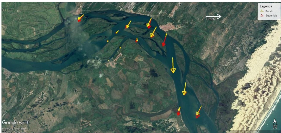
Figura 20 - Média vertical da velocidade e direção da corrente em cada estação amostral. Campanha 19 - Vazante 2 - 21/03/2018.
