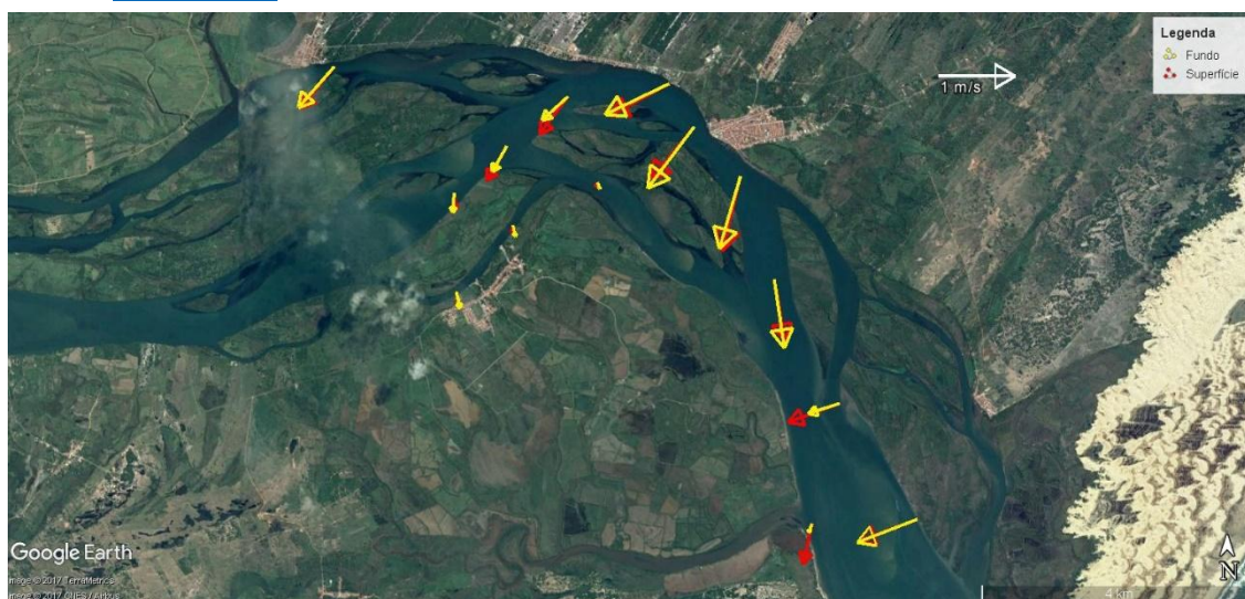
Figura 36 - Média vertical da velocidade e direção da corrente em cada estação amostral. Campanha 20 - Vazante 1 - 05/04/2018.
