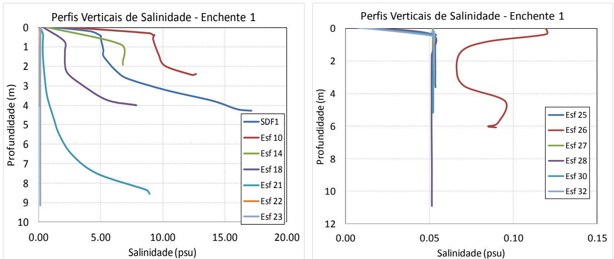
Figura 19 - Perfis verticais de salinidade para as estações amostrais. Campanha 19 - Enchente 1 - 20/03/2018. Resolução CONAMA 357/2005 (I - águas doces: águas com salinidade igual ou inferior a 0,5‰).
