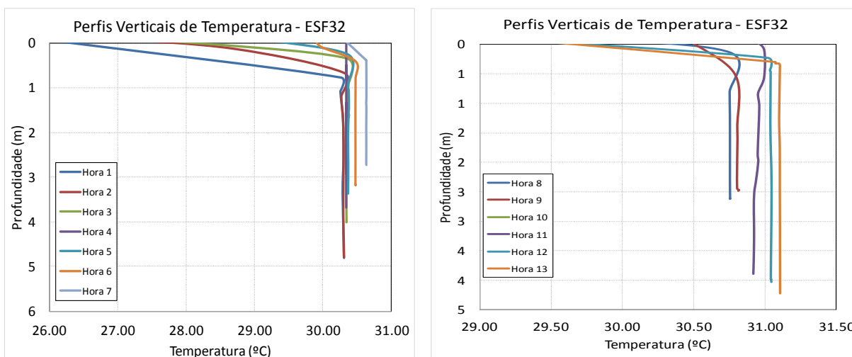
Figura 6 - Perfis verticais de temperatura para a estação amostral fixa ESF 32. Campanha 19 - Vazante 19/03/2018.
