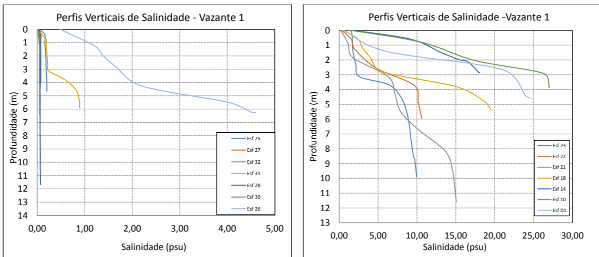
Figura 39 - Perfis verticais de salinidade para as estações amostrais. Campanha 20 - Vazante 1 - 05/04/2018.
