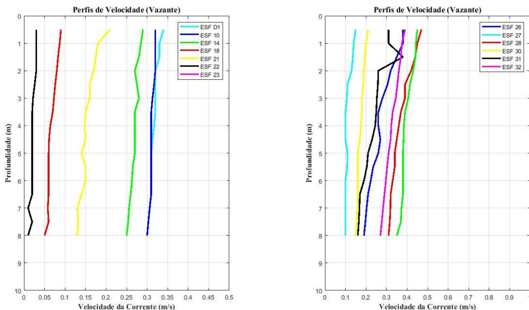
Figura 45 - Perfis verticais de velocidade de corrente para as estações amostrais em período de maré vazante. Campanha 20 - Vazante 2 - 06/04/2018.
