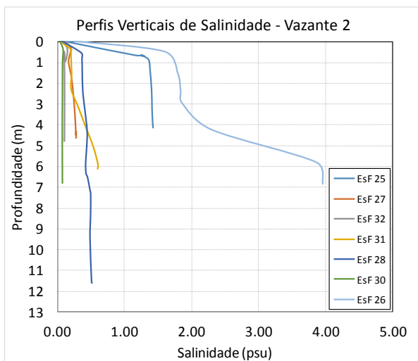
Figura 23 - Perfis verticais de salinidade para as estações amostrais. Campanha 19 - Vazante 2 - 21/03/2018. Resolução CONAMA 357/2005 (I - águas doces: águas com salinidade igual ou inferior a 0,5‰).
