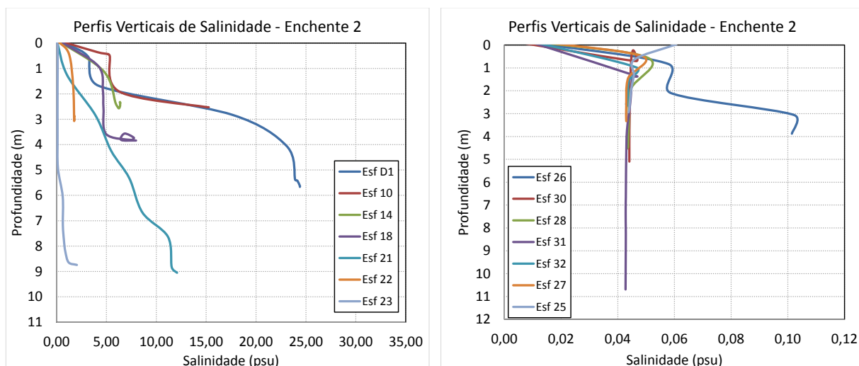
Figura 51 - Perfis verticais de salinidade para as estações amostrais. Campanha 20 - Enchente 2 - 06/04/2018.
