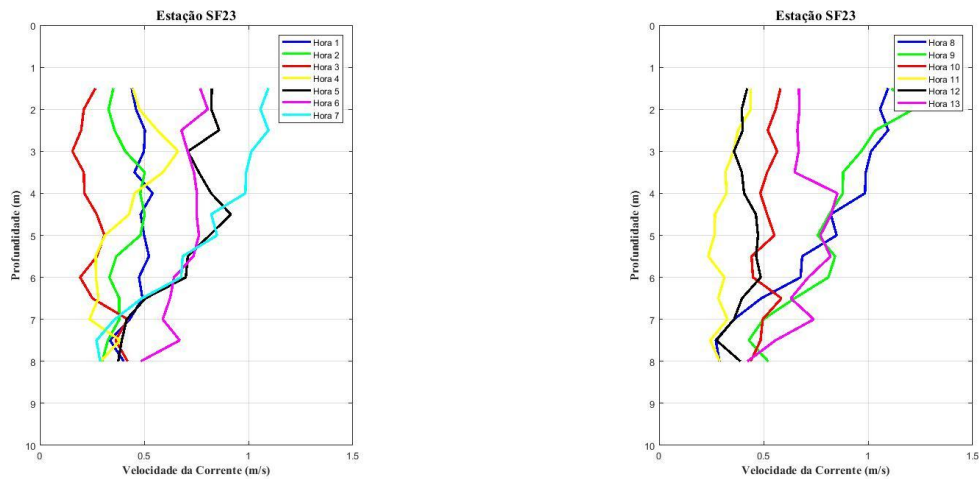
Figura 33 - Perfis verticais de velocidade de corrente na estação fixa ESF 23. Campanha 20 - 03/04/2018.
