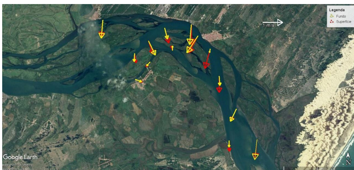
Figura 12 - Média vertical da velocidade e direção da corrente em cada estação amostral. Campanha 19 - Vazante 1 - 20/03/2018.
