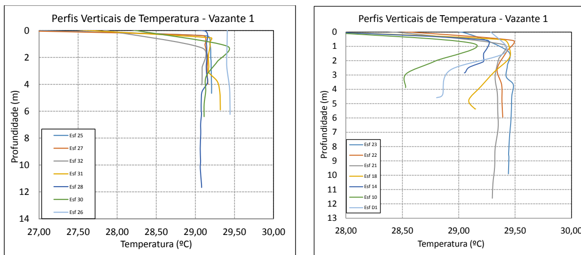
Figura 38 - Perfis verticais de temperatura para as estações amostrais. Campanha 20 – Vazante 1 - 05/04/2018.
