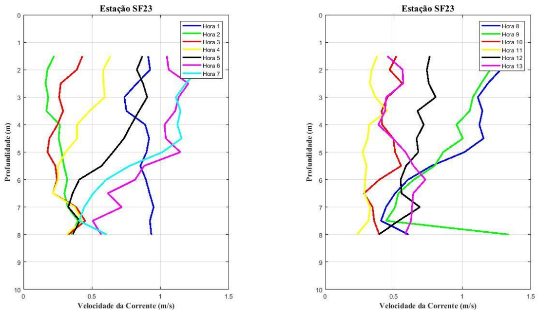
Figura 9 - Perfis verticais de velocidade de corrente na estação fixa ESF 23. Campanha 19 - 18/03/2018.
