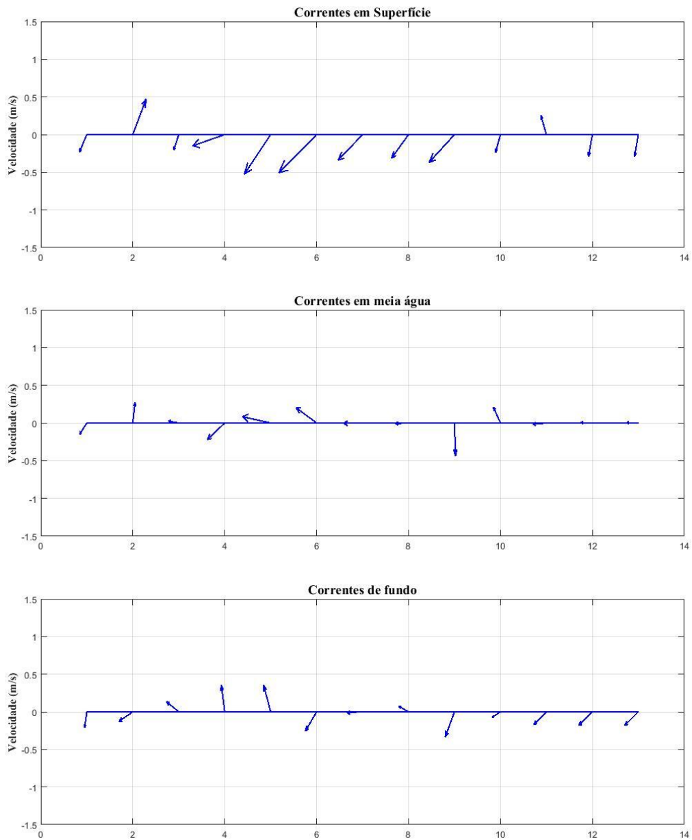
Figura 4 - Diagrama de vetores das correntes em superfície, meia água e fundo para a estação fixa ESF 32. Campanha 19 - 19/03/2018.
