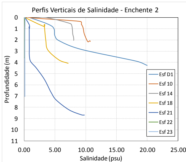
Figura 27 - Perfis verticais de salinidade para as estações amostrais. Campanha 19 - Enchente 2 - 21/03/2018. Resolução CONAMA 357/2005 (I - águas doces: águas com salinidade igual ou inferior a 0,5‰).
