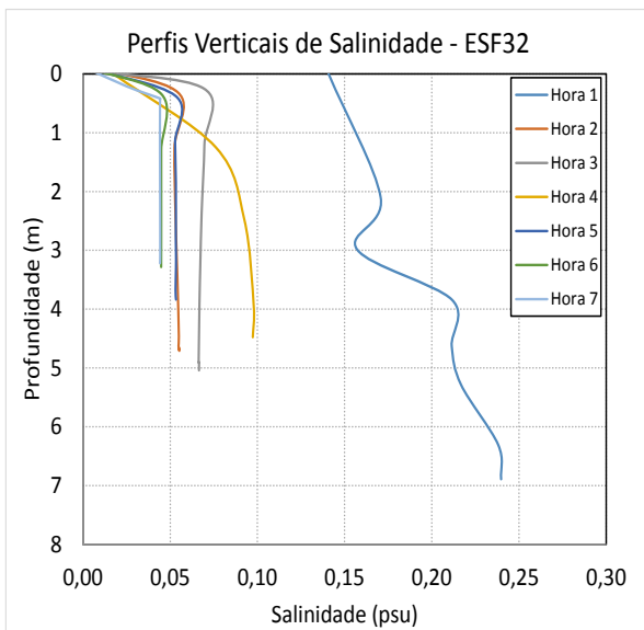
Figura 31- Perfis verticais de salinidade na estação fixa ESF_32. Campanha 20 - 04/04/2018. Resolução CONAMA 357/2005 (I - águas doces: águas com salinidade igual ou inferior a 0,5‰).
