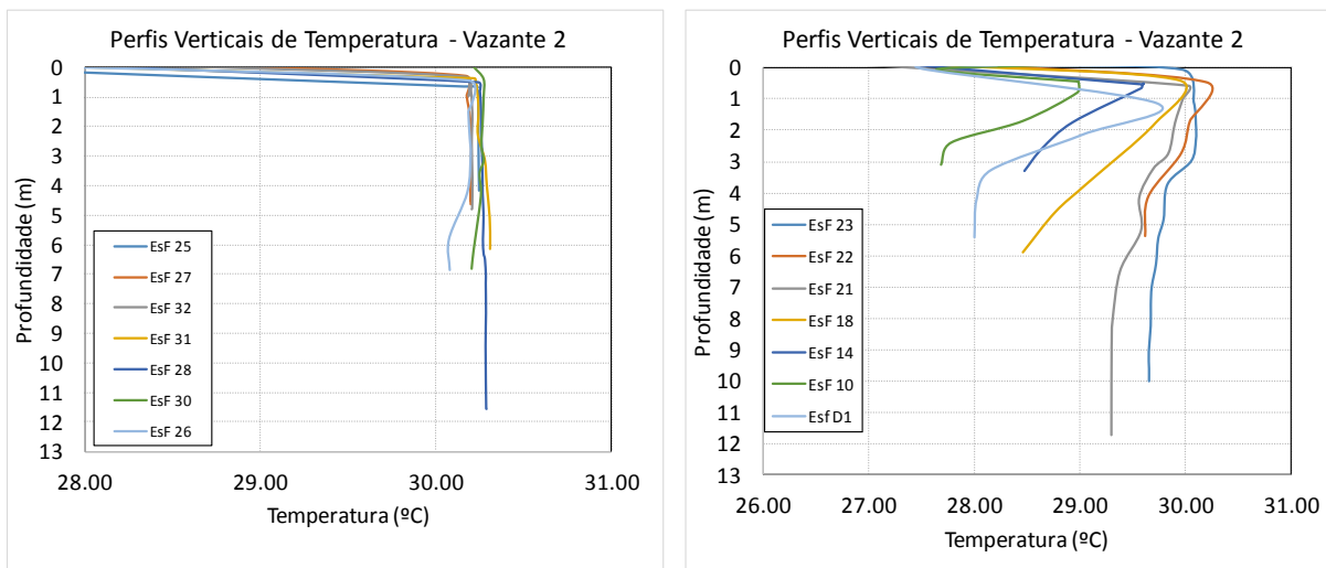
Figura 22 - Perfis verticais de temperatura para as estações amostrais. Campanha 19 - Vazante 2 - 21/03/2018.
