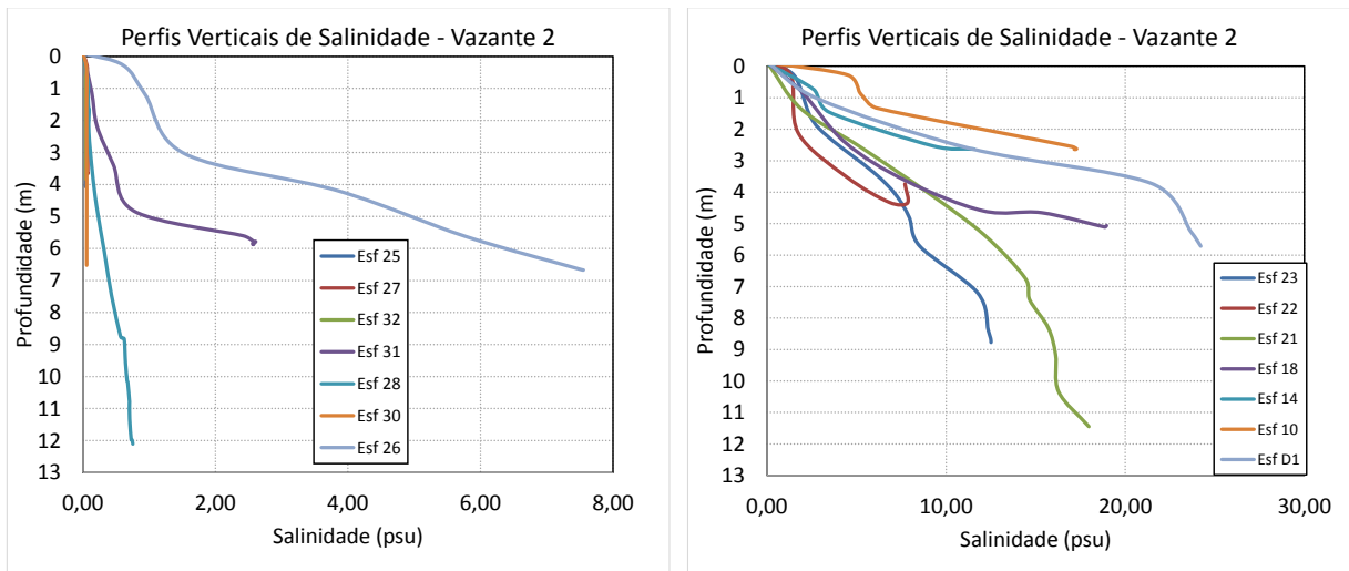
Figura 47 - Perfis verticais de salinidade para as estações amostrais. Campanha 20 - Vazante 2 - 06/04/2018.
