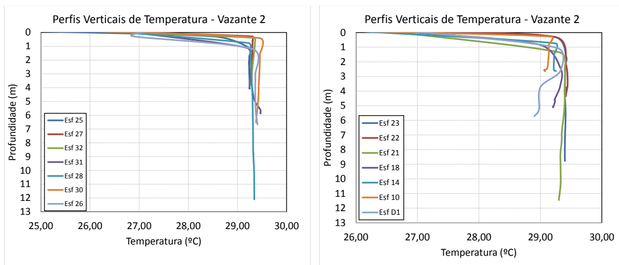
Figura 46 - Perfis verticais de temperatura para as estações amostrais. Campanha 20 - Vazante 2 - 06/04/2018.
