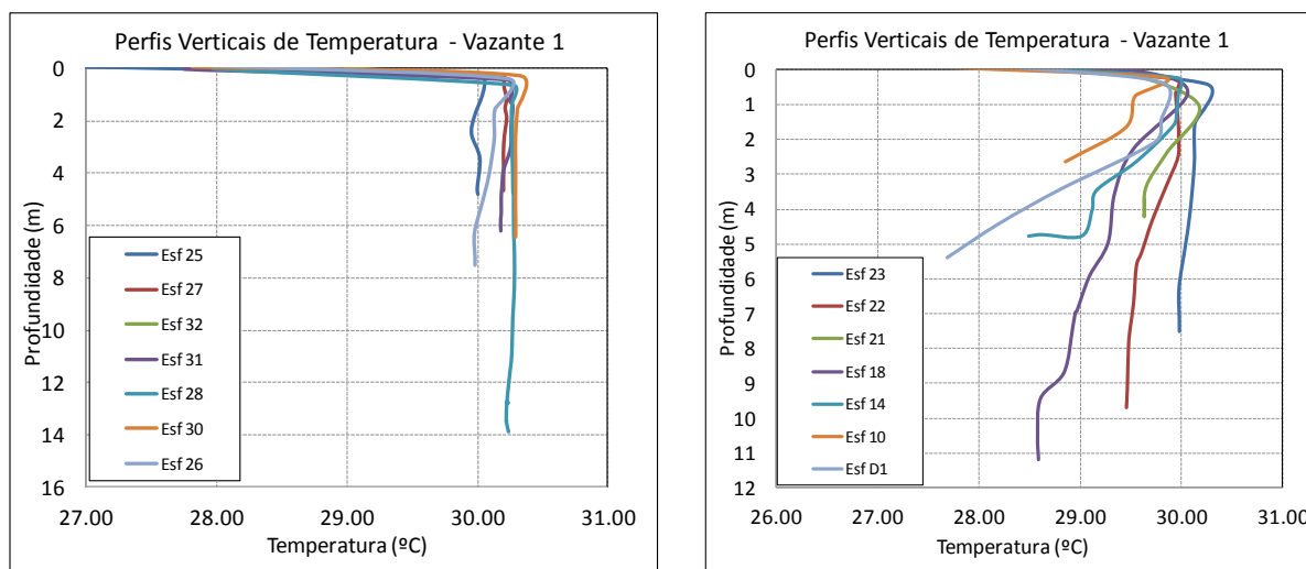
Figura 14 - Perfis verticais de temperatura para as estações amostrais. Campanha 19- Vazante 1 - 20/03/2018.
