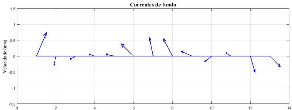
Figura 8 - Diagrama de vetores das correntes em superfície, meia água e fundo para a estação fixa ESF 23. Campanha 19 - 18/03/2018.
