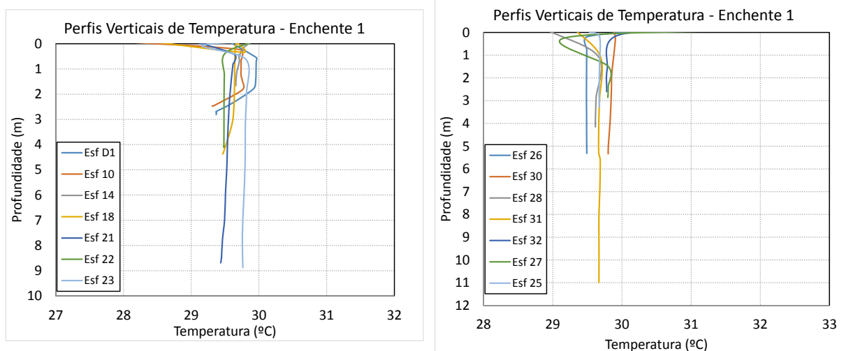
Figura 42 - Perfis verticais de temperatura para as estações amostrais. Campanha 20 - Enchente 1 - 05/04/2018.
