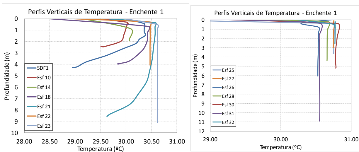
Figura 18 - Perfis verticais de temperatura para as estações amostrais. Campanha 19 - Enchente 1 - 16/02/2018.
