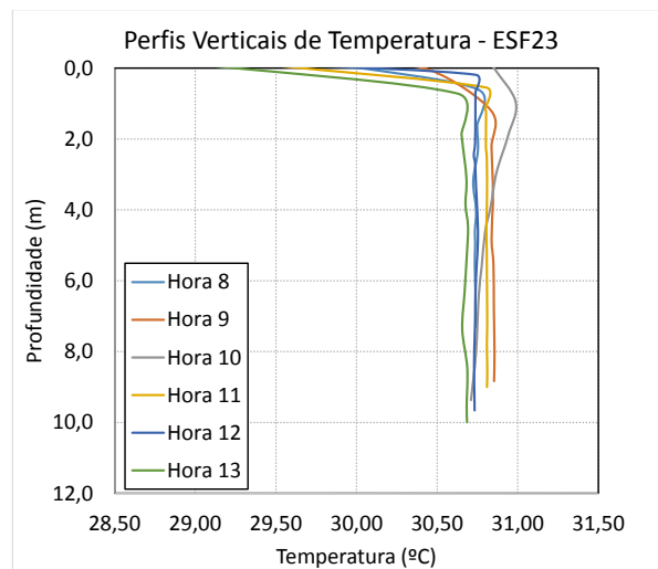
Figura 34 - Perfis verticais de temperatura para a estação fixa na estação fixa ESF 23. Campanha 20 - 03/04/2018.
