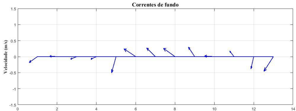
Figura 32 - Diagrama de vetores das correntes em superfície, meia água e fundo para a estação fixa ESF 23. Campanha 20 - 03/04/2018.
