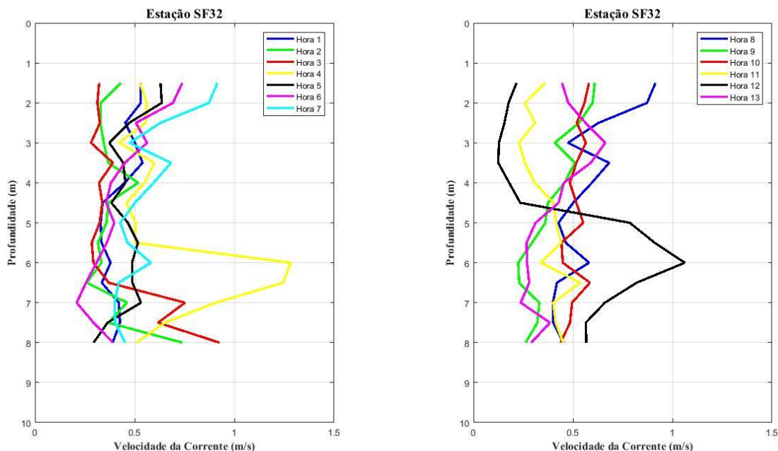
Figura 29 - Perfis verticais de velocidade de corrente na estação fixa ESF 32. Campanha 20 - 04/04/2018.
