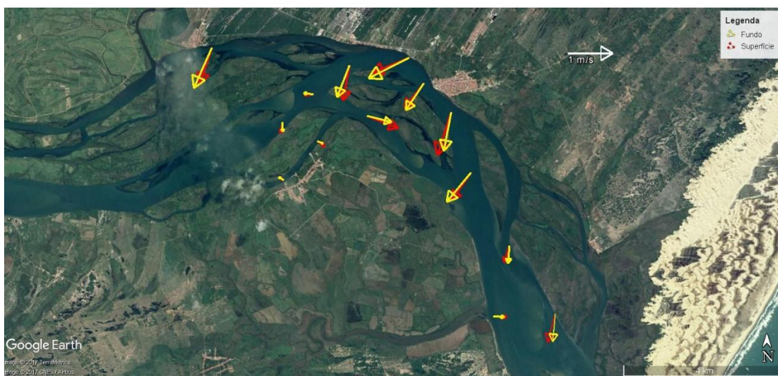
Figura 40 - Média vertical da velocidade e direção da corrente em cada estação amostral. Campanha 20 - Enchente 1 - 05/04/2018.
