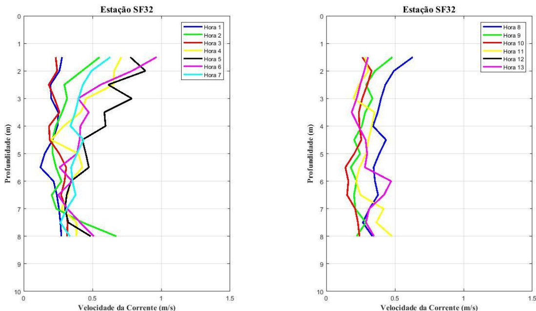
Figura 5 - Perfis verticais de velocidade de corrente na estação fixa ESF 32. Campanha 19 - 19/03/2018.
