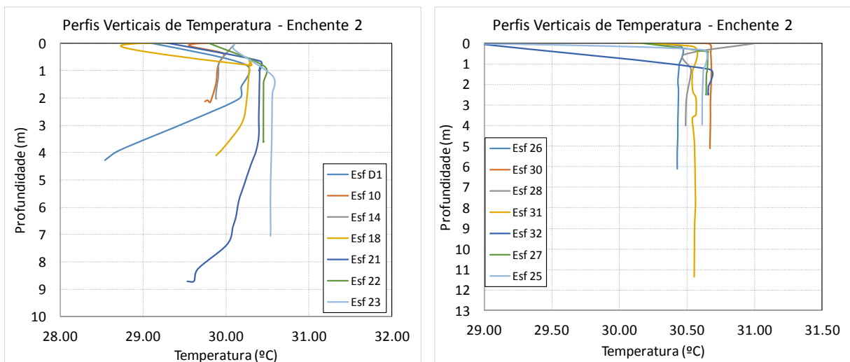
Figura 26 - Perfis verticais de temperatura para as estações amostrais. Campanha 19 - Enchente 2 - 21/03/2018.
