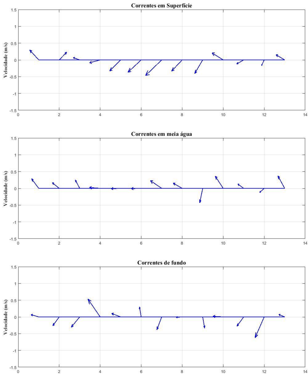
Figura 28 - Diagrama de vetores das correntes em superfície, meia água e fundo para a estação fixa ESF 32. Campanha 20 - 04/04/2018.
