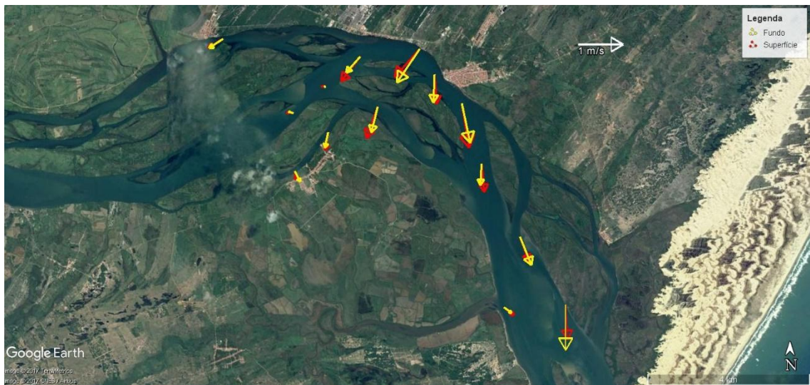
Figura 48 - Média vertical da velocidade e direção da corrente em cada estação amostral. Campanha 20 - Enchente 2 - 06/04/2018.
