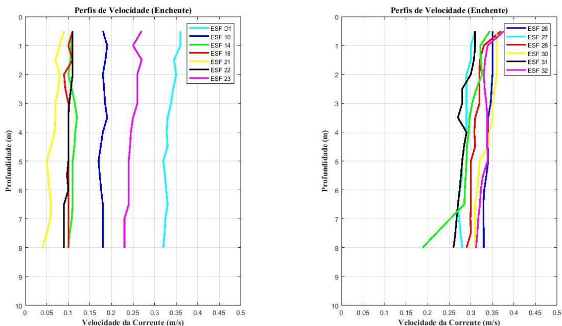
Figura 49 - Perfis verticais de velocidade de corrente para as estações amostrais em período de maré enchente. Campanha 20 - Enchente 2 - 06/04/2018.
