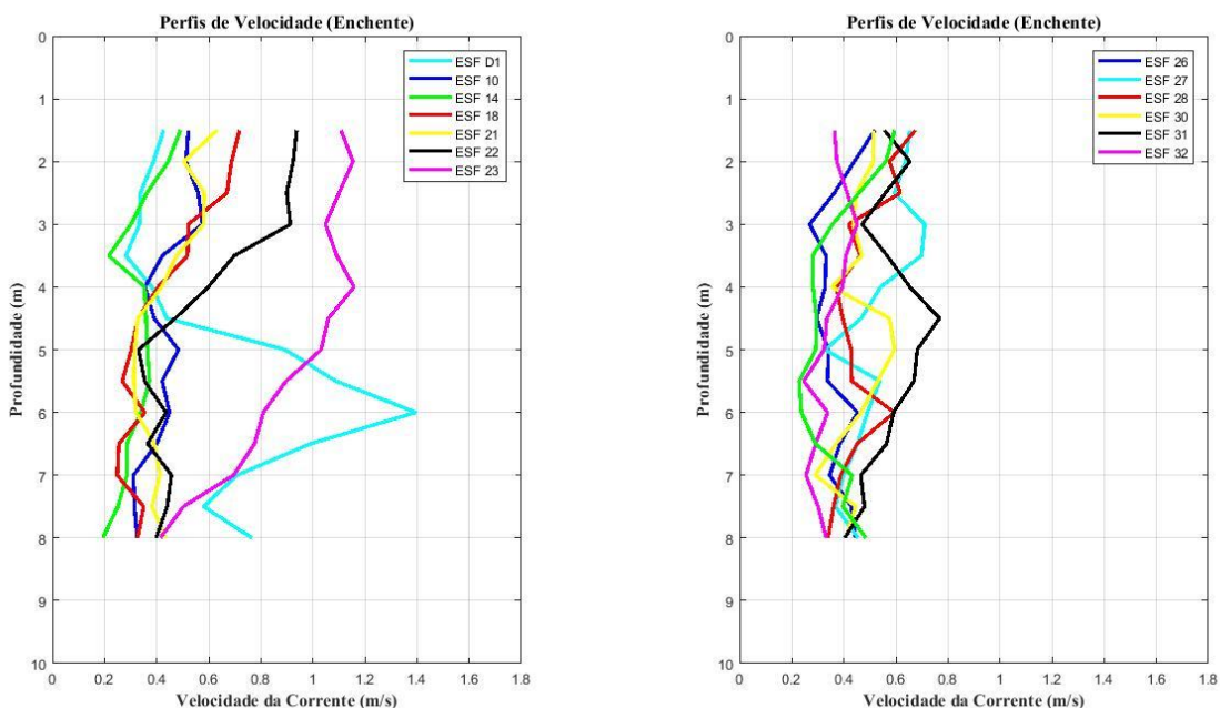
Figura 17 - Perfis verticais de velocidade de corrente para as estações amostrais em período de maré enchente. Campanha 19 - Enchente 1 - 20/03/2018.
