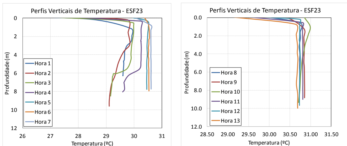
Figura 10 - Perfis verticais de temperatura para a estação amostral fixa ESF 23. Campanha 19 - 18/03/2018.
