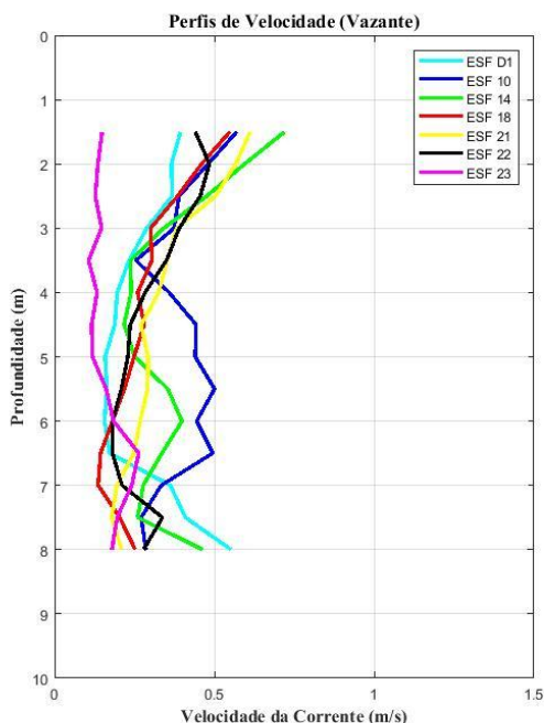
Figura 21 - Perfis verticais de velocidade de corrente para as estações amostrais em período de maré vazante. Campanha 15 - Vazante 2 - 07/01/2018.
