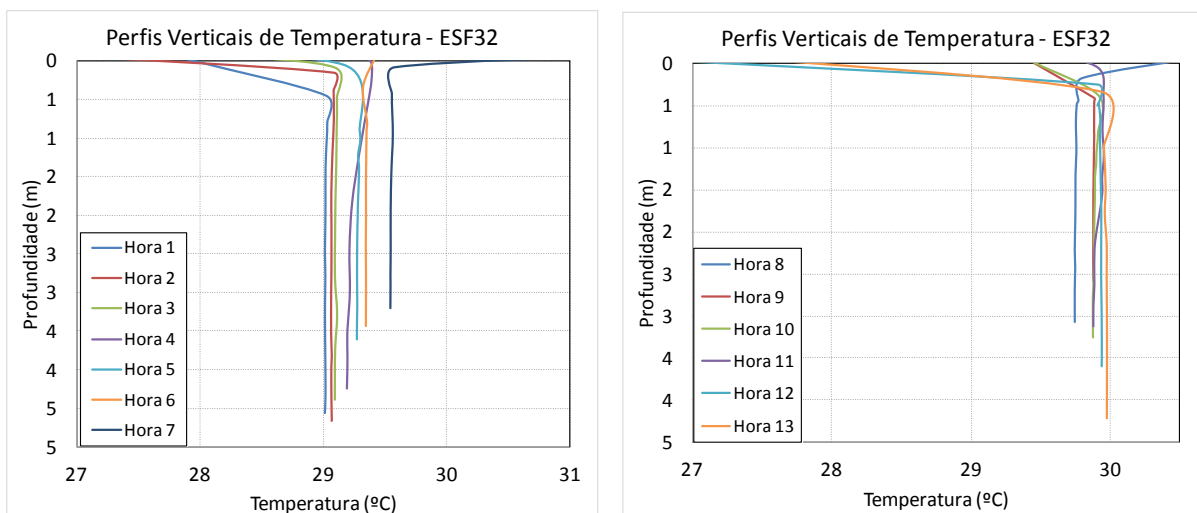
Figura 6 - Perfis verticais de temperatura para a estação amostral fixa ESF 32. Campanha 15 - Vazante 06/01/2018.
