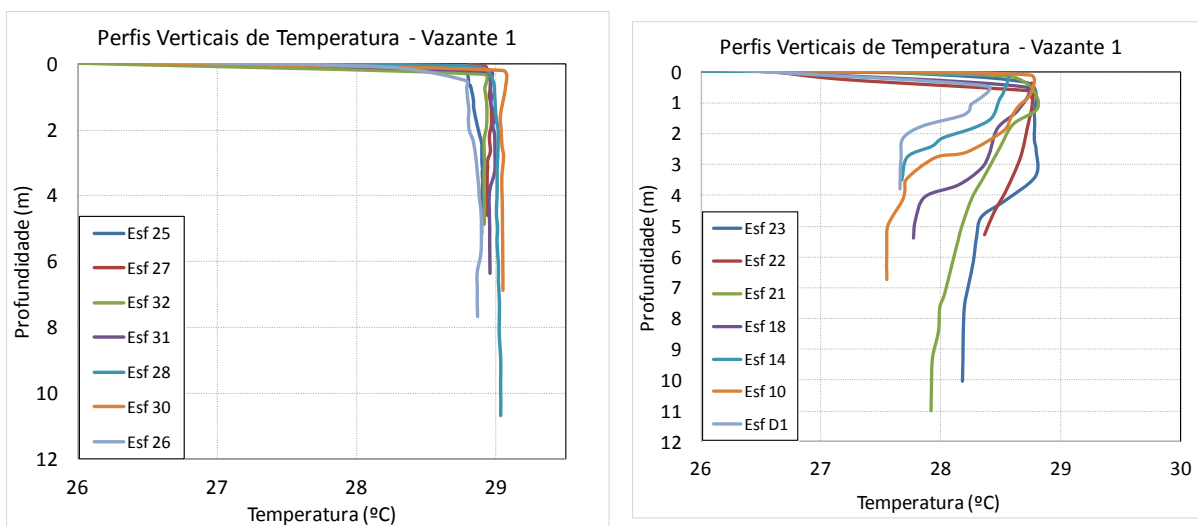
Figura 14 - Perfis verticais de temperatura para as estações amostrais. Campanha 15- Vazante 1 - 04/01/2018.
