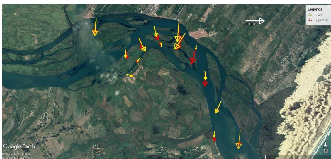
Figura 12 - Média vertical da velocidade e direção da corrente em cada estação amostral. Campanha 15 - Vazante 1 - 04/01/2018.
