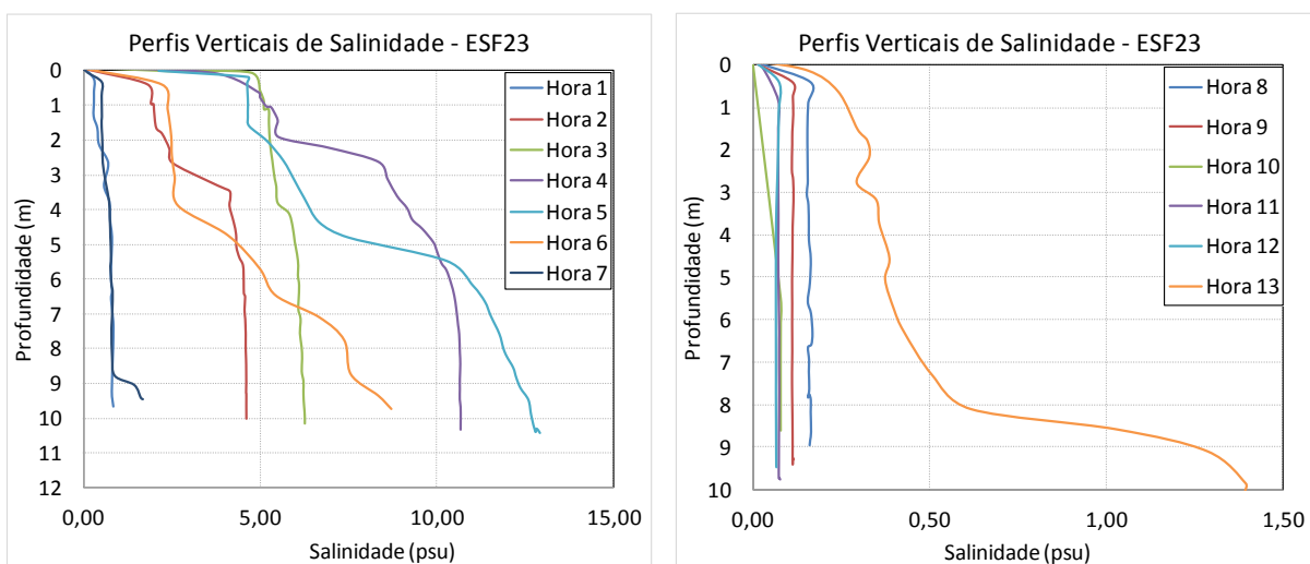
Figura 11 - Perfis verticais de salinidade para a estação amostral fixa ESF 23. Campanha 15 - 05/01/2018. Resolução CONAMA 357/2005 (I - águas doces: águas com salinidade igual ou inferior a 0,5‰).
