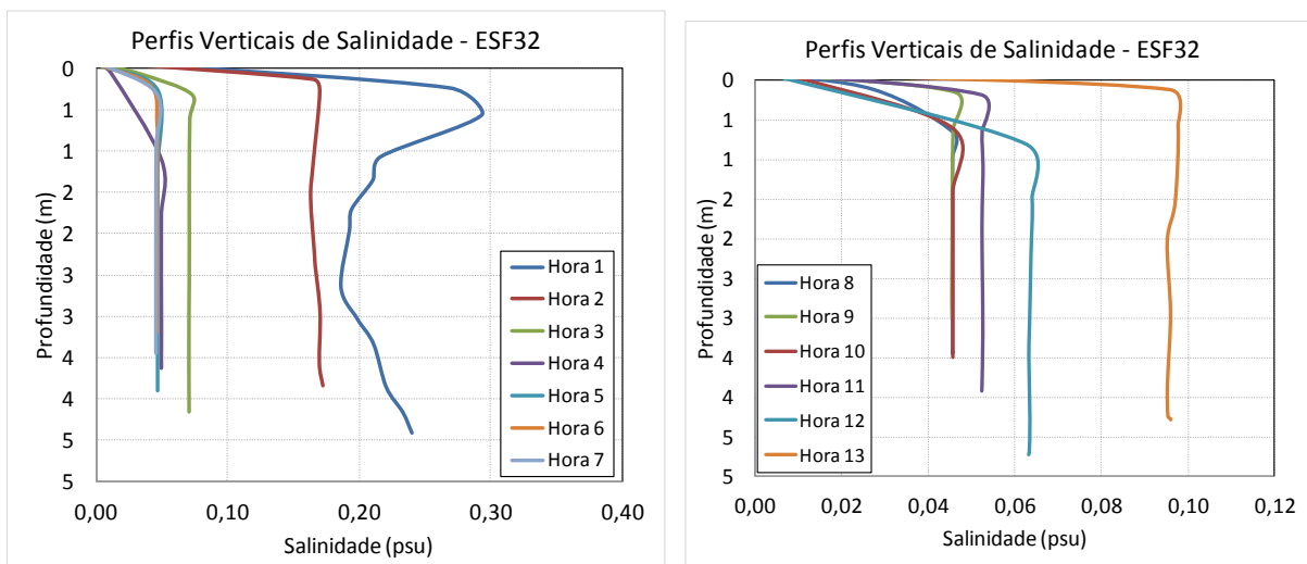
Figura 31- Perfis verticais de salinidade na estação fixa ESF_32. Campanha 16 - 17/01/2018. Resolução CONAMA 357/2005 (I - águas doces: águas com salinidade igual ou inferior a 0,5‰).
