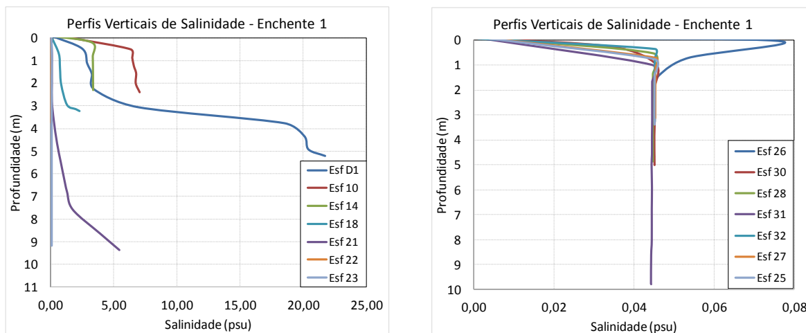
Figura 43 - Perfis verticais de salinidade para as estações amostrais. Campanha 16 - Enchente 1 - 20/01/2018.
