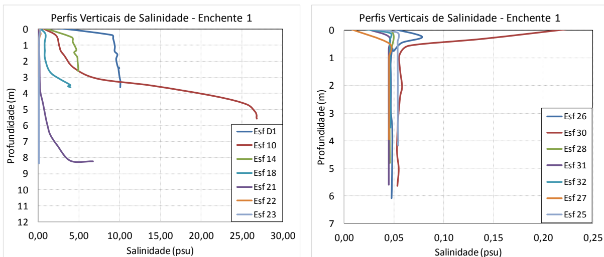
Figura 19 - Perfis verticais de salinidade para as estações amostrais. Campanha 15 - Enchente 1 - 04/01/2018. Resolução CONAMA 357/2005 (I - águas doces: águas com salinidade igual ou inferior a 0,5‰).
