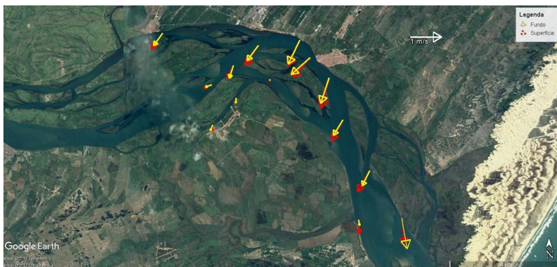
Figura 44 - Média vertical da velocidade e direção da corrente em cada estação amostral. Campanha 16 - Vazante 2 - 21/01/2018.
