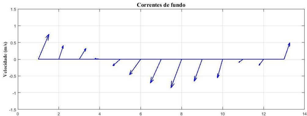
Figura 8 - Diagrama de vetores das correntes em superfície, meia água e fundo para a estação fixa ESF 23. Campanha 15 - 05/01/2018.
