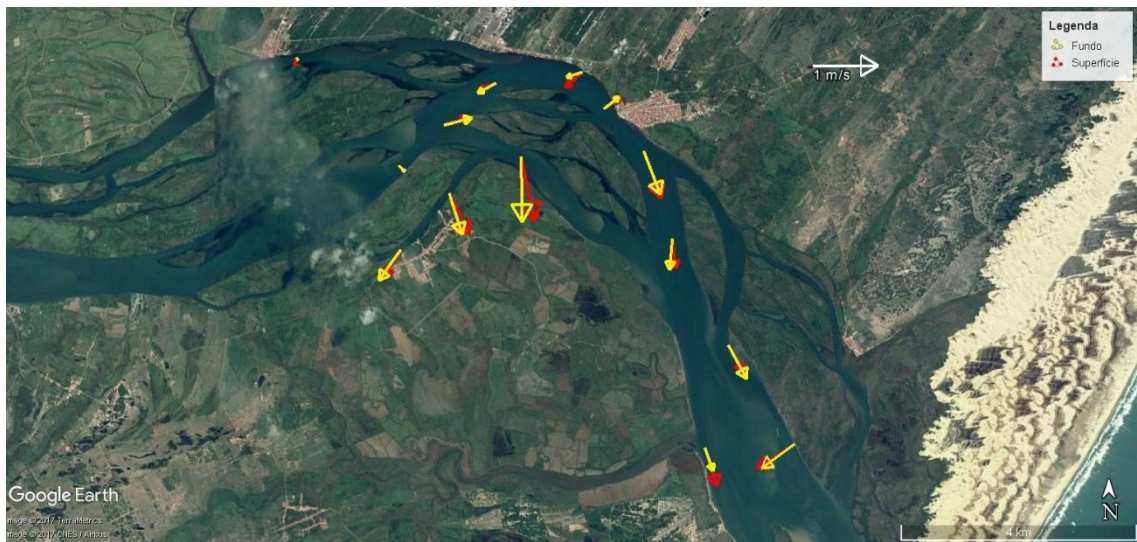
Figura 24 - Média vertical da velocidade e direção da corrente em cada estação amostral. Campanha 15 - Enchente 2 - 07/01/2018.
