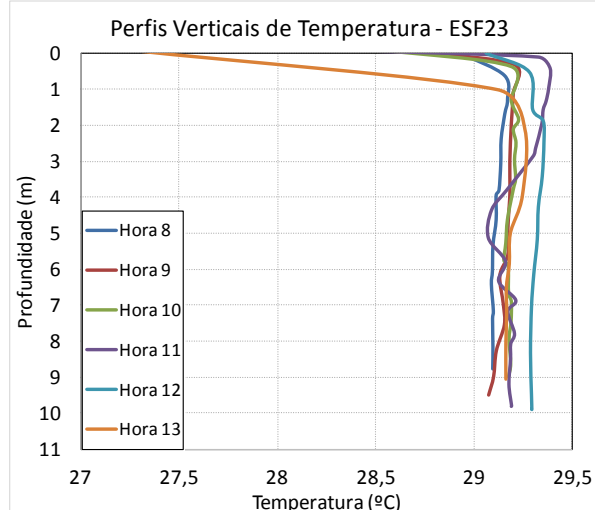
Figura 34 - Perfis verticais de temperatura para a estação fixa na estação fixa ESF 23. Campanha 16 - 18/01/2018.
