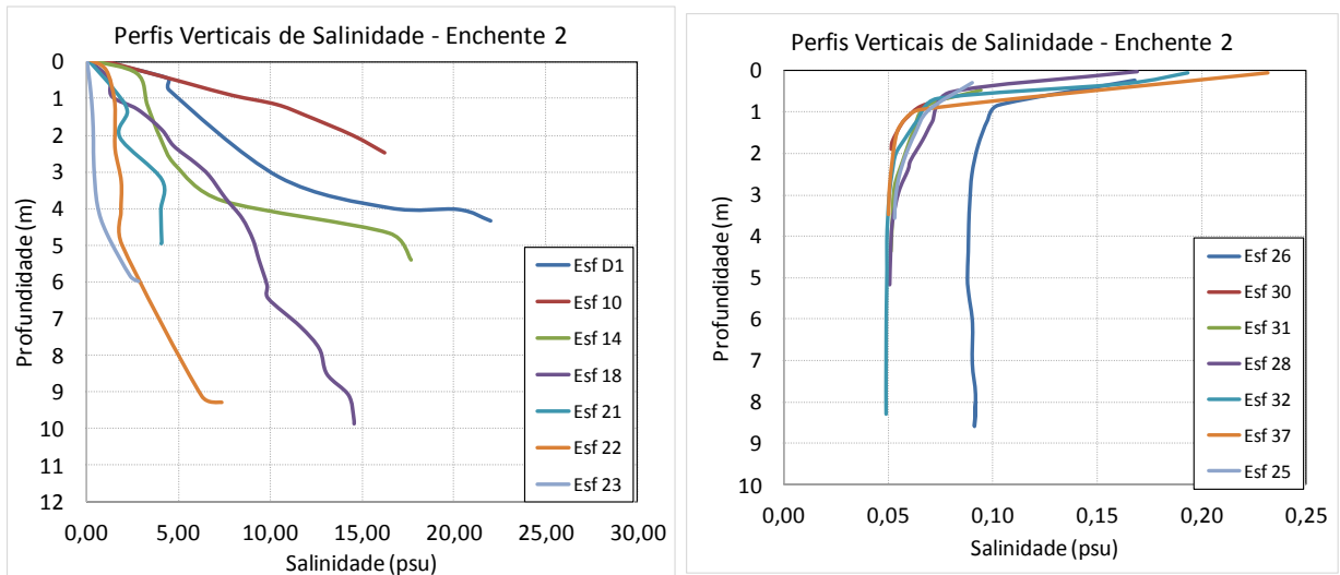
Figura 27 - Perfis verticais de salinidade para as estações amostrais. Campanha 15 - Enchente 2 - 07/01/2018. Resolução CONAMA 357/2005 (I - águas doces: águas com salinidade igual ou inferior a 0,5‰).
