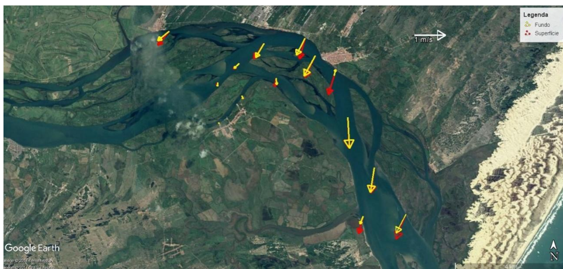
Figura 20 - Média vertical da velocidade e direção da corrente em cada estação amostral. Campanha 15 - Vazante 2 - 07/01/2018.
