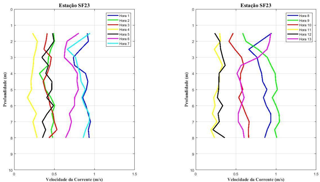
Figura 9 - Perfis verticais de velocidade de corrente na estação fixa ESF 23. Campanha 15 - 05/01/2018.
