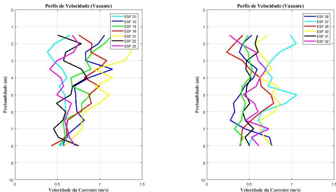
Figura 37 - Perfis verticais de velocidade de corrente para as estações amostrais em período de maré vazante Campanha 16 - Vazante 1 - 20/01/2018.
