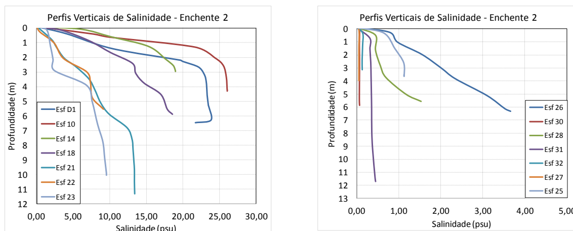
Figura 51 - Perfis verticais de salinidade para as estações amostrais. Campanha 16 - Enchente 2 - 21/01/2018.
