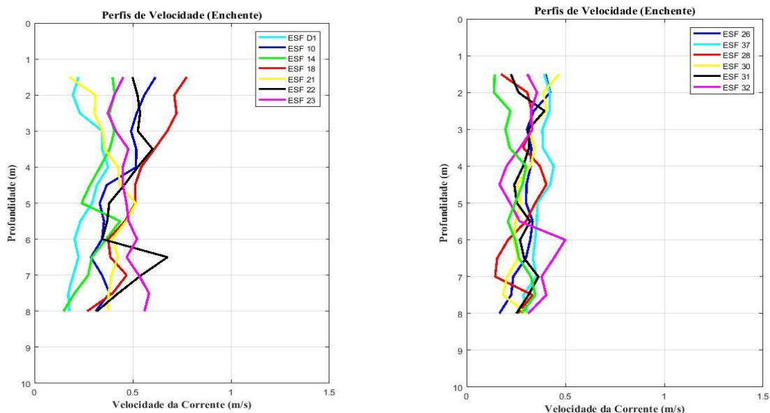
Figura 41 - Perfis verticais de velocidade de corrente para as estações amostrais em período de maré enchente. Campanha 16 - Enchente 1 - 20/01/2018.
