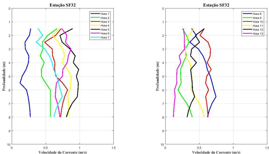
Figura 29 - Perfis verticais de velocidade de corrente na estação fixa ESF 32. Campanha 16 - 17/01/2018.
