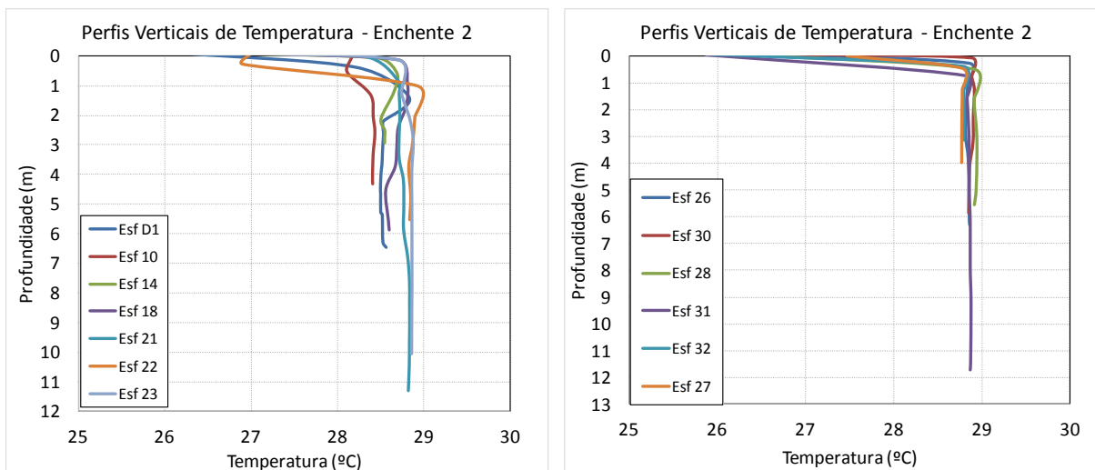
Figura 50 - Perfis verticais de temperatura para as estações amostrais. Campanha 16 - Enchente 2 - 21/01/2018.
