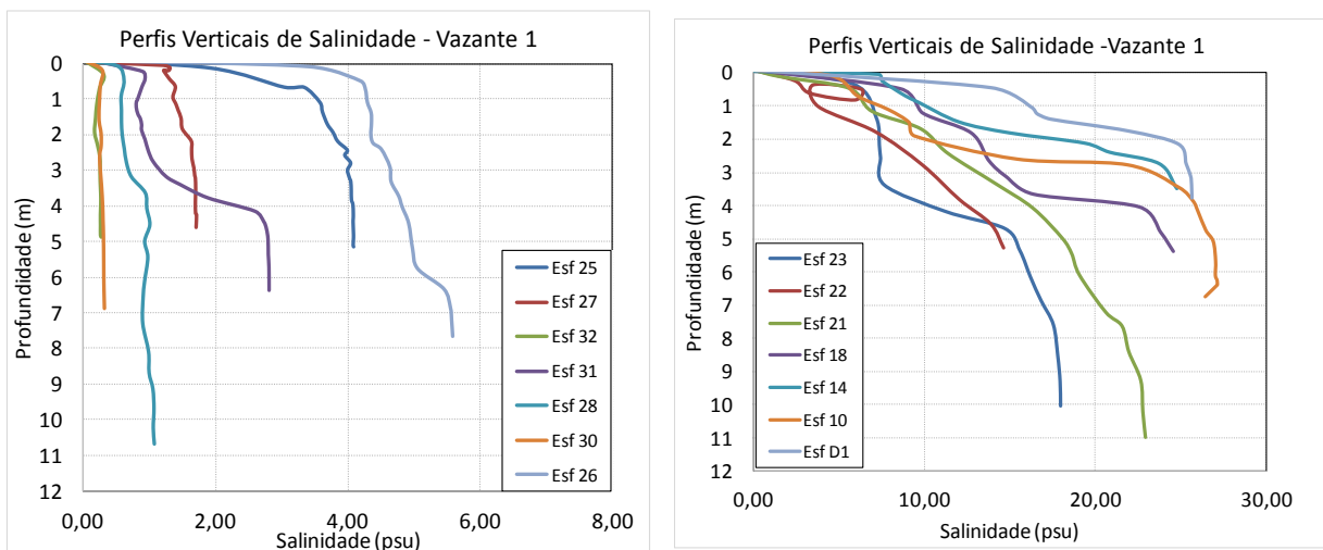
Figura 15 - Perfis verticais de salinidade para as estações amostrais. Campanha 15 - Vazante 1 - 04/01/2018. CONAMA 357/2005 (I - águas doces: águas com salinidade igual ou inferior a 0,5‰).
