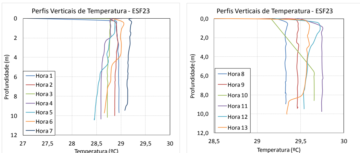
Figura 10 - Perfis verticais de temperatura para a estação amostral fixa ESF 23. Campanha 15 - 05/01/2018.
