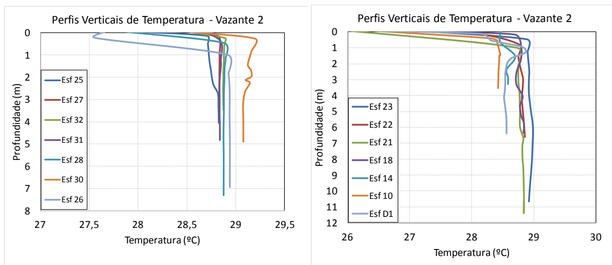
Figura 46 - Perfis verticais de temperatura para as estações amostrais. Campanha 16 - Vazante2 - 21/01/2018.
