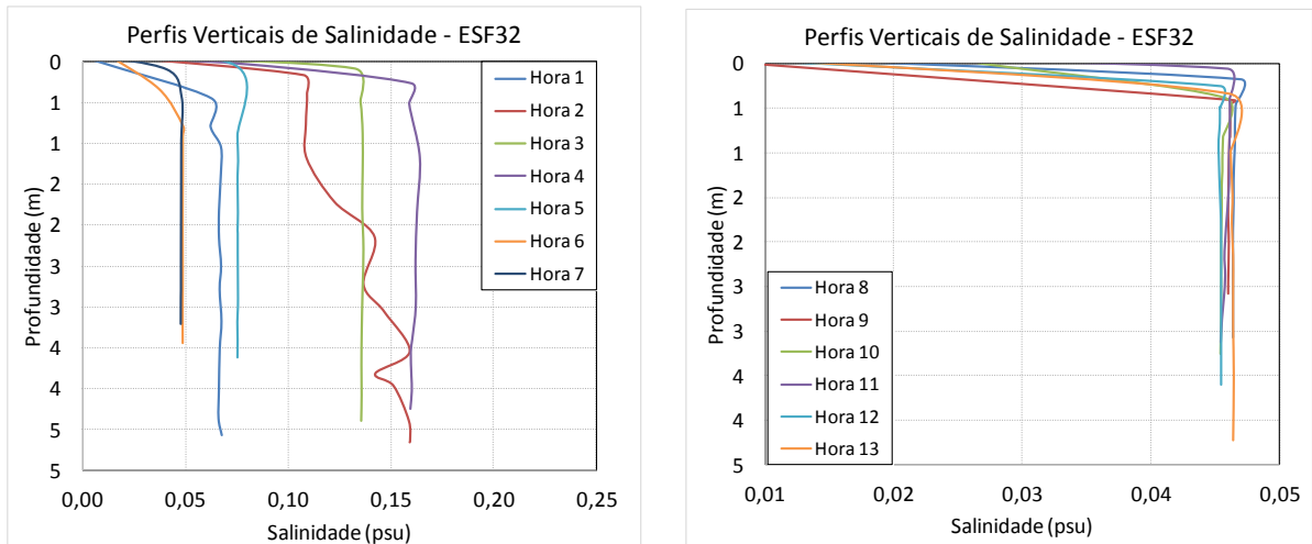
Figura 7 - Perfis verticais de salinidade para a estação amostral fixa ESF 32. Campanha 15 - 06/01/2018. Resolução CONAMA 357/2005 (I - águas doces: águas com salinidade igual ou inferior a 0,5‰).
