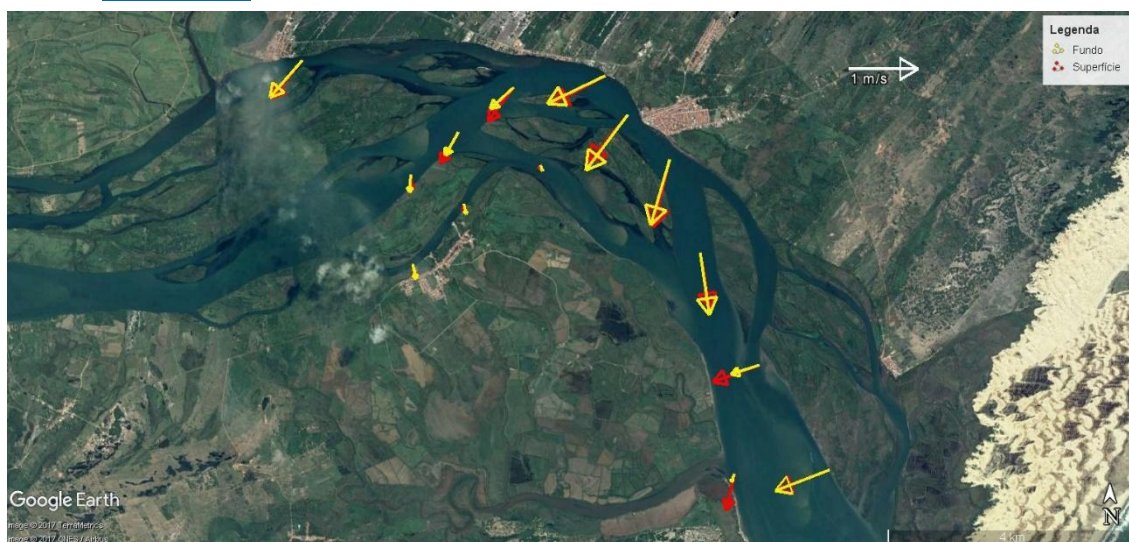
Figura 36 - Média vertical da velocidade e direção da corrente em cada estação amostral. Campanha 16 - Vazante 1 - 20/01/2018.
