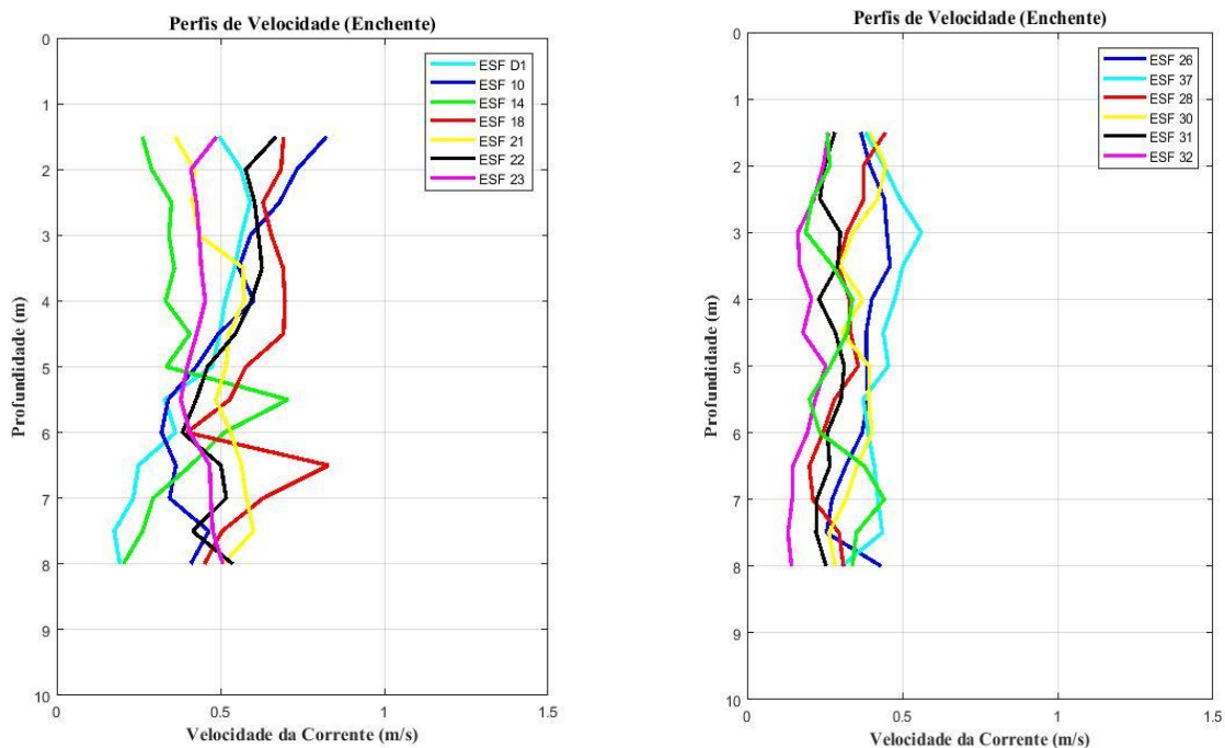
Figura 49 - Perfis verticais de velocidade de corrente para as estações amostrais em período de maré enchente. Campanha 16 - Enchente 2 - 21/01/2018.
