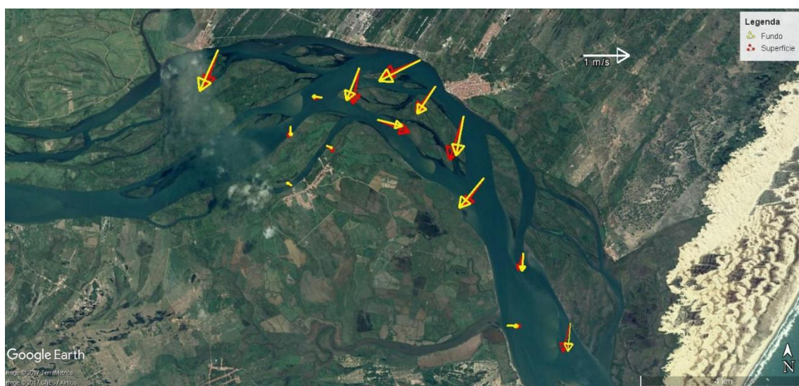
Figura 40 - Média vertical da velocidade e direção da corrente em cada estação amostral. Campanha 16 - Enchente 1 - 20/01/2018.
