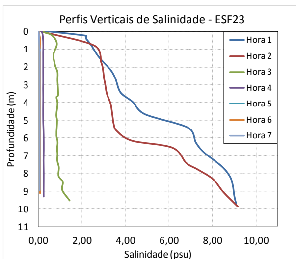
Figura 35 - Perfis verticais de salinidade na estação fixa ESF 23 Campanha 16 - 18/01/2018. Resolução CONAMA 357/2005 (I - águas doces: águas com salinidade igual ou inferior a 0,5‰).
