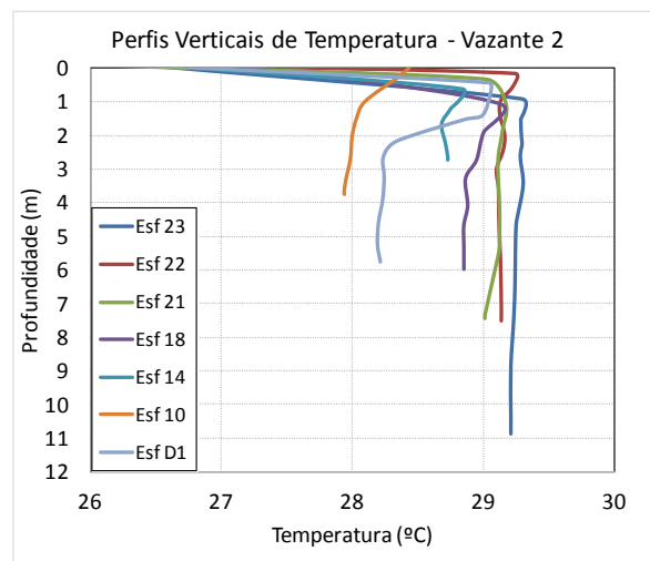
Figura 22 - Perfis verticais de temperatura para as estações amostrais. Campanha 15 - Vazante 2 - 07/01/2018.
