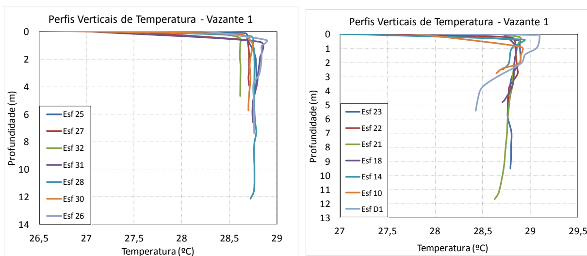
Figura 38 - Perfis verticais de temperatura para as estações amostrais. Campanha 16 – Vazante 1 - 20/01/2018.
