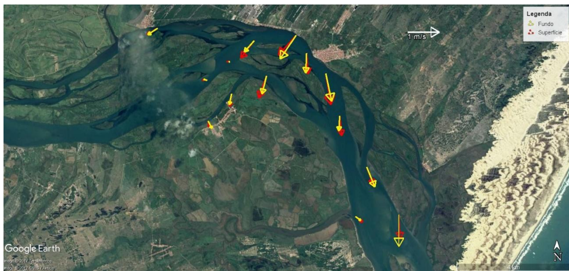
Figura 48 - Média vertical da velocidade e direção da corrente em cada estação amostral. Campanha 16 - Enchente 2 - 21/01/2018.
