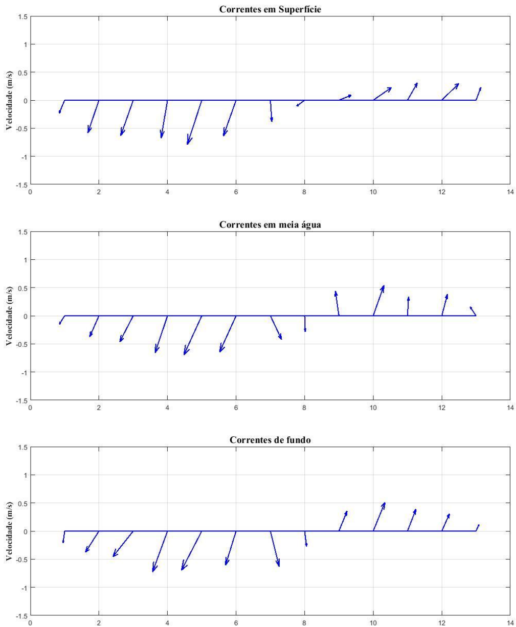
Figura 28 - Diagrama de vetores das correntes em superfície, meia água e fundo para a estação fixa ESF 32. Campanha 16-17/01/2018.
