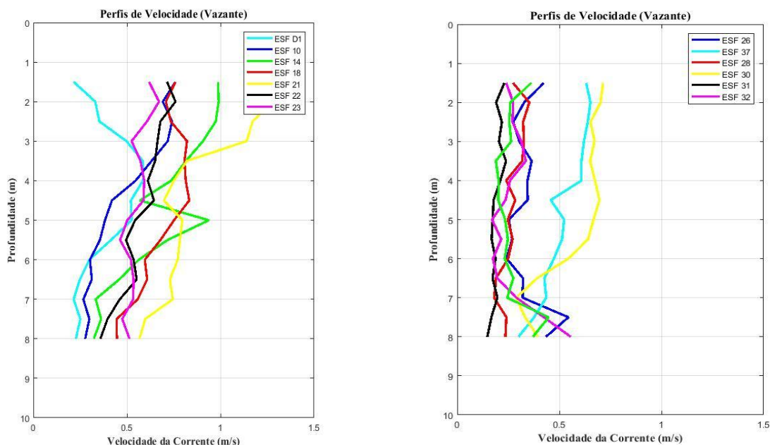
Figura 45 - Perfis verticais de velocidade de corrente para as estações amostrais em período de maré vazante. Campanha 16 - Vazante 2 - 21/01/2018.
