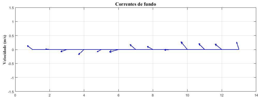
Figura 32 - Diagrama de vetores das correntes em superfície, meia água e fundo para a estação fixa ESF 23. Campanha 16-18/01/2018.
