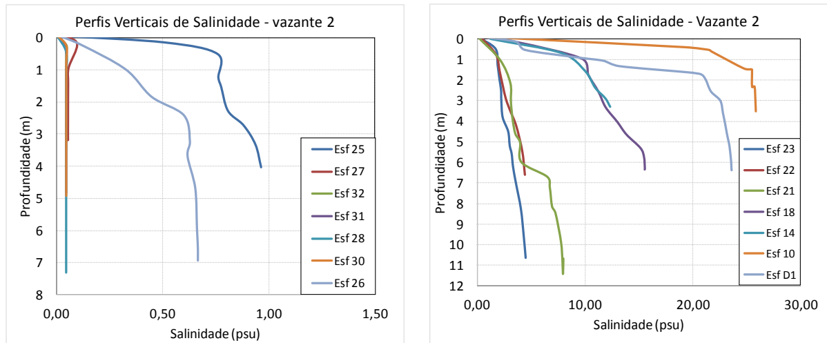
Figura 47 - Perfis verticais de salinidade para as estações amostrais. Campanha 16 - Vazante 2 - 21/01/2018.
