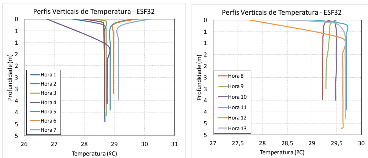
Figura 30- Perfis verticais de temperatura para a estação fixa ESF_32. Campanha 2 - 13 horas - Campanha 16 - 17/01/2018.
