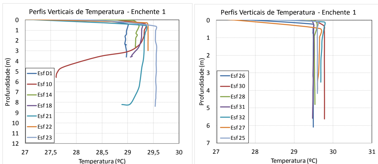
Figura 18 - Perfis verticais de temperatura para as estações amostrais. Campanha 15 - Enchente 1 - 04/01/2018.
