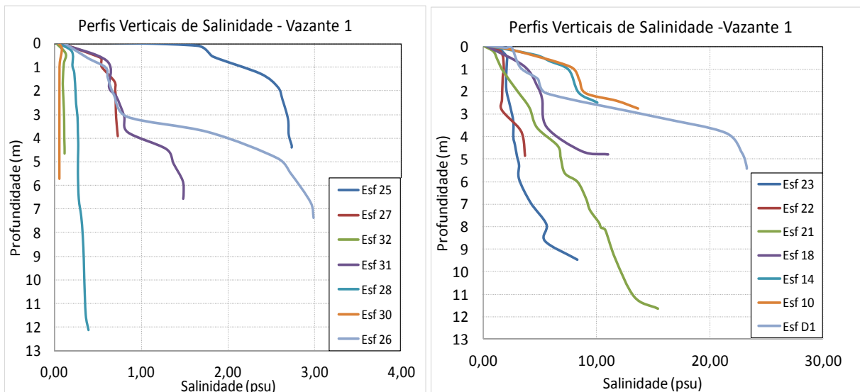
Figura 39 - Perfis verticais de salinidade para as estações amostrais. Campanha 16 - Vazante 1 - 20/01/2018.
