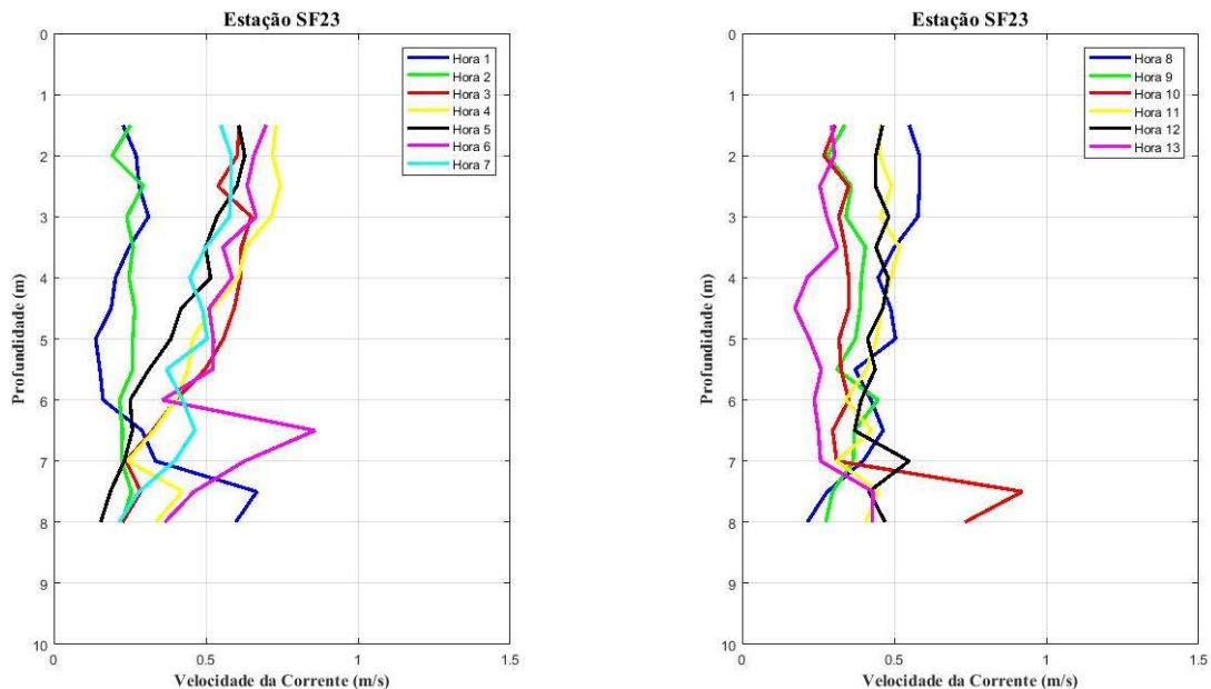
Figura 33 - Perfis verticais de velocidade de corrente na estação fixa ESF 23. Campanha 16 - 18/01/2018.
