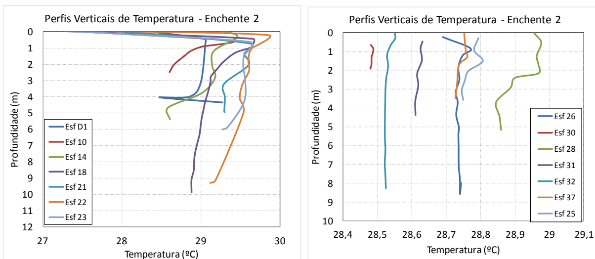
Figura 26 - Perfis verticais de temperatura para as estações amostrais. Campanha 15 - Enchente 2 - 07/01/2018.
