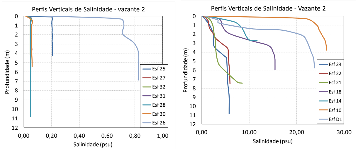
Figura 23 - Perfis verticais de salinidade para as estações amostrais. Campanha 15 - Vazante 2 - 07/01/2018. Resolução CONAMA 357/2005 (I - águas doces: águas com salinidade igual ou inferior a 0,5‰).
