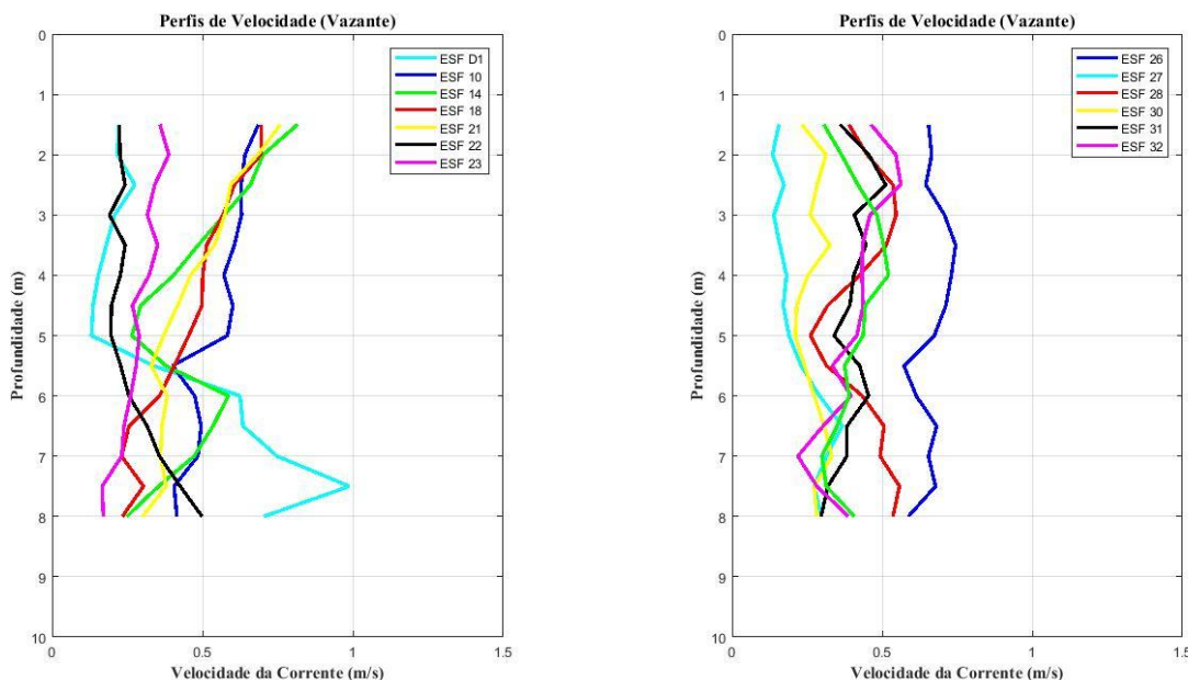
Figura 17 - Perfis verticais de velocidade de corrente para as estações amostrais em período de maré enchente. Campanha 15 - Enchente 1 - 04/01/2018.
