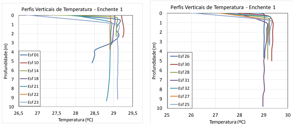
Figura 42 - Perfis verticais de temperatura para as estações amostrais. Campanha 16 - Enchente 1 - 20/01/2018.
