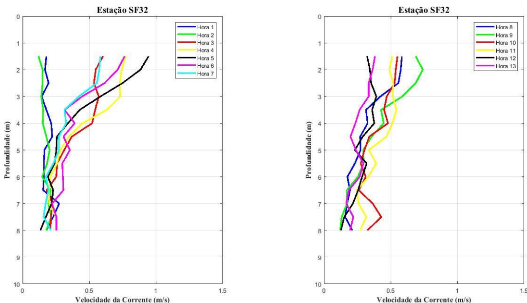
Figura 5 - Perfis verticais de velocidade de corrente na estação fixa ESF 32. Campanha 15 - 06/01/2018.
