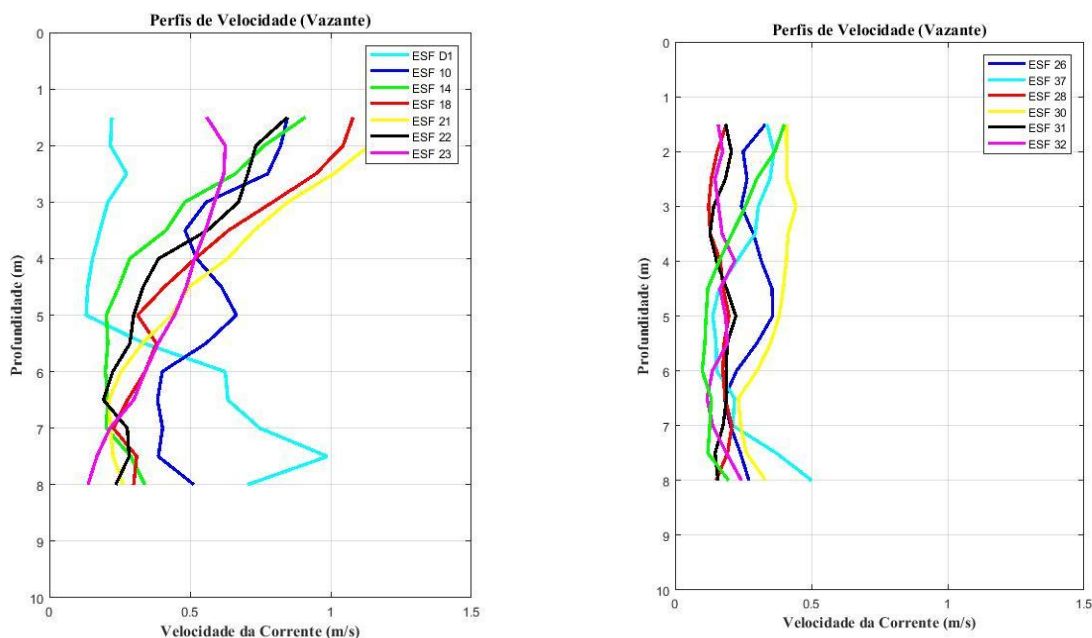
Figura 13 - Perfis verticais de velocidade de corrente para as estações amostrais em período de maré vazante. Campanha 15 - Vazante 1 - 04/01/2018.
