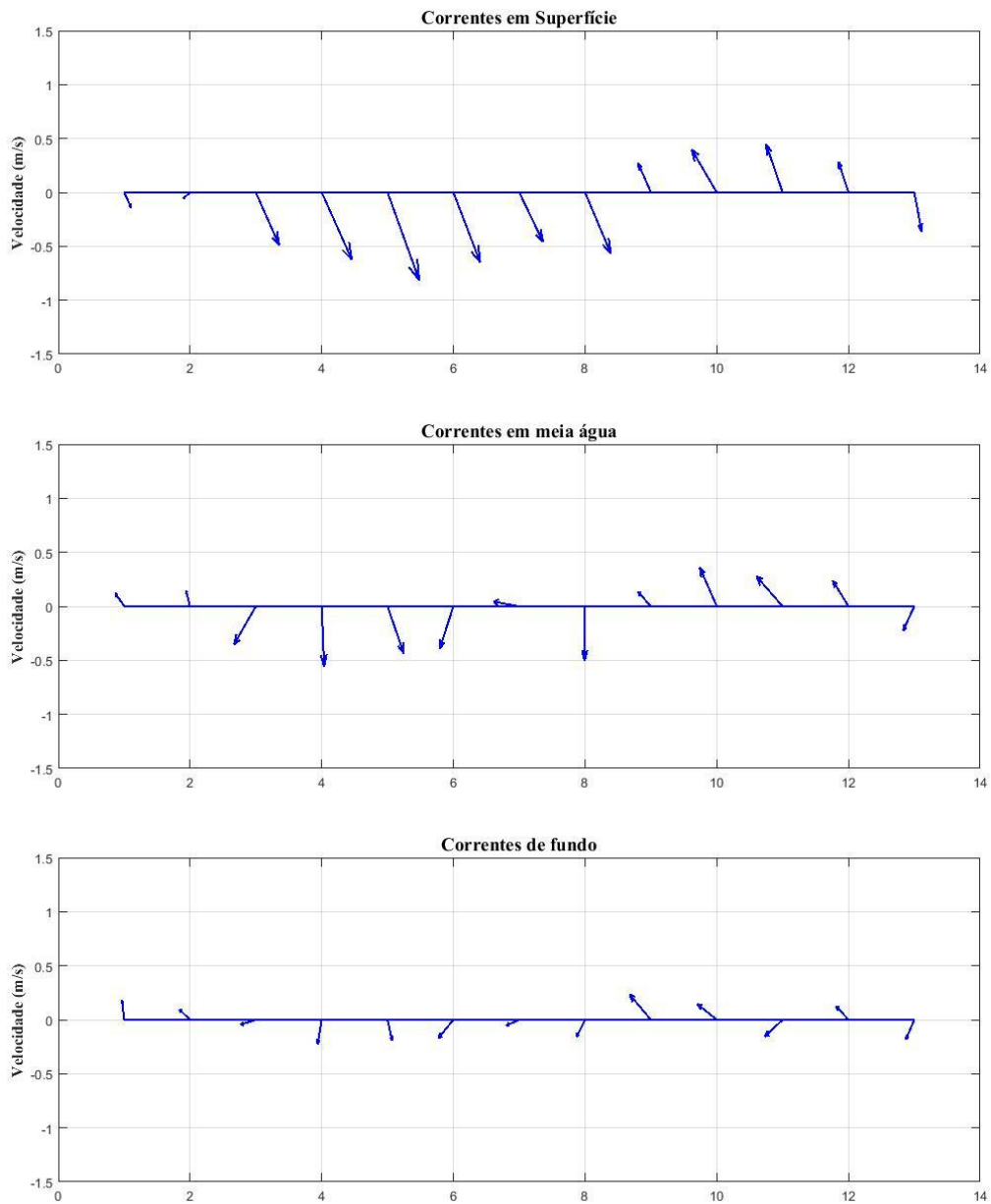
Figura 4 - Diagrama de vetores das correntes em superfície, meia água e fundo para a estação fixa ESF 32. Campanha 15 - 06/01/2018.
