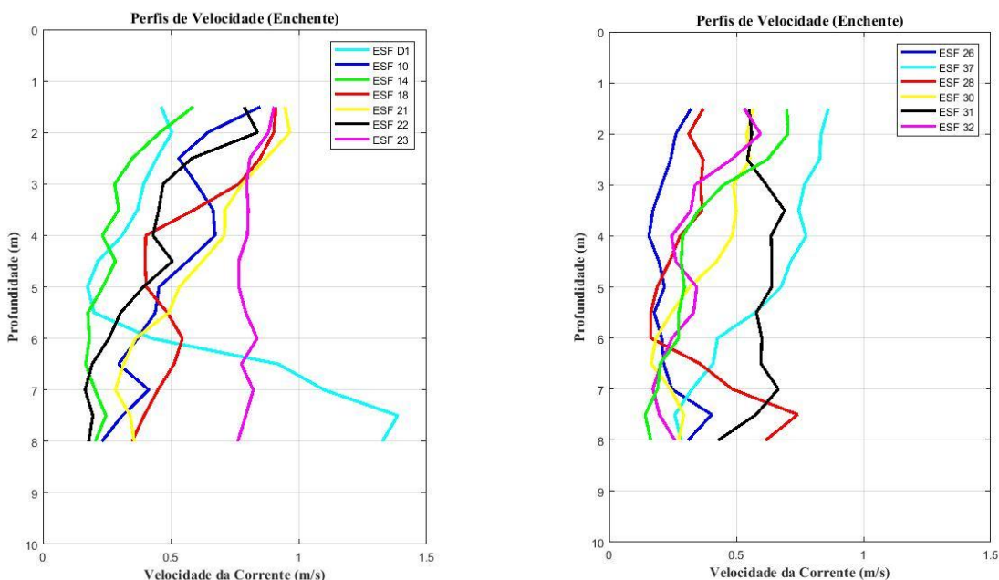
Figura 25 - Perfis verticais de velocidade de corrente para as estações amostrais em período de maré enchente. Campanha 15 - Enchente 2 - 07/01/2018.
