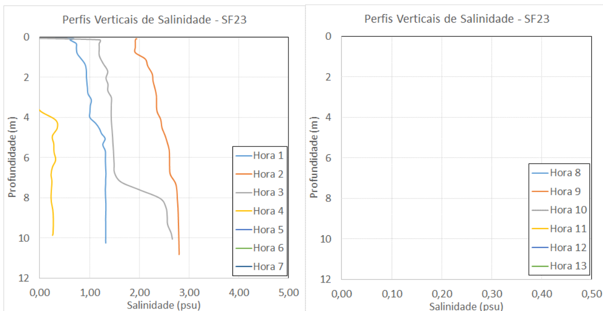
Figura 35 - Perfis verticais de salinidade na estação fixa ESF 23 Campanha 6 - 08/08/2017. Resolução CONAMA 357/2005 (I - águas doces: águas com salinidade igual ou inferior a 0,5 ‰).
