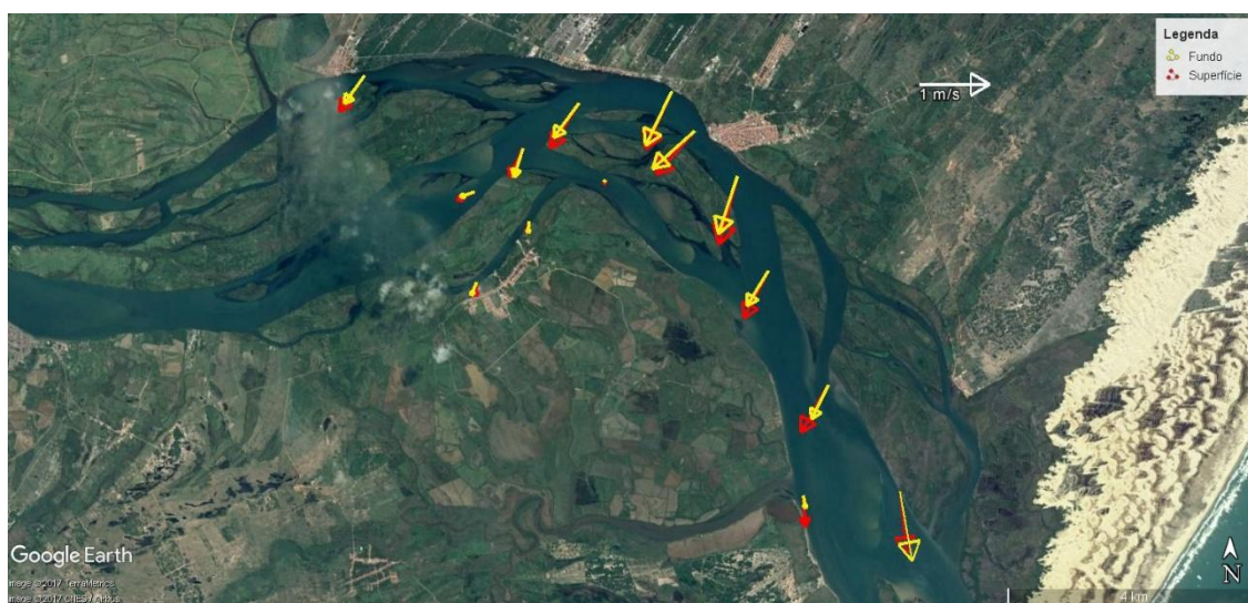
Figura 44 - Média vertical da velocidade e direção da corrente em cada estação amostral. Campanha 6 - Vazante 2 - 11/08/2017.
