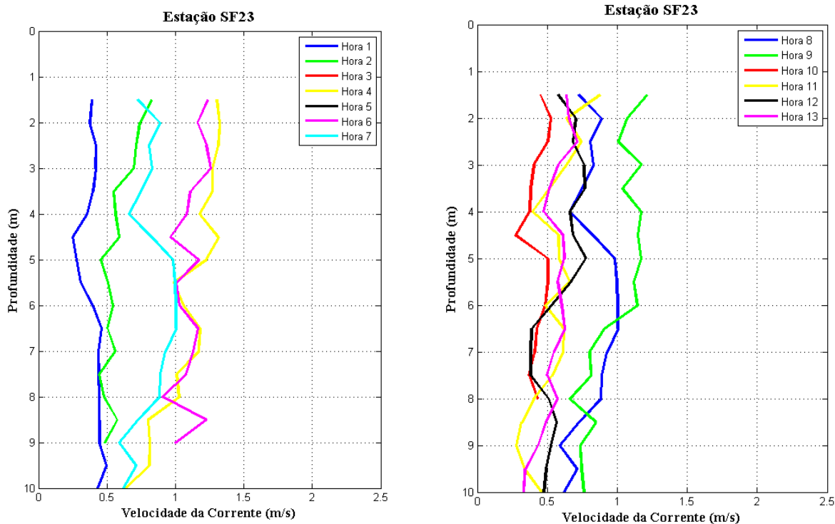
Figura 9 - Perfis verticais de velocidade de corrente na estação fixa ESF 23. Campanha 5 - 22/07/2017.
