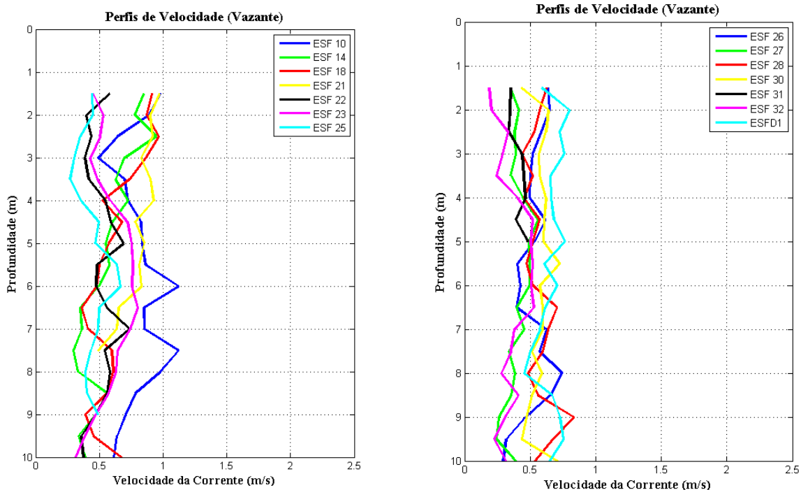
Figura 13 - Perfis verticais de velocidade de corrente para as estações amostrais em período de maré vazante. Campanha 5 - Vazante 1 - 24/07/2017.
