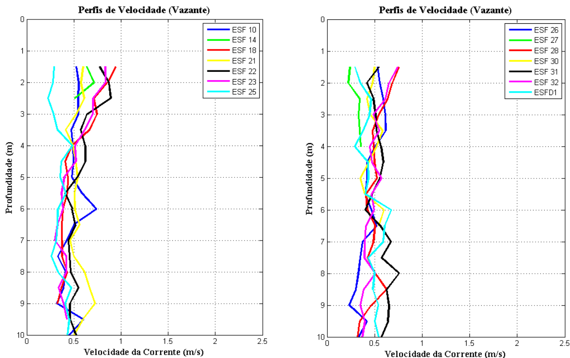
Figura 45 - Perfis verticais de velocidade de corrente para as estações amostrais em período de maré enchente. Campanha 6 - Vazante 2 - 11/08/2017.
