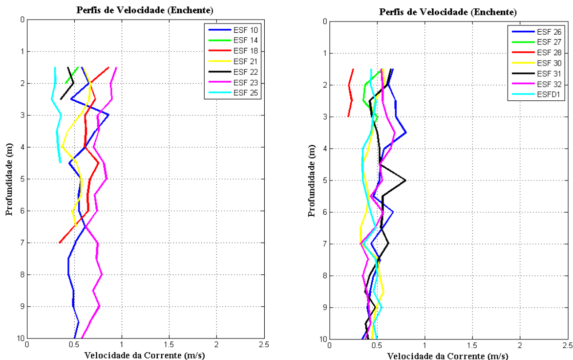
Figura 41 - Perfis verticais de velocidade de corrente para as estações amostrais em período de maré enchente. Campanha 6 - Enchente 1 - 10/08/2017.
