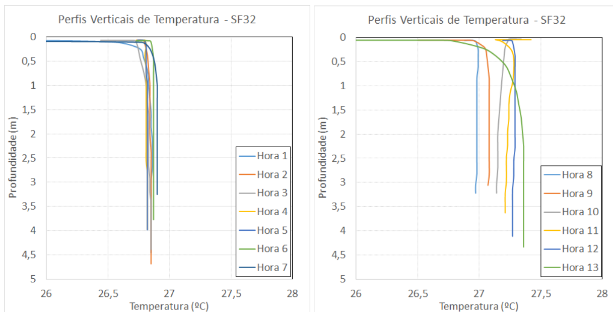
Figura 30 - Perfis verticais de temperatura para a estação fixa ESF_32. Campanha 2 - 12 horas - data: Campanha 6 - 09/08/2017.
