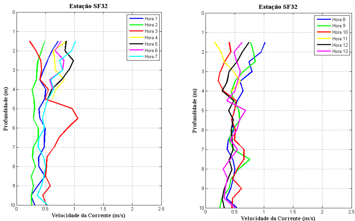
Figura 29 - Perfis verticais de velocidade de corrente na estação fixa ESF 32. Campanha 6 - 09/08/2017.
