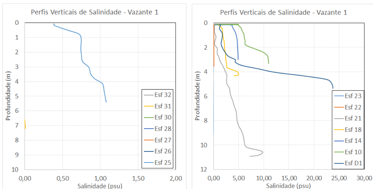
Figura 15 - Perfis verticais de salinidade para as estações amostrais. Campanha 5 - Vazante 1 - 24/07/2017. CONAMA 357/2005 (I - águas doces: águas com salinidade igual ou inferior a 0,5 ‰).
