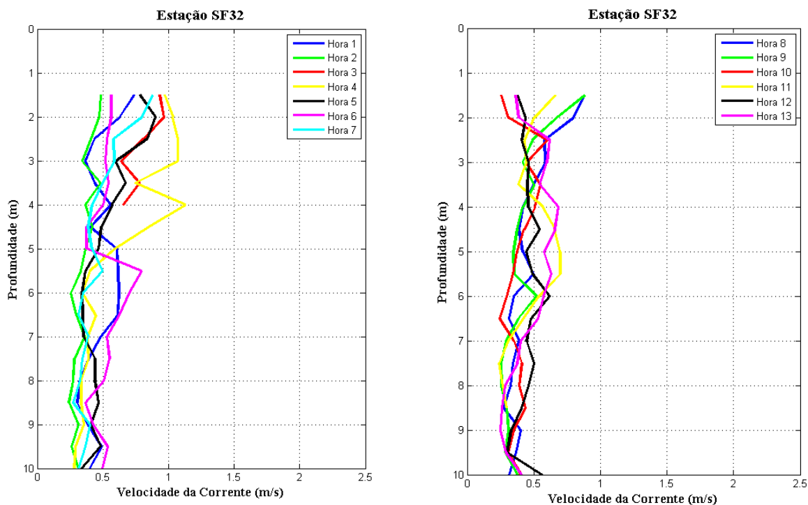
Figura 5 - Perfis verticais de velocidade de corrente na estação fixa ESF 32. Campanha 5 - 23/07/2017.
