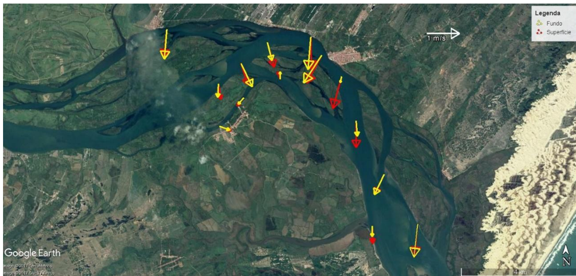
Figura 12 - Média vertical da velocidade e direção da corrente em cada estação amostral. Campanha 5 - Vazante 1 - 24/07/2017.
