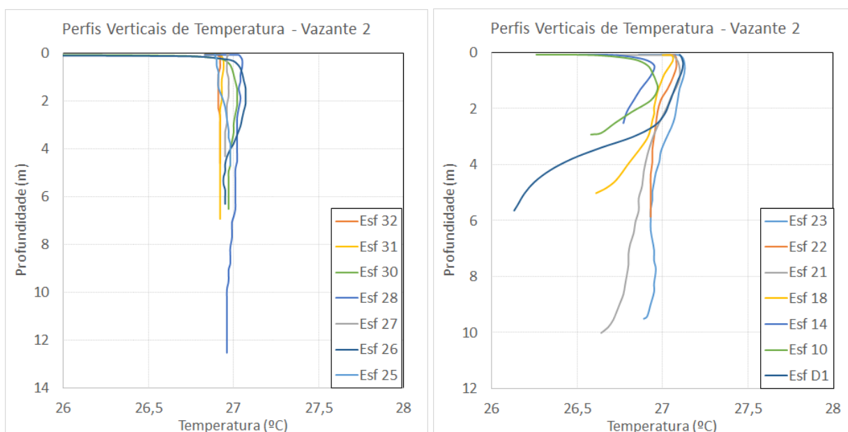
Figura 46 - Perfis verticais de temperatura para as estações amostrais. Campanha 6 - Vazante 2 - 11/08/2017.
