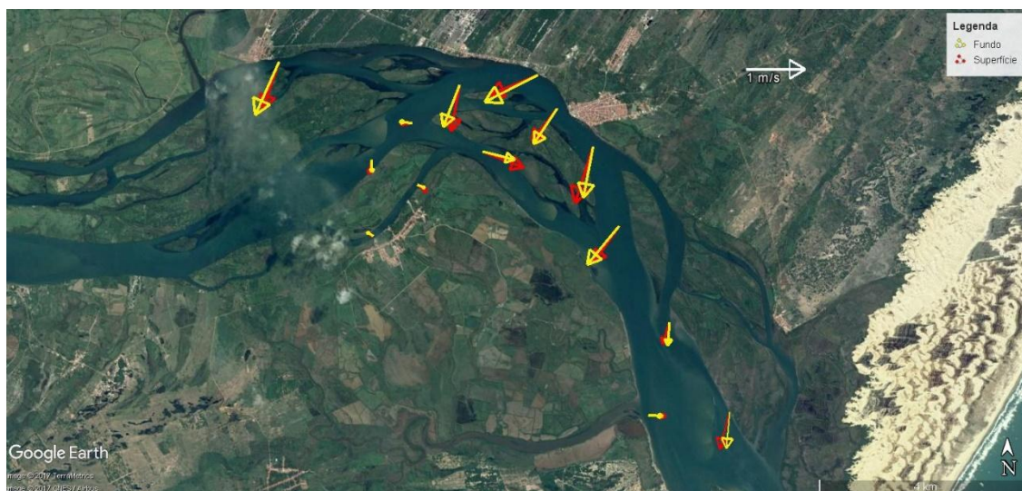
Figura 40 - Média vertical da velocidade e direção da corrente em cada estação amostral. Campanha 6 - Enchente 1 - 10/08/2017.
