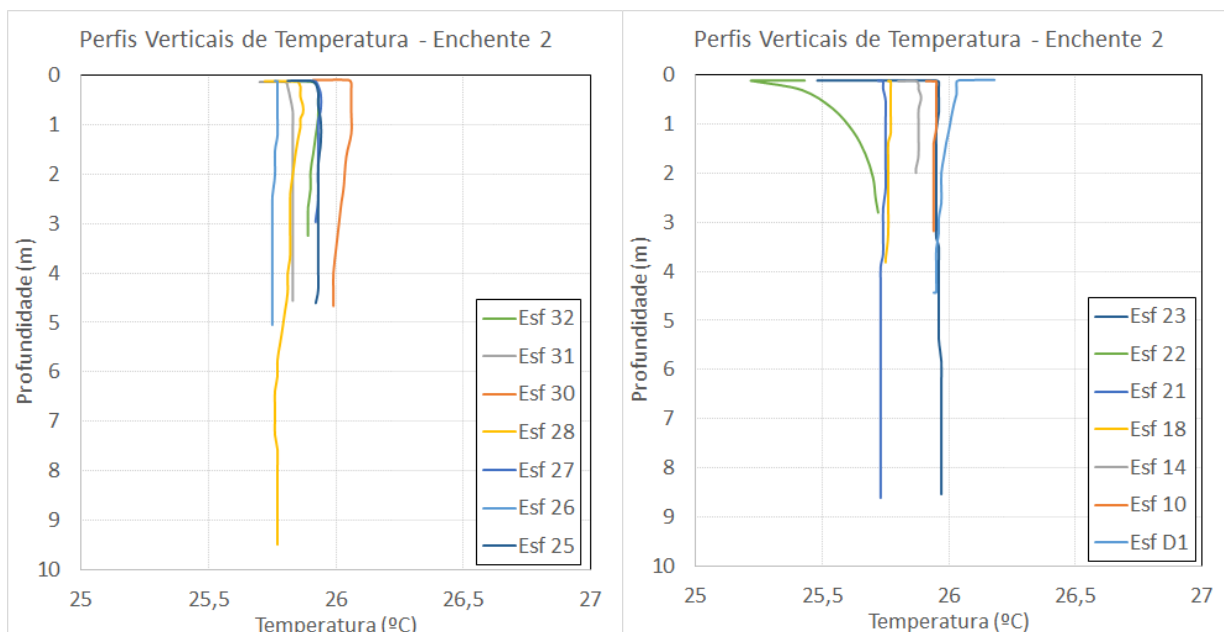
Figura 26 - Perfis verticais de temperatura para as estações amostrais. Campanha 5 - Enchente 2 - 25/07/2017.
