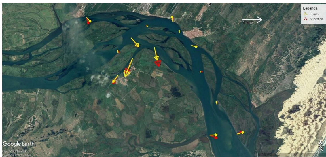
Figura 16 - Média vertical da velocidade e direção da corrente em cada estação amostral. Campanha 5 - Enchente 1 - 24/07/2017.
