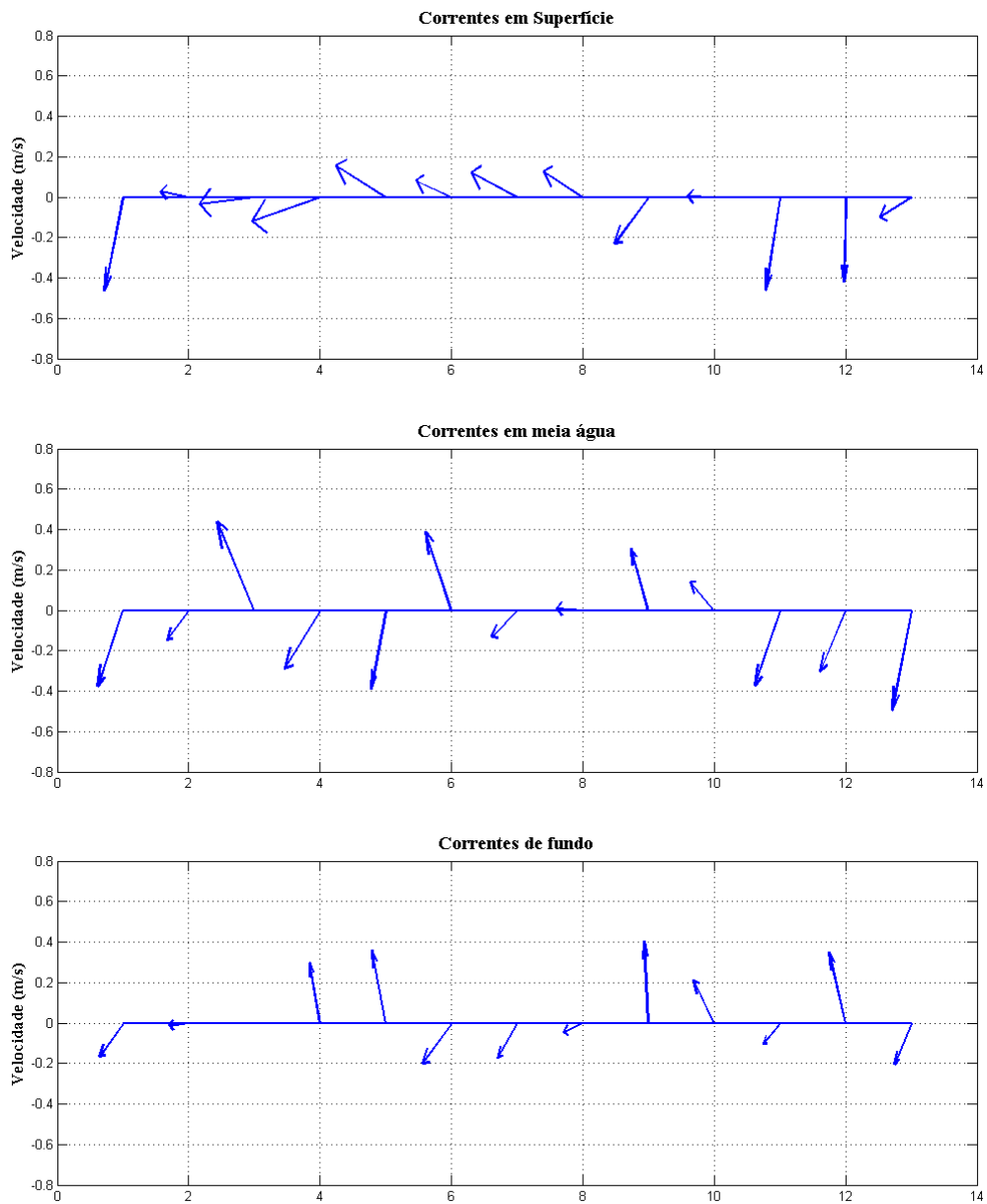
Figura 4 - Diagrama de vetores das correntes em superfície, meia água e fundo para a estação fixa ESF 32. Campanha 5 - 23/07/2017.
