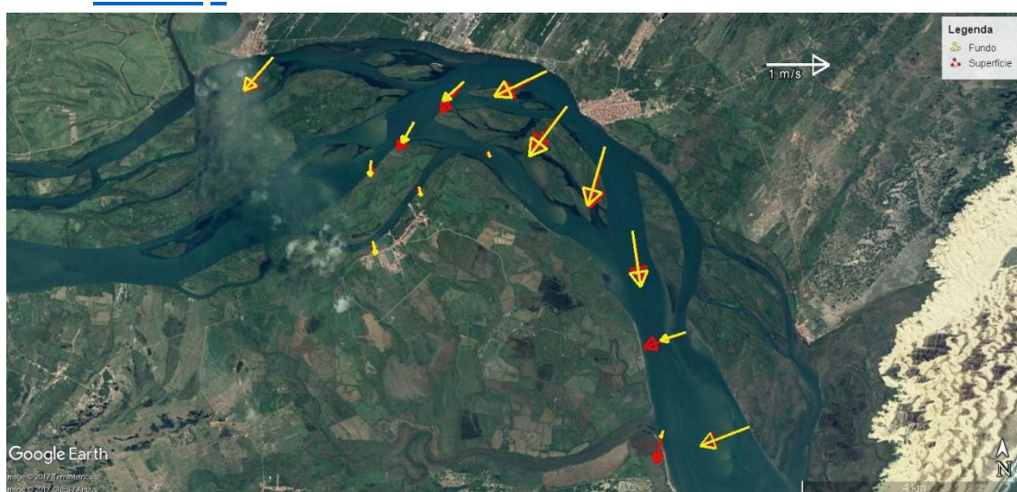
Figura 36 - Média vertical da velocidade e direção da corrente em cada estação amostral. Campanha 6 - Vazante 1 - 10/08/2017.
