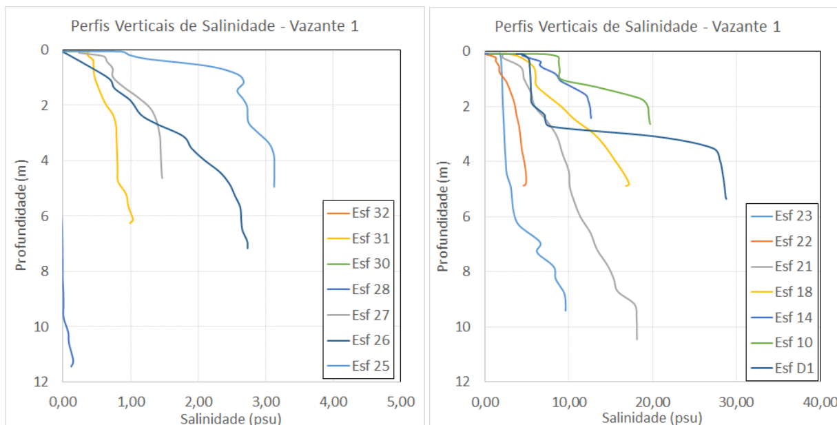
Figura 39 - Perfis verticais de salinidade para as estações amostrais. Campanha 6 - Vazante 1 - 10/08/2017.
