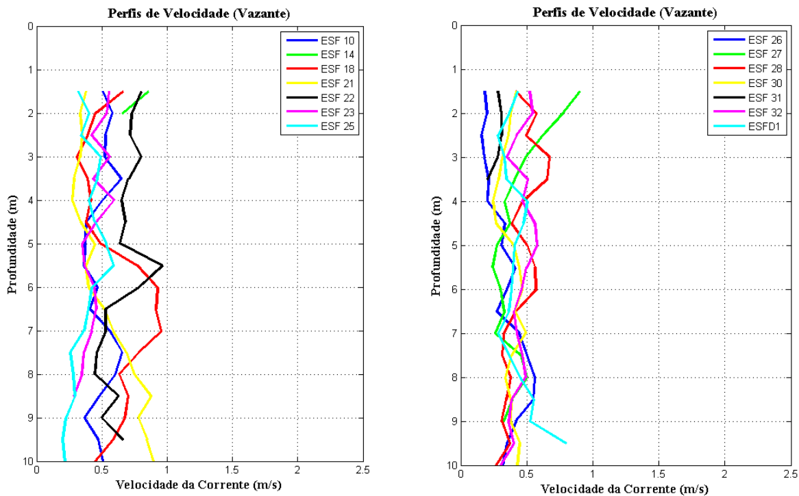
Figura 37 - Perfis verticais de velocidade de corrente para as estações amostrais em período de maré enchente. Campanha 6 - Vazante 1 - 10/08/2017.
