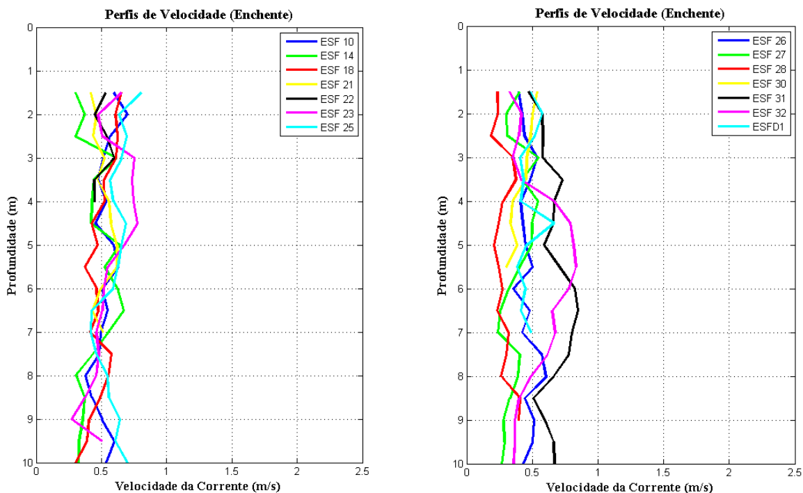
Figura 49 - Perfis verticais de velocidade de corrente para as estações amostrais em período de maré enchente. Campanha 6 - Enchente 2 - 11/08/2017.
