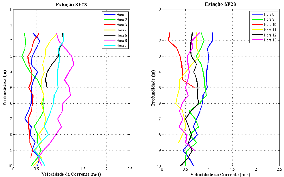
Figura 33 - Perfis verticais de velocidade de corrente na estação fixa ESF 23. Campanha 6 - 08/08/2017.
