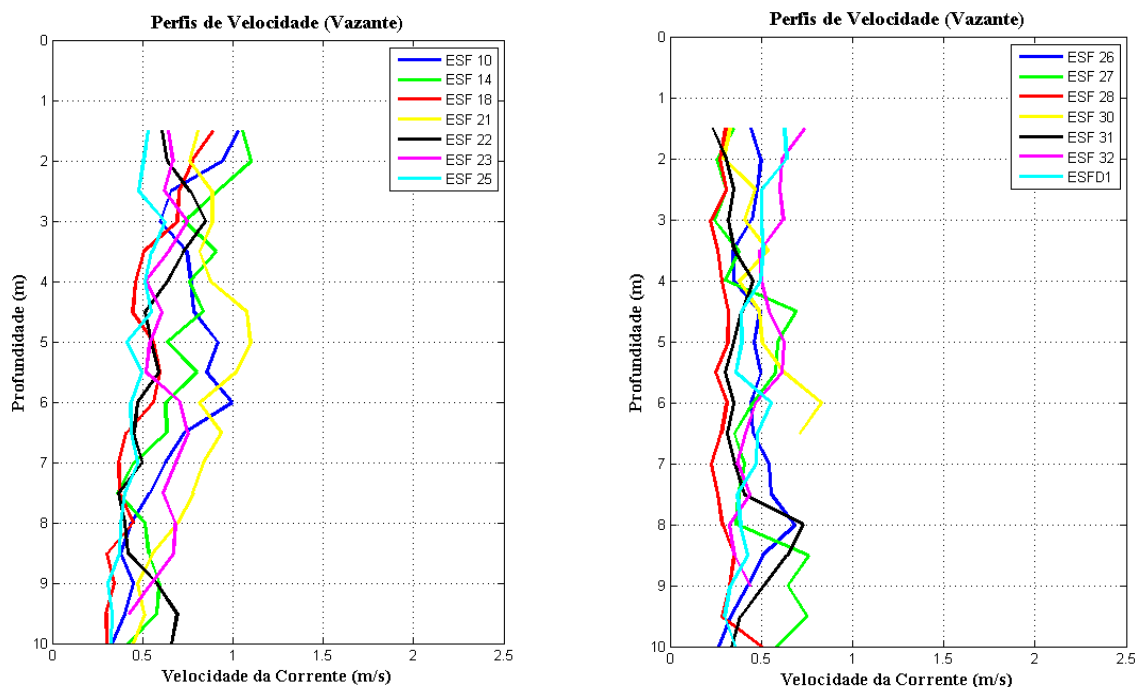
Figura 21 - Perfis verticais de velocidade de corrente para as estações amostrais em período de maré vazante. Campanha 5 - Vazante 2 - 25/07/2017.
