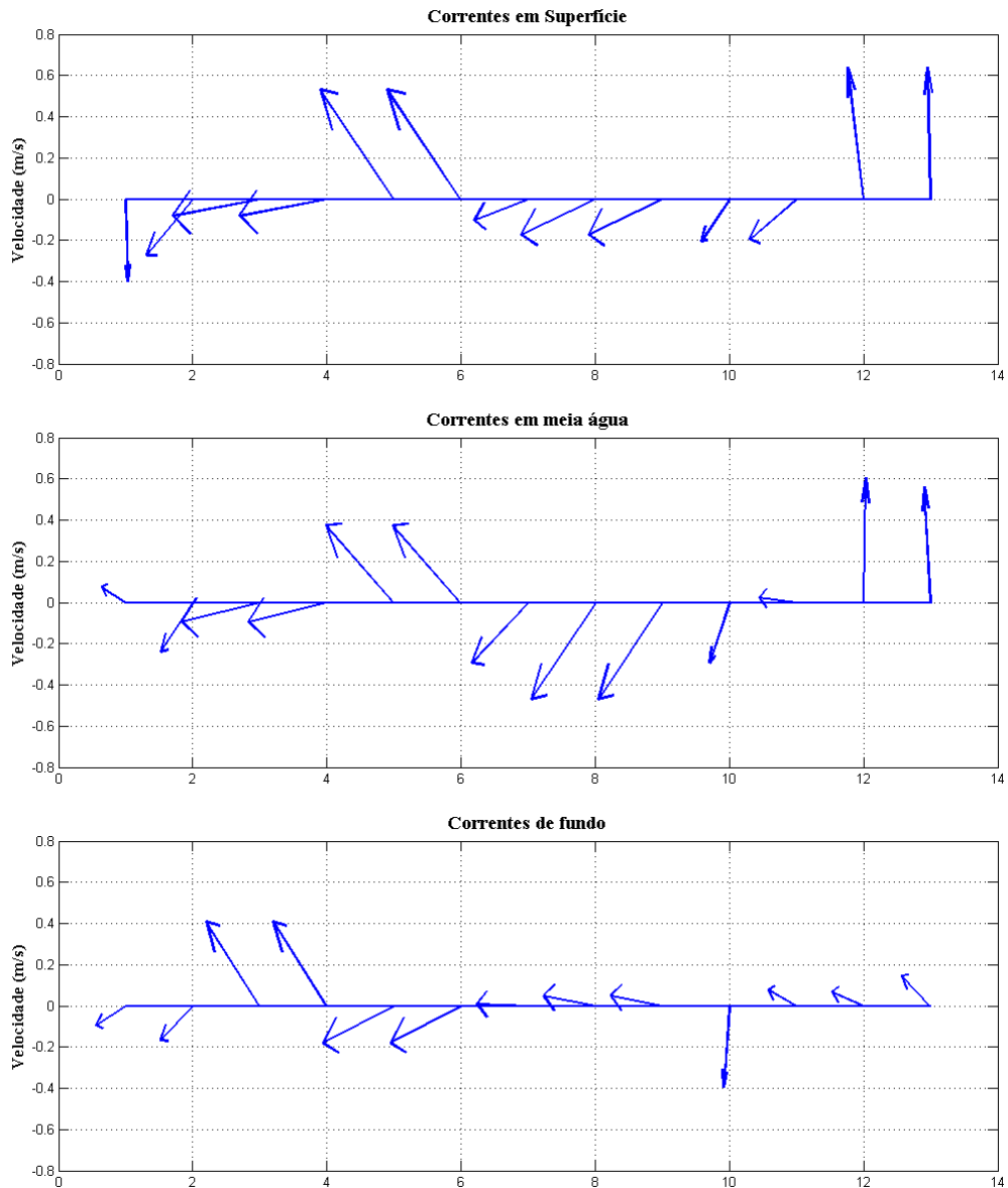
Figura 8 - Diagrama de vetores das correntes em superfície, meia água e fundo para a estação fixa ESF 23. Campanha 5 - 22/07/2017.
