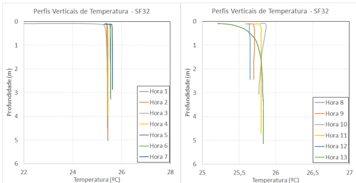
Figura 6 - Perfis verticais de temperatura para a estação amostral fixa ESF 32. Campanha 5 - Vazante 23/07/2017.
