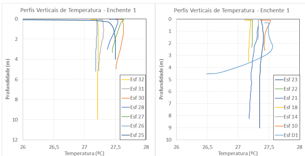
Figura 42 - Perfis verticais de temperatura para as estações amostrais. Campanha 6 - Enchente 1 - 10/08/2017.
