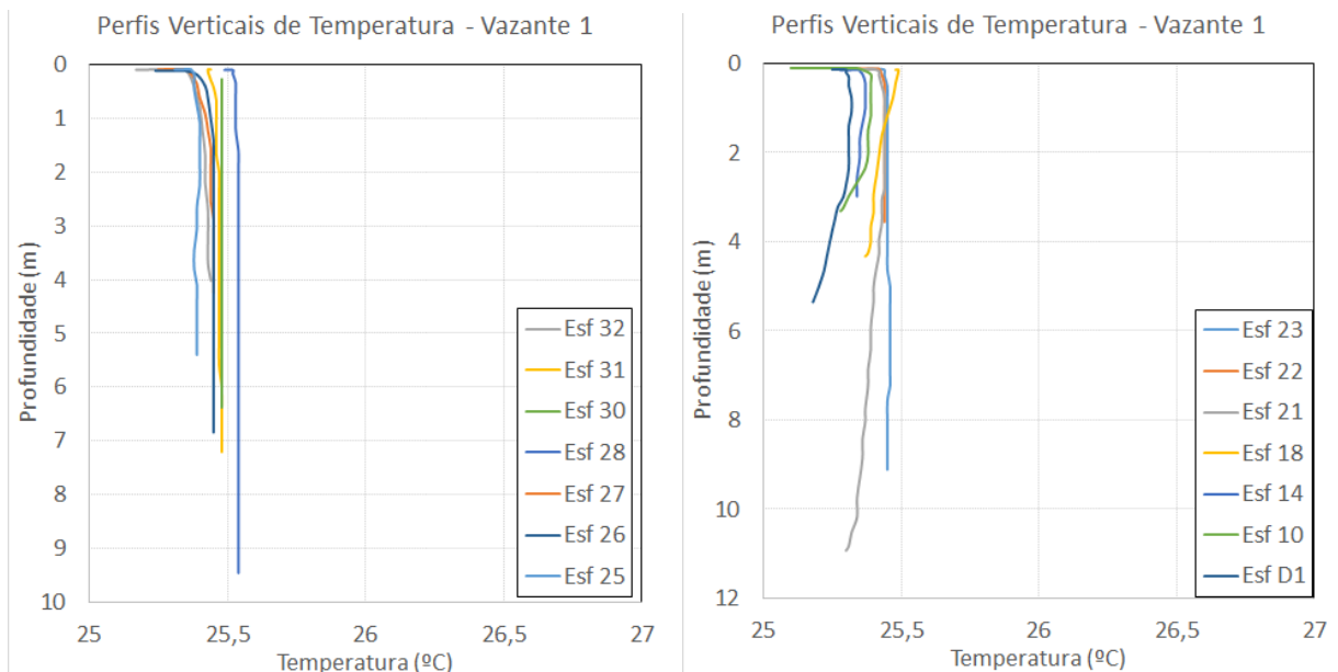
Figura 14 - Perfis verticais de temperatura para as estações amostrais. Campanha 5 - Vazante 1 - 24/07/2017.
