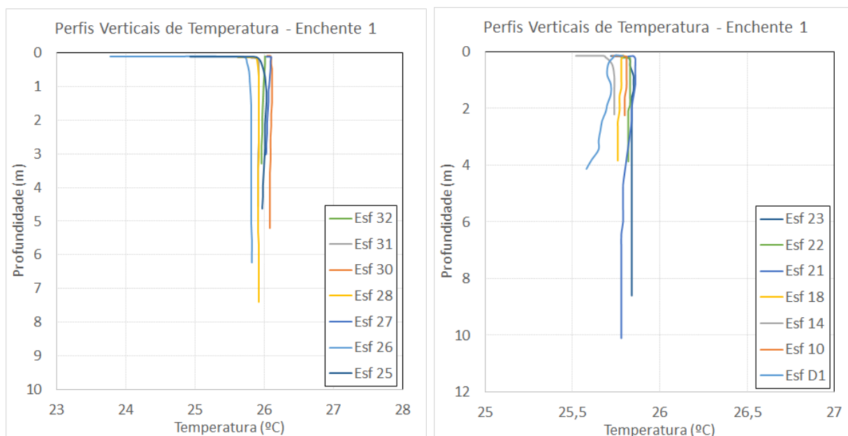
Figura 18 - Perfis verticais de temperatura para as estações amostrais. Campanha 5 - Enchente 1 - 24/07/2017.
