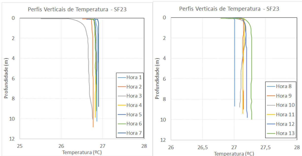
Figura 34 - Perfis verticais de temperatura para a estação fixa na estação fixa ESF 23. Campanha 6 - 08/08/2017.
