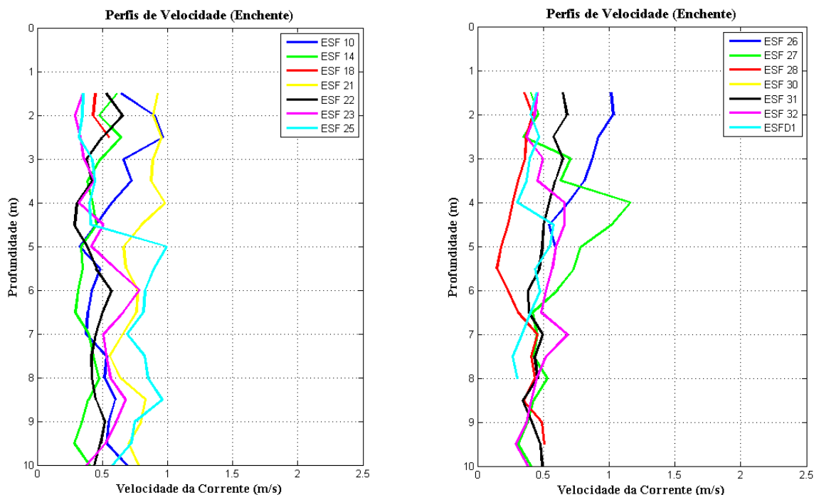
Figura 25 - Perfis verticais de velocidade de corrente para as estações amostrais em período de maré enchente. Campanha 5 - Enchente 2 - 25/07/2017.
