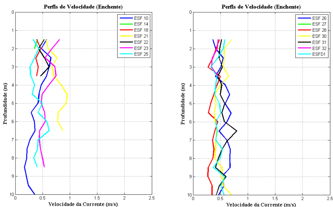
Figura 17 - Perfis verticais de velocidade de corrente para as estações amostrais em período de maré enchente. Campanha 5 - Enchente 1 - 24/07/2017.
