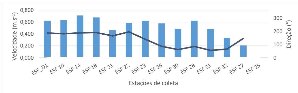
Figura 5: Variação média da velocidade (barras azuis) e da direção (linha azul escuro) das correntes na coluna entre pelas estações de amostragem da cunha salina da foz do Rio São Francisco, durante a Baixamar da maré de sizígia (lua nova) do dia 13/04/2021.
