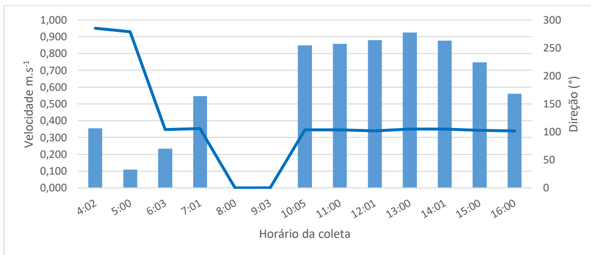
Figura 26: Dados hidrodinâmicos coletados durante a campanha fixa na bomba de captação de água da cidade de Brejo Grande, SE (ESF 32), no dia 15 de Abril de 2021. As barras azuis representam a velocidade da corrente e a linha laranja a direção.
