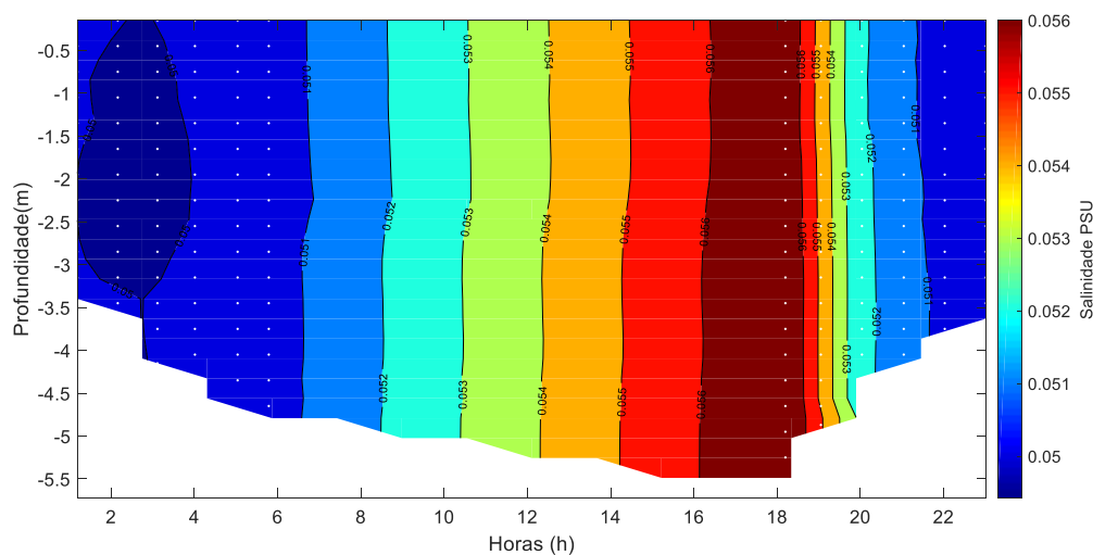
Figura 30: Distribuição temporal da salinidade da água durante o monitoramento fixo da cunha salina, realizado no dia 27-28 de Abril de 2021, nas proximidades da bomba de captação de água de Penedinho (ESF 30). Os pontos brancos representam o momento do dia da campanha quando os perfis foram realizados e o formato do fundo corresponde à variação do nível da coluna d'água ou o ponto máximo de alcance do CTD.
