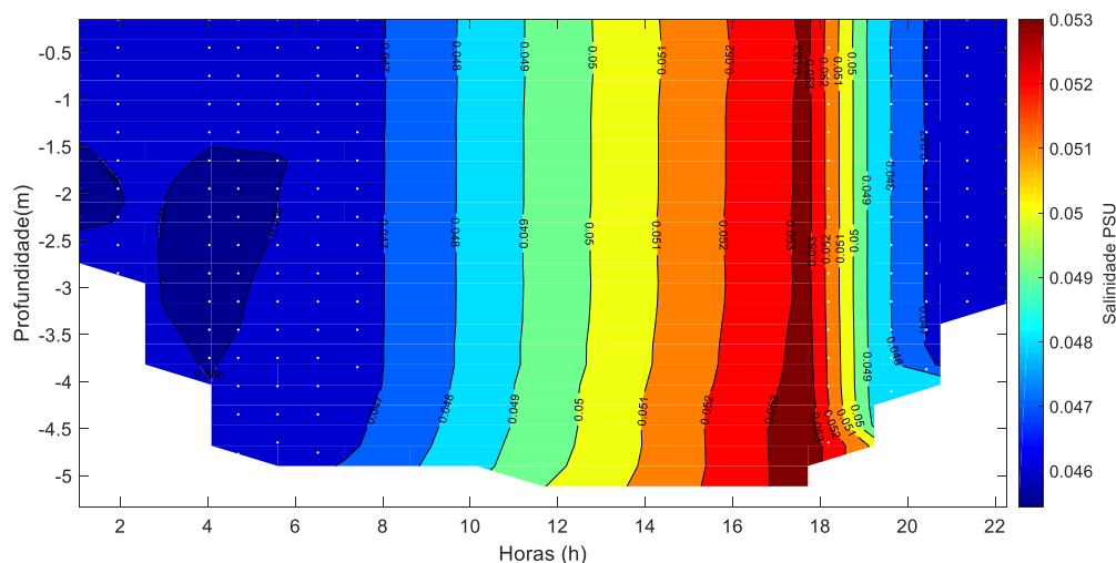
Figura 27: Distribuição temporal da salinidade da água durante o monitoramento fixo da cunha salina, realizado no dia 13-14 de Abril de 2021, nas proximidades da bomba de captação de água da cidade de Brejo Grande- SE. Os pontos brancos representam o momento do dia da campanha quando os perfis foram realizados e o formato do fundo corresponde à variação do nível da coluna d'água ou o ponto máximo de alcance do CTD.
