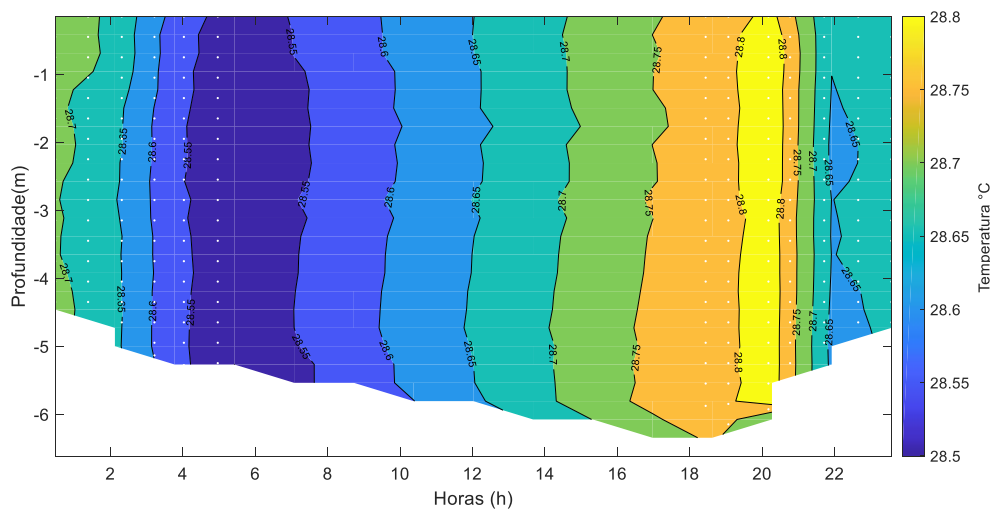
Figura 32: Distribuição temporal da temperatura para o monitoramento fixo de 12 horas da cunha salina, realizado no dia 14-15 de Abril de 2021 nas proximidades da bomba de captação de água da cidade de Brejo Grande (ESF 32). Os pontos brancos representam o momento do dia da campanha quando os perfis foram realizados e o formato do fundo corresponde à variação do nível da coluna d'água ou o ponto máximo de alcance do CTD.
