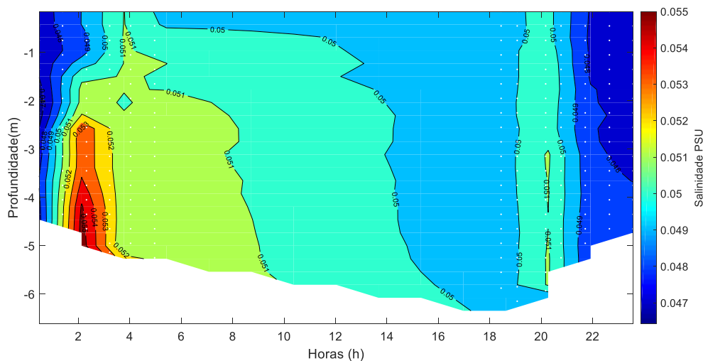
Figura 28: Distribuição temporal da salinidade da água durante o monitoramento fixo da cunha salina, realizado no dia 14-15 de Abril de 2021, nas proximidades da bomba de captação de água da cidade de Penedinho (ESF 30), ESF 32. Os pontos brancos representam o momento do dia da campanha quando os perfis foram realizados e o formato do fundo corresponde à variação do nível da coluna d'água ou o ponto máximo de alcance do CTD.
