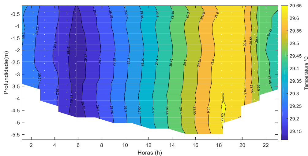
Figura 34: Distribuição temporal da temperatura para o monitoramento fixo de 12 horas da cunha salina, realizado no dia 28-29 de Abril de 2021 nas proximidades da bomba de captação de água da cidade Brejo Grande-SE (ESF 32). Os pontos brancos representam o momento do dia da campanha quando os perfis foram realizados e o formato do fundo corresponde à variação do nível da coluna d'água ou o ponto máximo de alcance do CTD.
