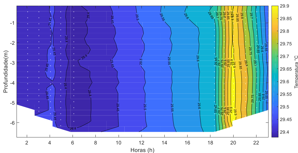
Figura 33: Distribuição temporal da temperatura para o monitoramento fixo de 12 horas da cunha salina, realizado no dia 27-28 de Abril de 2021 nas proximidades da bomba de captação de água da cidade de Piaçabuçu (Penedinho, ESF 30). Os pontos brancos representam o momento do dia da campanha quando os perfis foram realizados e o formato do fundo corresponde à variação do nível da coluna d'água ou o ponto máximo de alcance do CTD.
