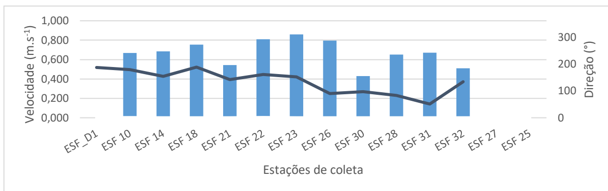
Figura 7: Variação média da velocidade (barras azuis) e da direção (linha azul escura) das correntes na coluna entre pelas estações de amostragem da cunha salina da foz do Rio São Francisco, durante a baixamar da maré de sizígia (lua nova) do dia 14/04/2021.
