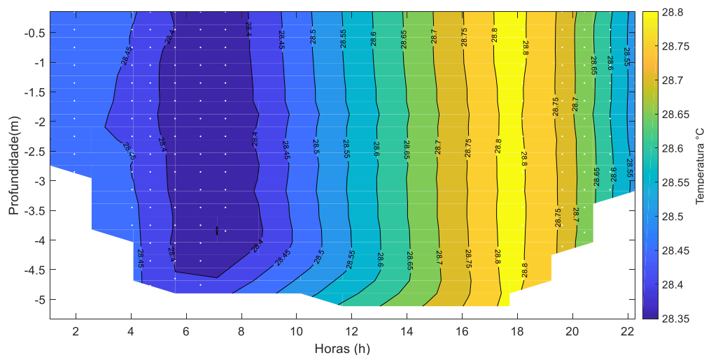
Figura 31: Distribuição temporal da temperatura da água durante o monitoramento fixo realizado no dia 13-14 de Abril de 2021, nas proximidades da bomba de captação de água da cidade de Brejo Grande (ESF 32). Os pontos brancos representam o momento do dia da campanha quando os perfis foram realizados e o formato do fundo corresponde à variação do nível da coluna d'água ou o ponto máximo de alcance do CTD.
