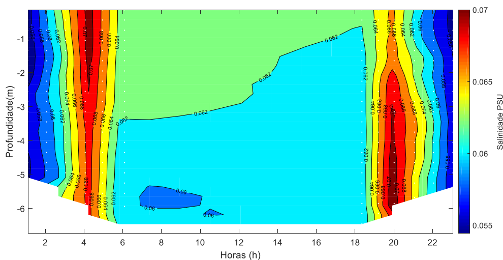
Figura 29: Distribuição temporal da salinidade da água durante o monitoramento fixo da cunha salina, realizado no dia 28-29 de Abril de 2021, nas proximidades da bomba de captação de água da cidade de Brejo Grande, ESF 32. Os pontos brancos representam o momento do dia da campanha quando os perfis foram realizados e o formato do fundo corresponde à variação do nível da coluna d'água ou o ponto máximo de alcance do CTD.
